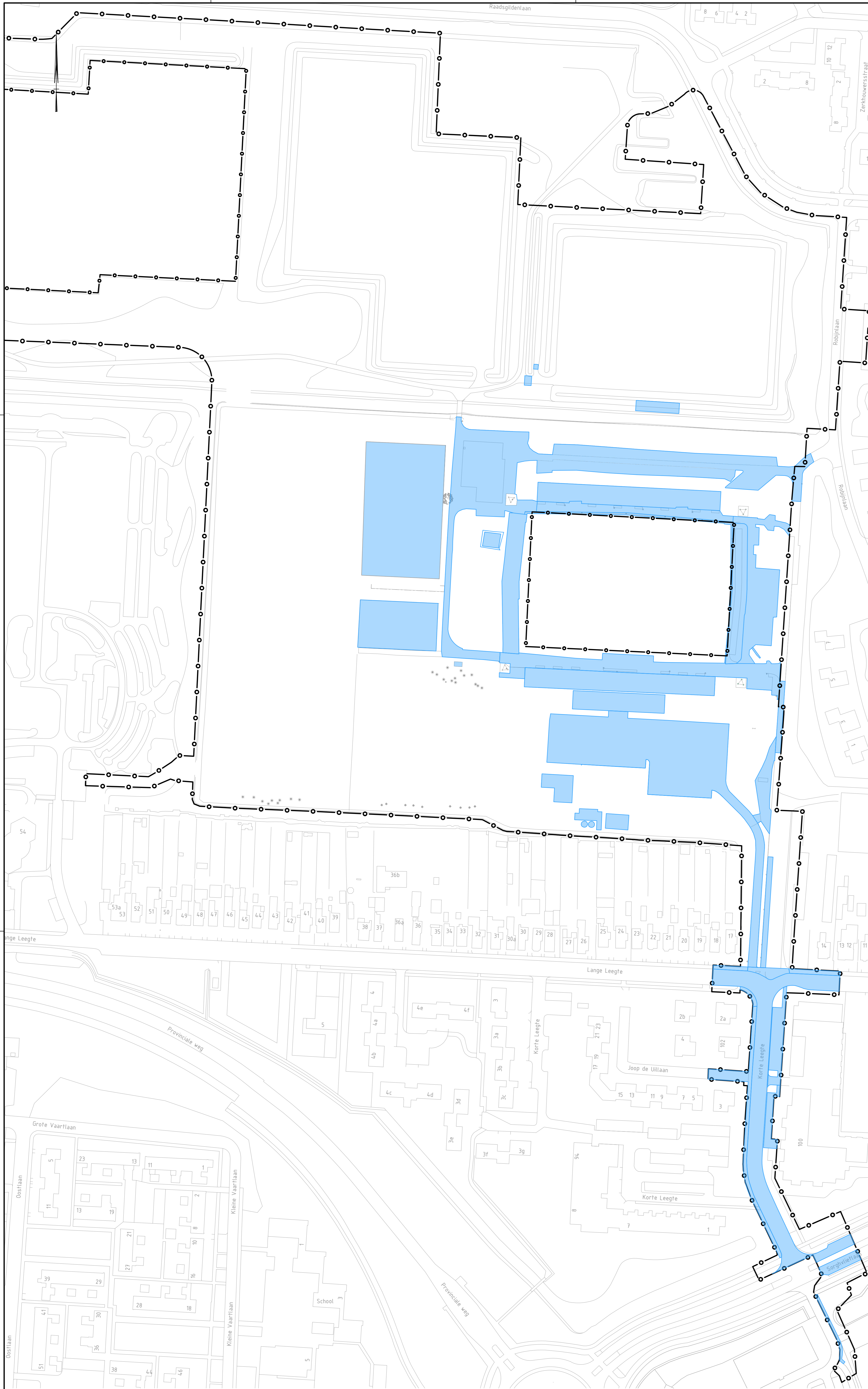
Bestaande situatie ingezameld afvoerend verhard oppervlak Opp: ca. 26369 m 2 schaal 1:1000
