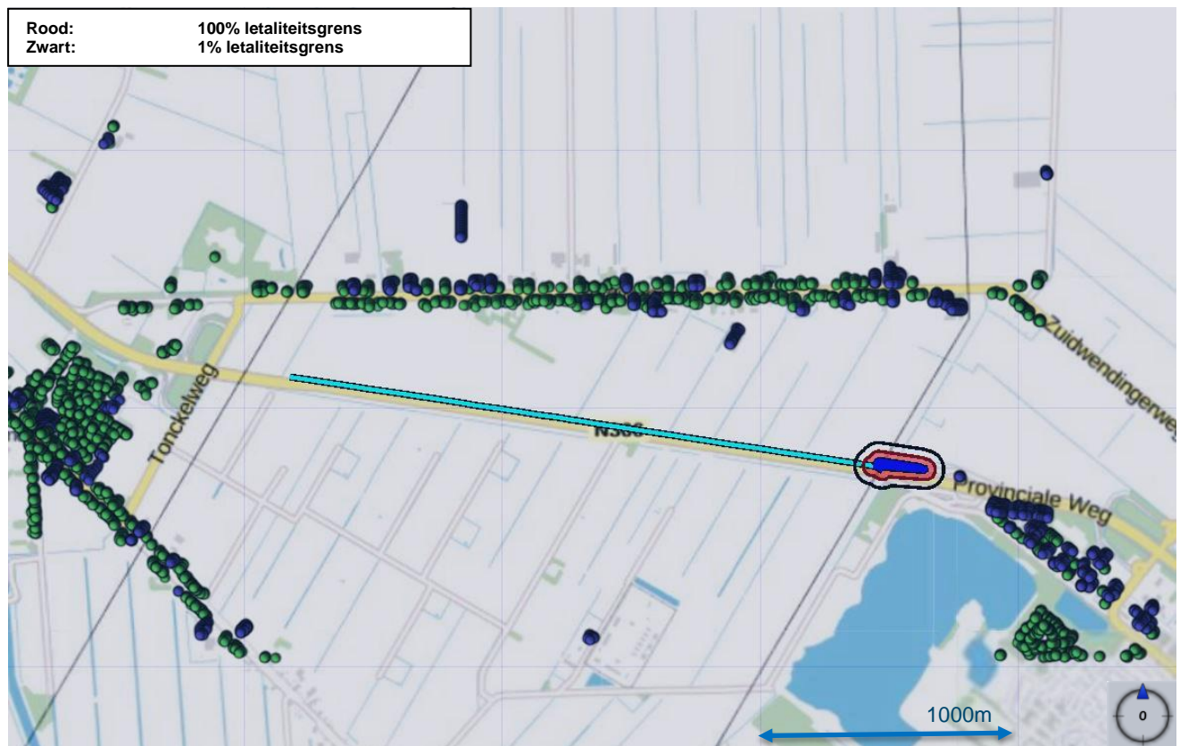
Figuur 2 Invloedsgebied van de leiding N-524-21 (donkerblauw) in de toekomstige situatie.
