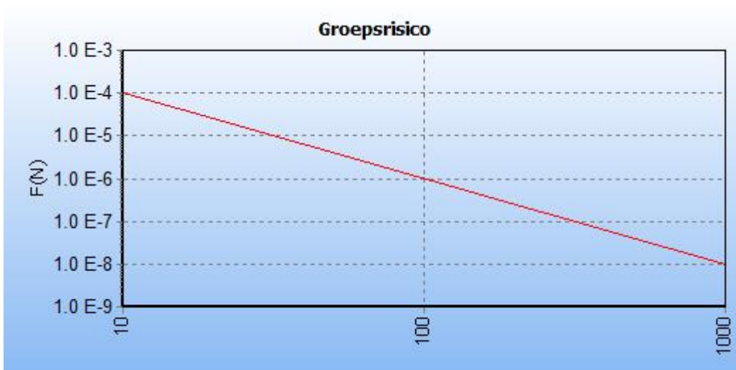
Figuur 6 FN-curve van gastransportleiding N-524-21 in de huidige situatie.
