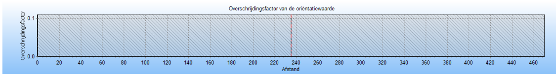
Figuur 7 Overschrijding van het groepsrisico als functie van de stationing van N-524-21 in de toekomstige situatie.
