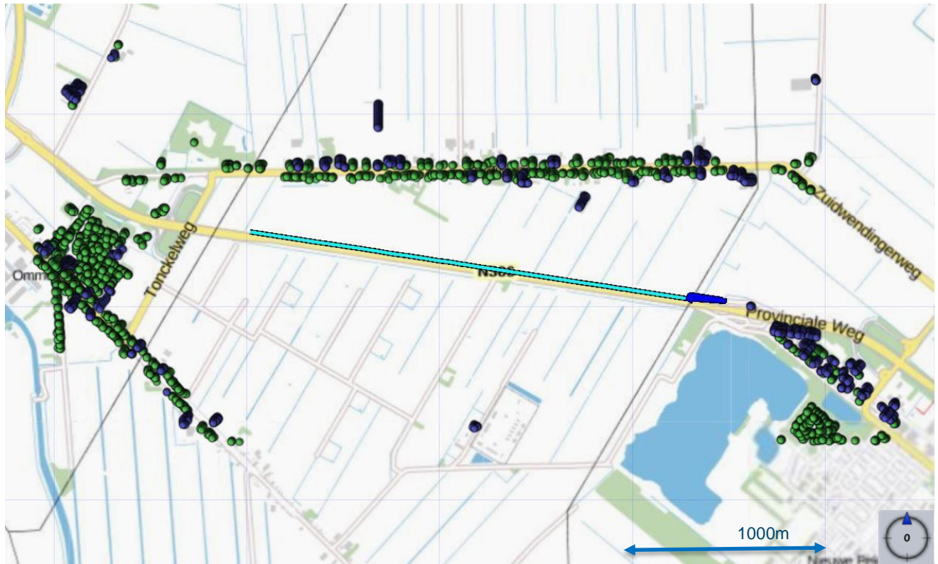
Figuur 1 Ligging van gastransportleidingen N-524-21 (donkerblauw) in de toekomstige situatie.
