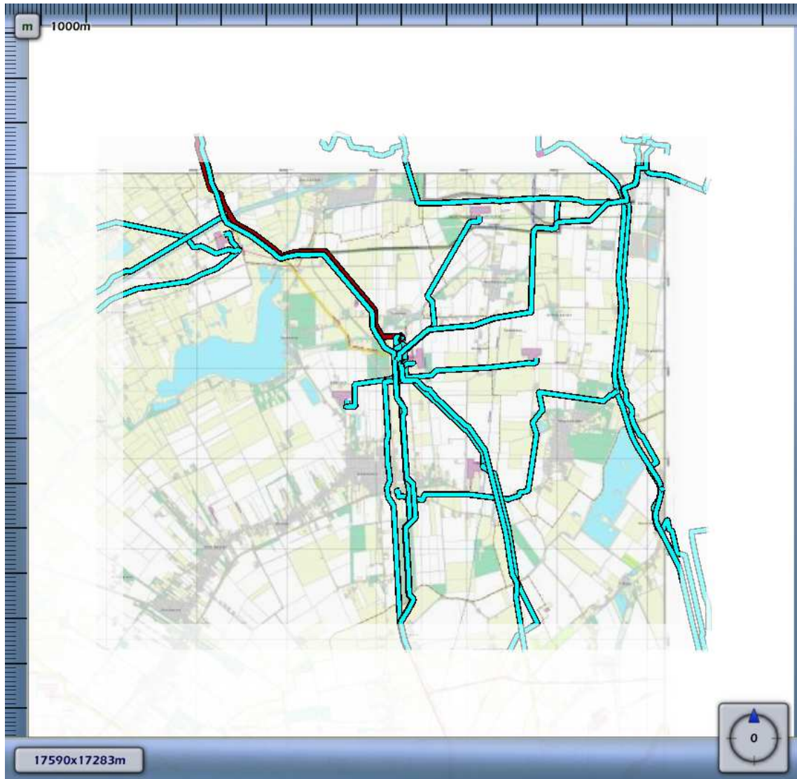
3.14 Figuur 3.14 Plaatsgebonden risico voor N-509-01 van N.V. Nederlandse Gasunie
