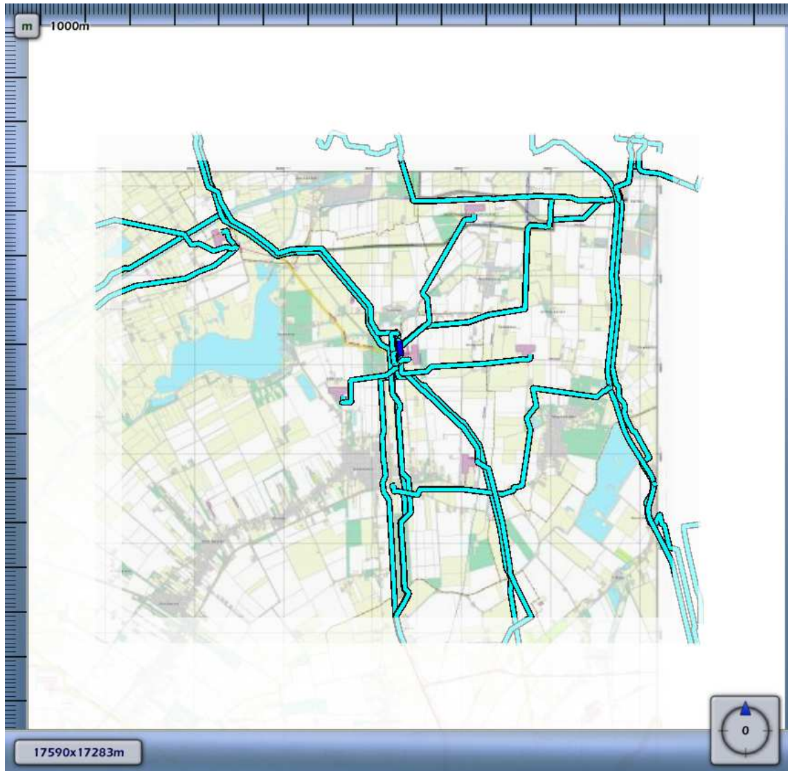
3.65 Figuur 3.65 Plaatsgebonden risico voor {E099BF5A-E453-4A9B-B3B7-392DC33A625A}_504115 van Nederlandse Aardolie Maatschappij BV
