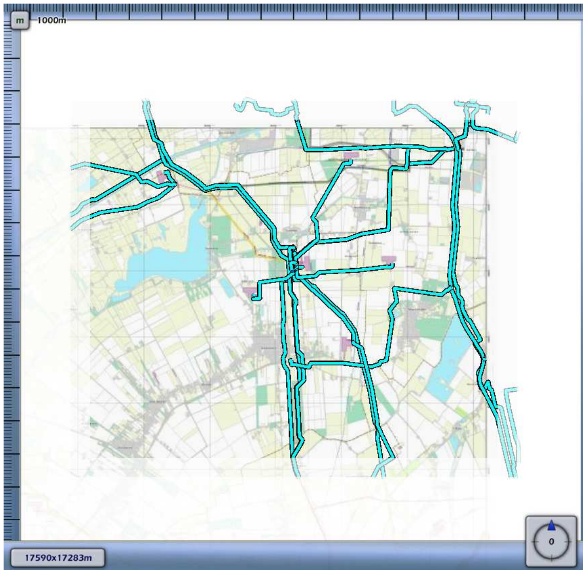
3.54 Figuur 3.54 Plaatsgebonden risico voor {E099BF5A-E453-4A9B-B3B7-392DC33A625A}_504068 van Nederlandse Aardolie Maatschappij BV
