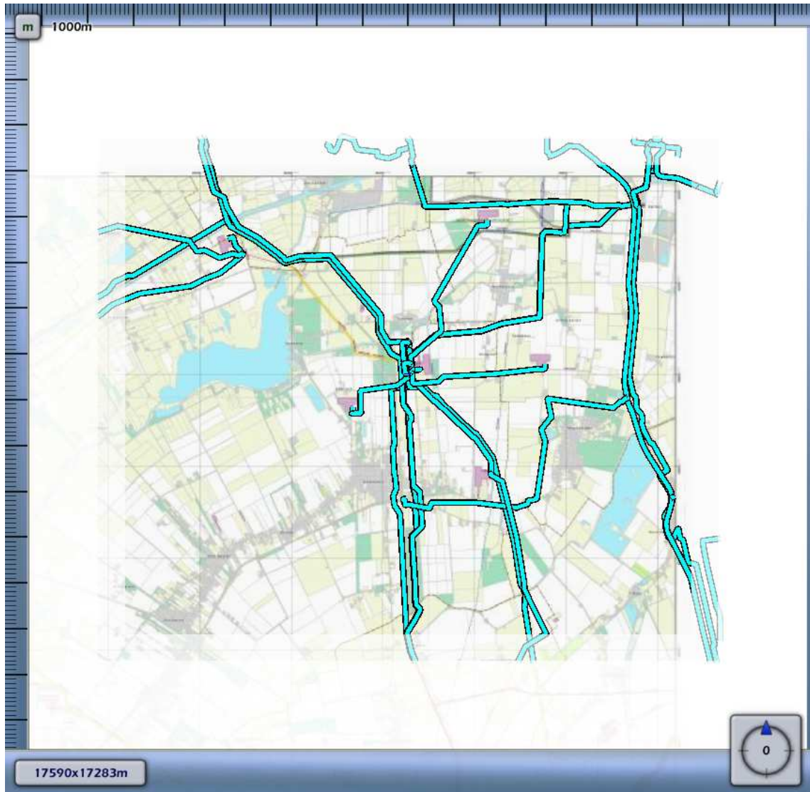
3.53 Figuur 3.53 Plaatsgebonden risico voor {E099BF5A-E453-4A9B-B3B7-392DC33A625A}_504067 van Nederlandse Aardolie Maatschappij BV
