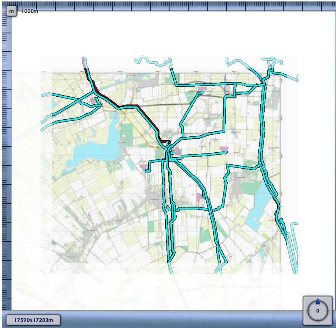
3.19 Figuur 3.19 Plaatsgebonden risico voor N-509-11 van N.V. Nederlandse Gasunie
