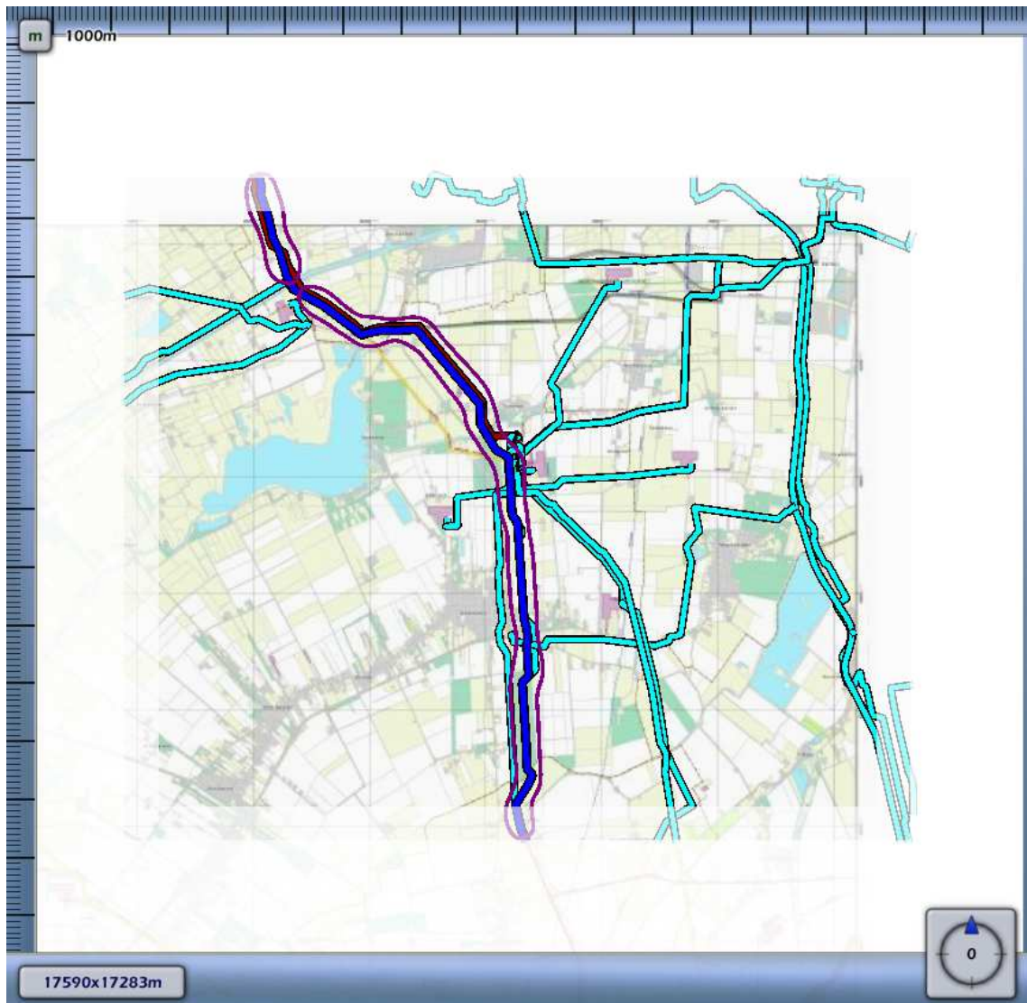
3.8 Figuur 3.8 Plaatsgebonden risico voor A-543 van N.V. Nederlandse Gasunie
