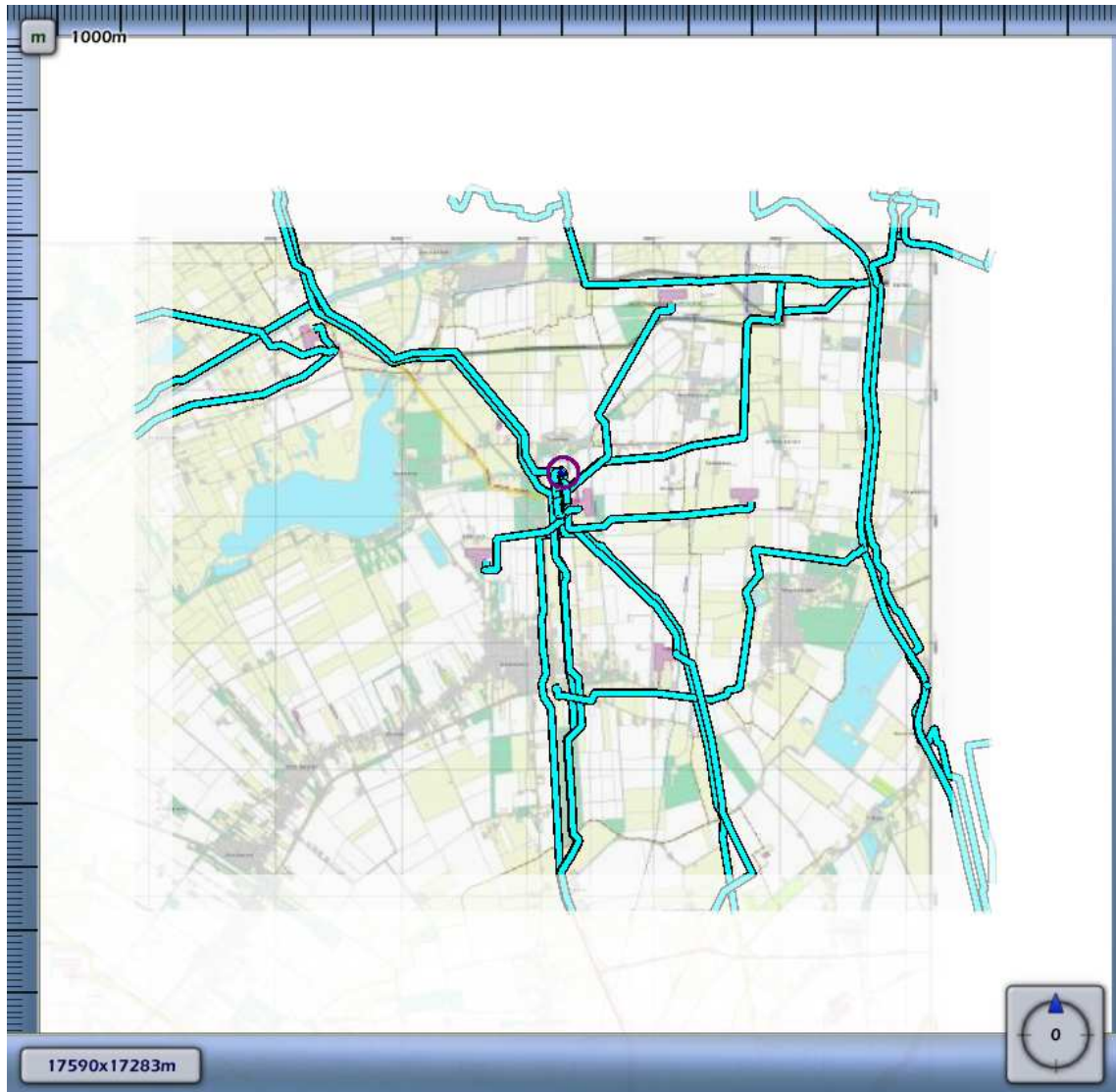
3.67 Figuur 3.67 Plaatsgebonden risico voor {E099BF5A-E453-4A9B-B3B7-392DC33A625A}_504119 van Nederlandse Aardolie Maatschappij BV
