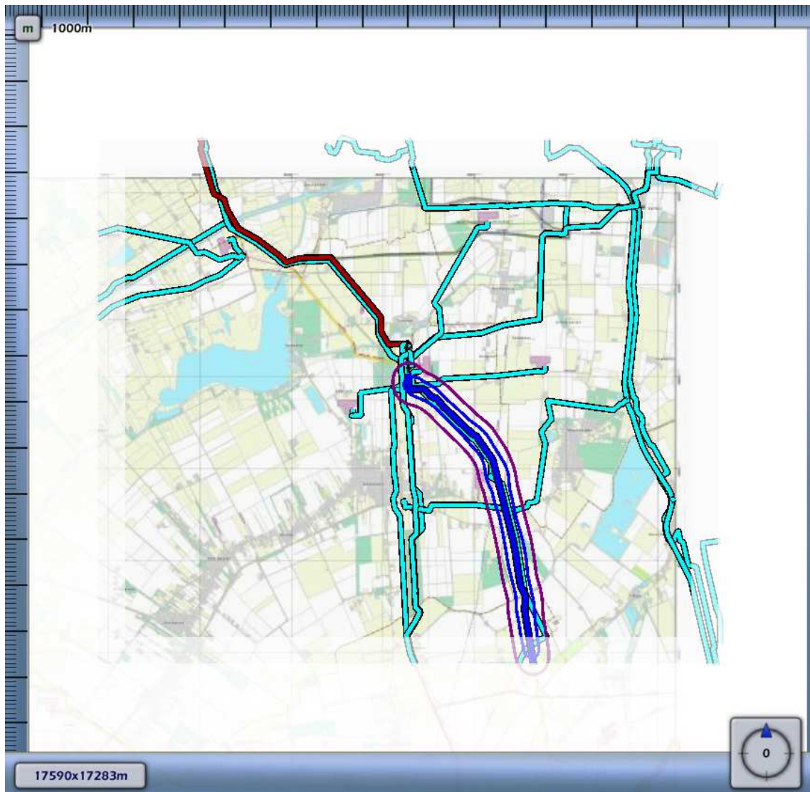
3.7 Figuur 3.7 Plaatsgebonden risico voor A-519 van N.V. Nederlandse Gasunie
