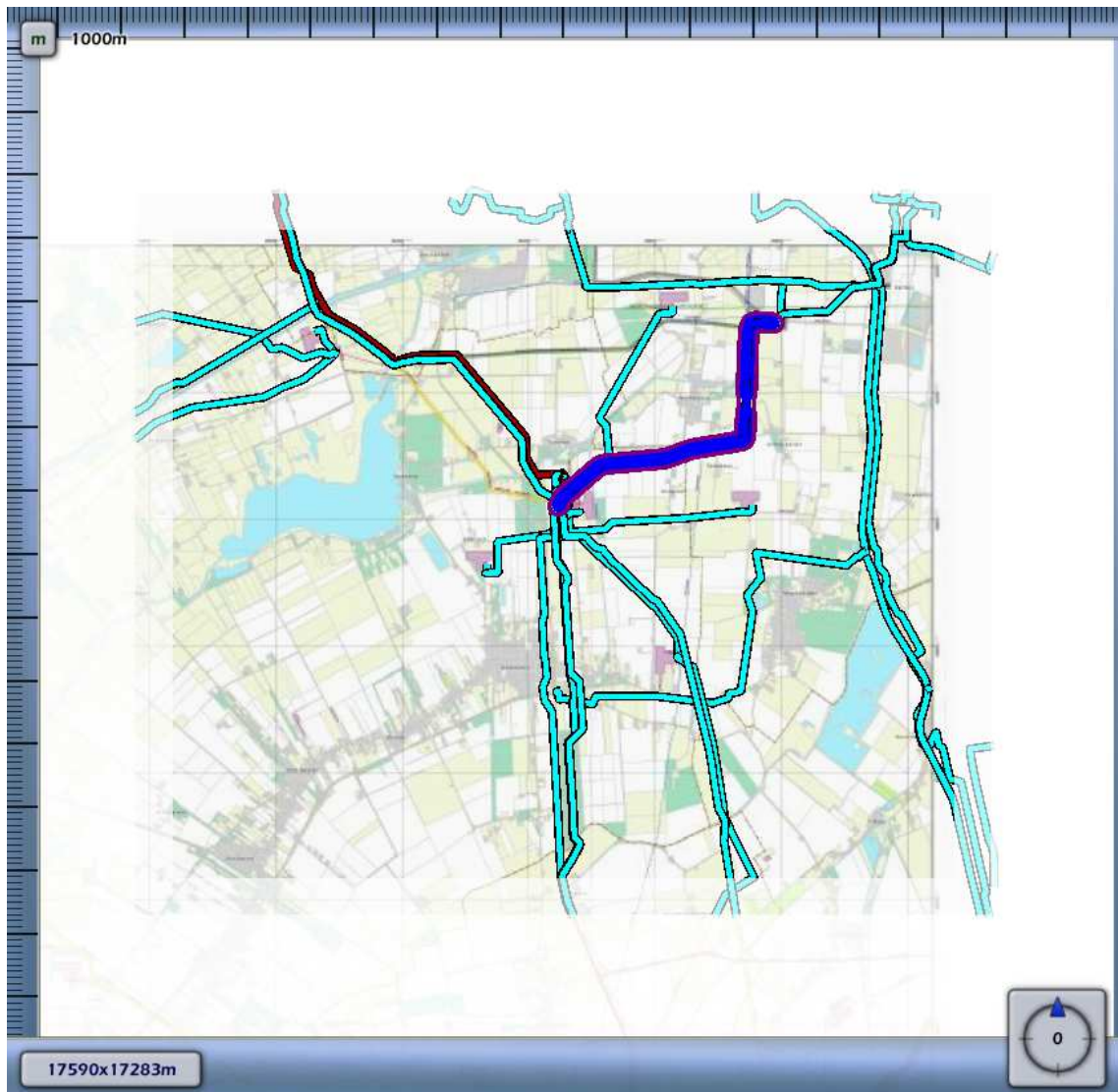
3.12 Figuur 3.12 Plaatsgebonden risico voor A-649 van N.V. Nederlandse Gasunie
