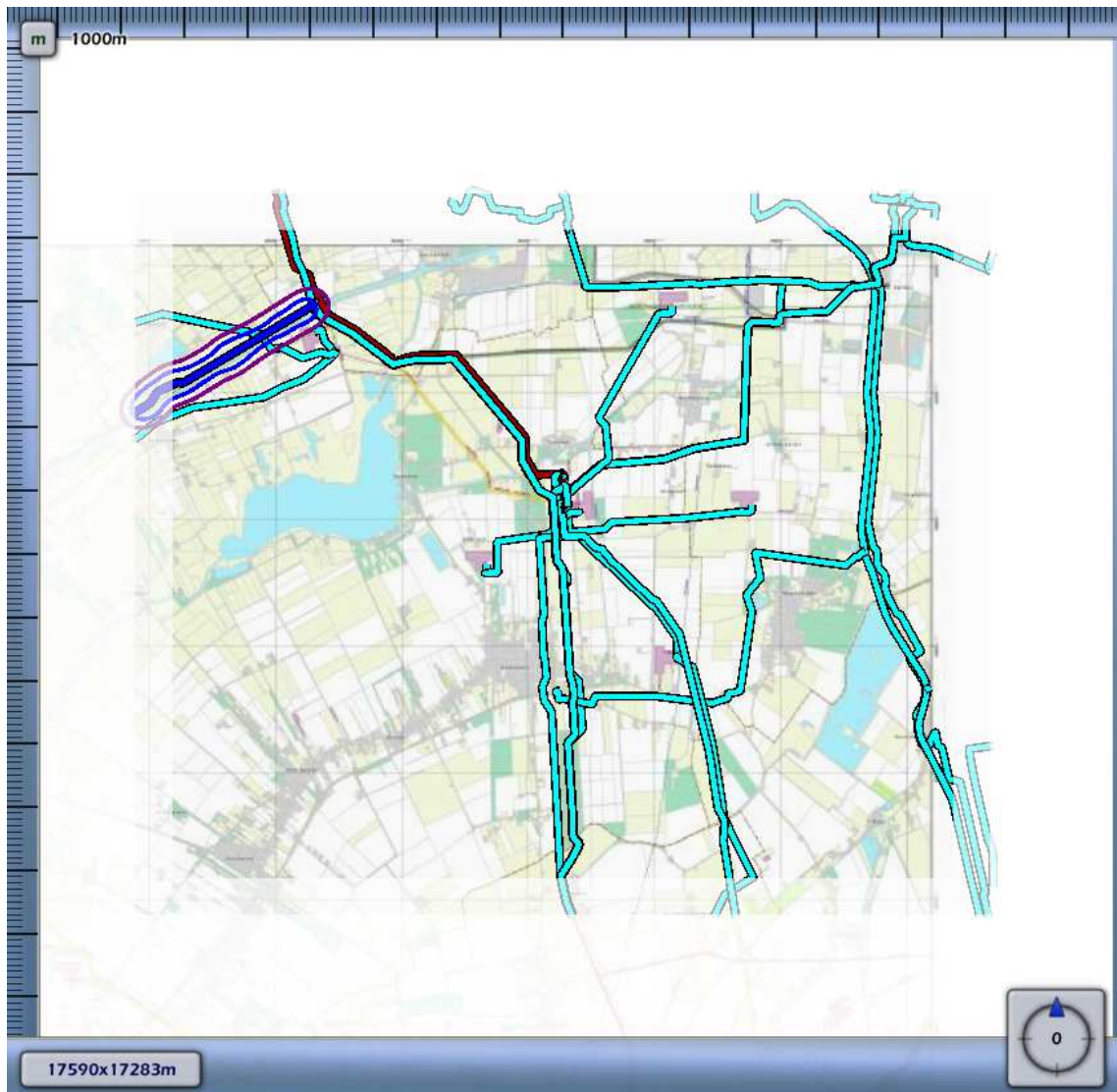
3.10 Figuur 3.10 Plaatsgebonden risico voor A-601 van N.V. Nederlandse Gasunie
