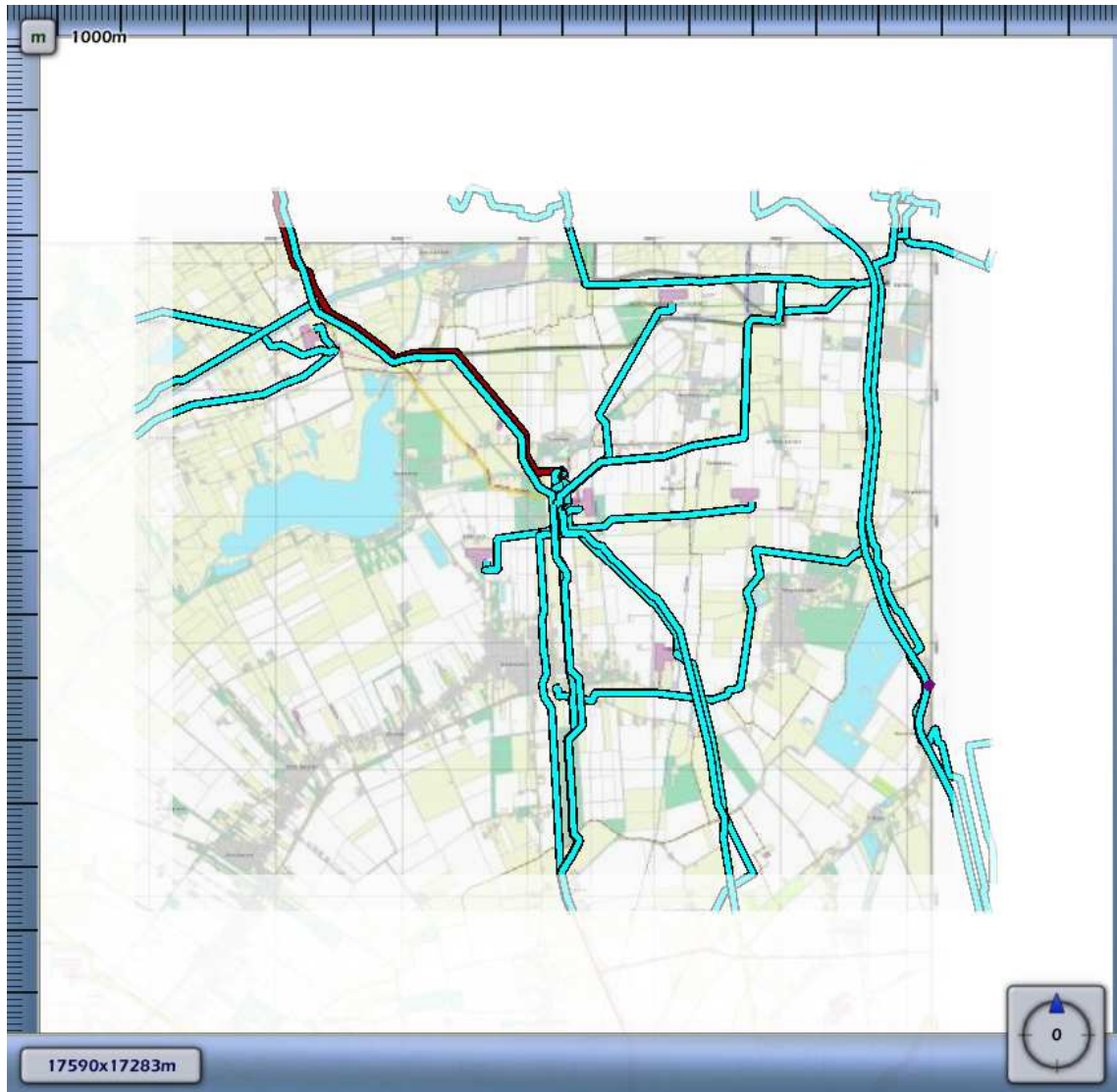
3.27 Figuur 3.27 Plaatsgebonden risico voor N-509-94 van N.V. Nederlandse Gasunie
