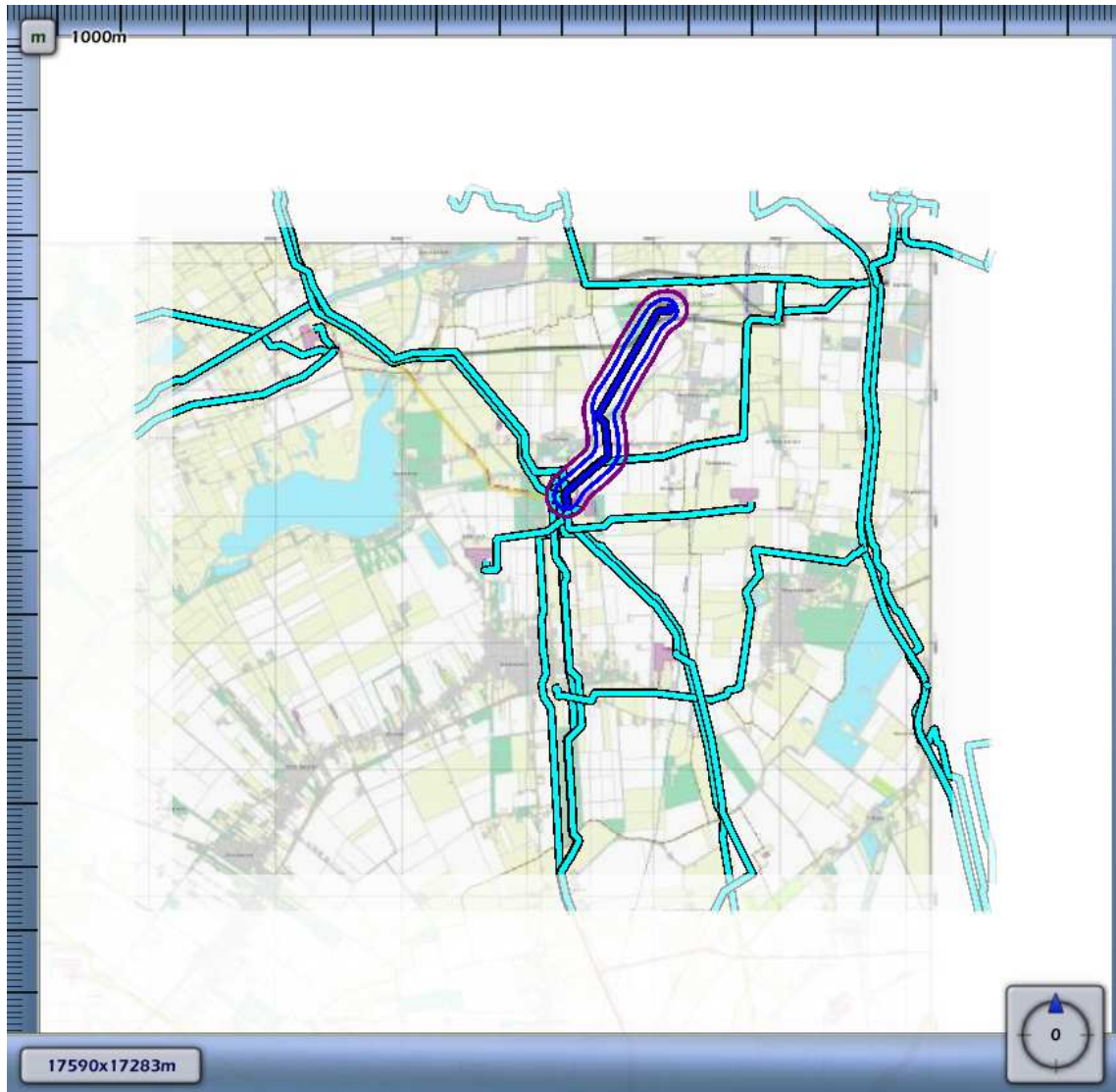
3.44 Figuur 3.44 Plaatsgebonden risico voor {E099BF5A-E453-4A9B-B3B7-392DC33A625A}_502230 van Nederlandse Aardolie Maatschappij BV
