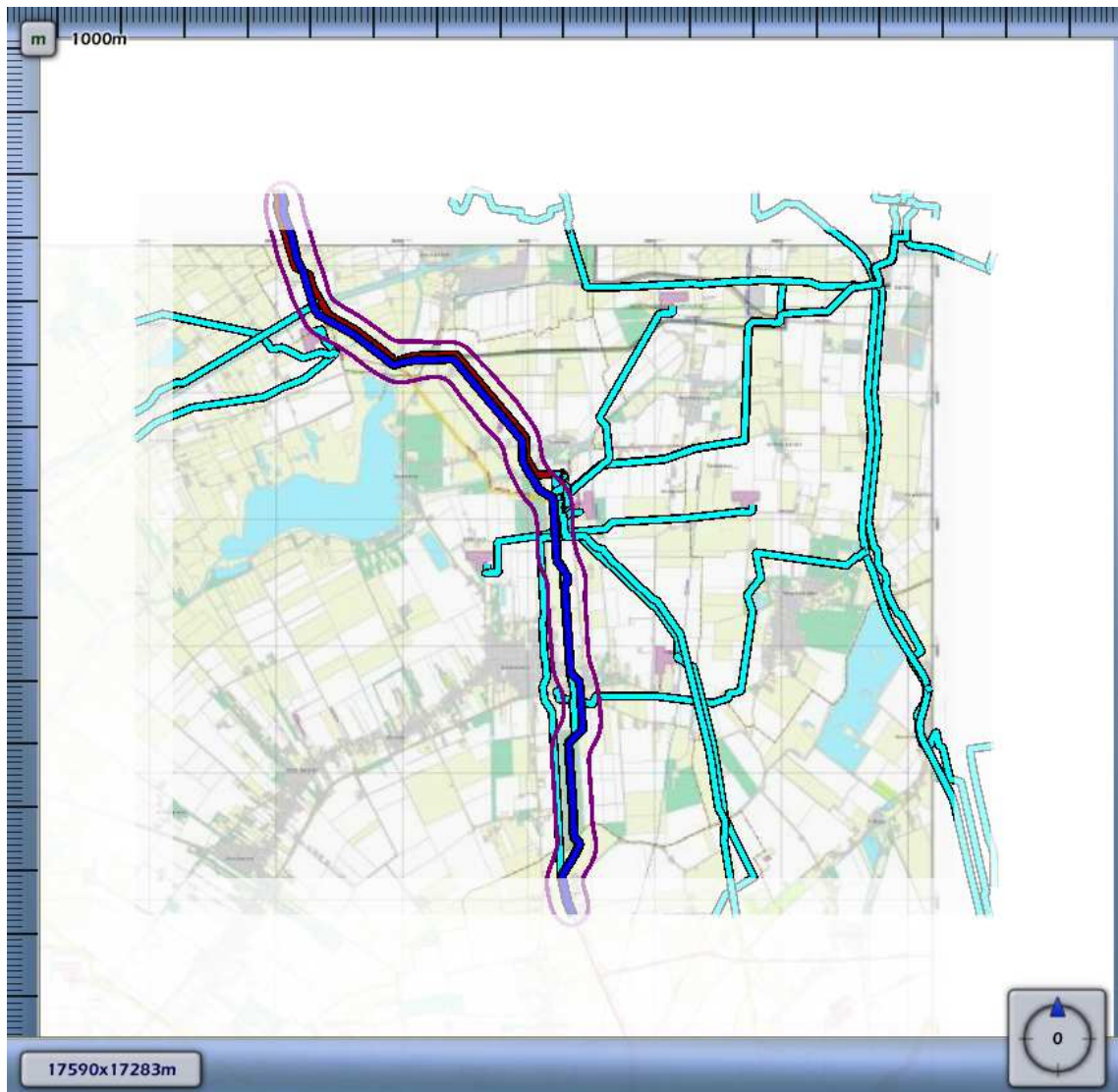
3.11 Figuur 3.11 Plaatsgebonden risico voor A-610 van N.V. Nederlandse Gasunie
