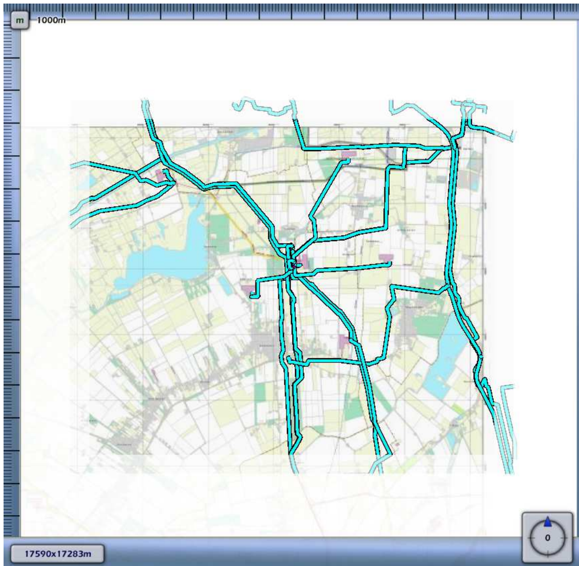
3.57 Figuur 3.57 Plaatsgebonden risico voor {E099BF5A-E453-4A9B-B3B7-392DC33A625A}_504102 van Nederlandse Aardolie Maatschappij BV
