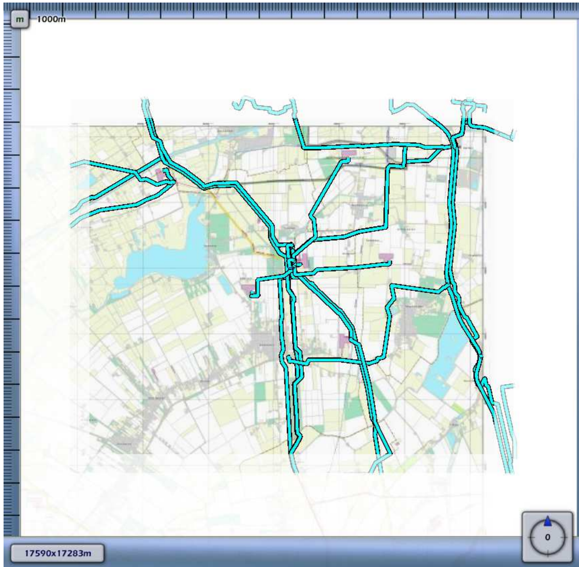
3.55 Figuur 3.55 Plaatsgebonden risico voor {E099BF5A-E453-4A9B-B3B7-392DC33A625A}_504069 van Nederlandse Aardolie Maatschappij BV
