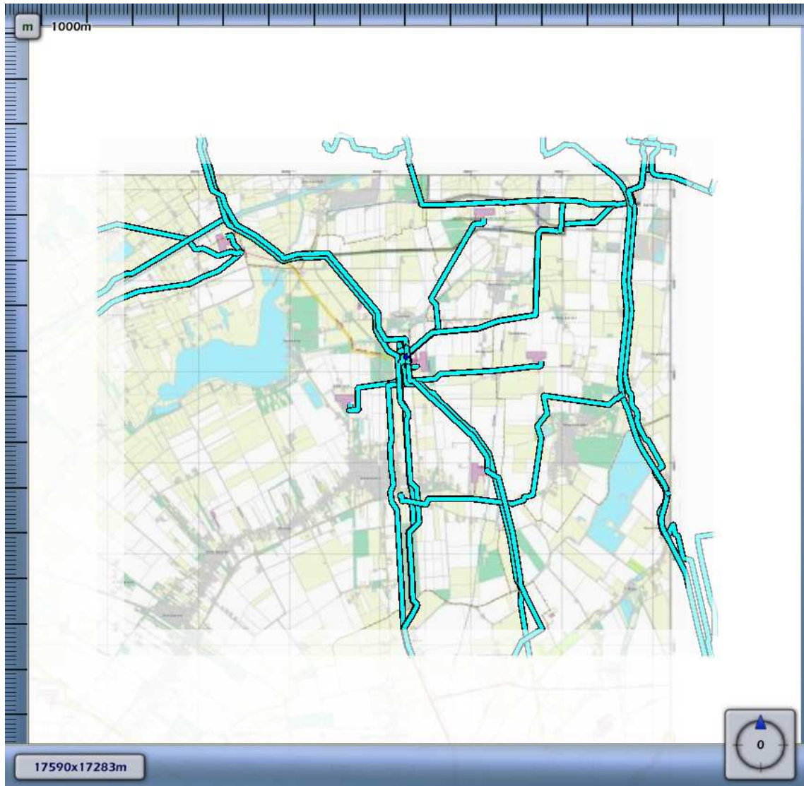
3.36 Figuur 3.36 Plaatsgebonden risico voor {E099BF5A-E453-4A9B-B3B7-392DC33A625A}_501066 van Nederlandse Aardolie Maatschappij BV
