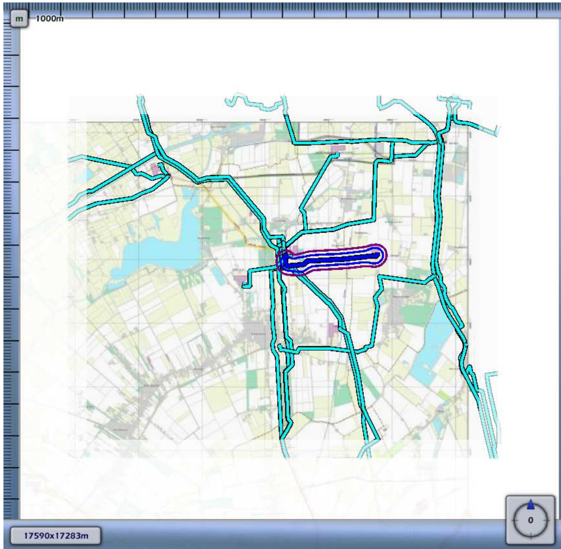
3.43 Figuur 3.43 Plaatsgebonden risico voor {E099BF5A-E453-4A9B-B3B7-392DC33A625A}_502220 van Nederlandse Aardolie Maatschappij BV
