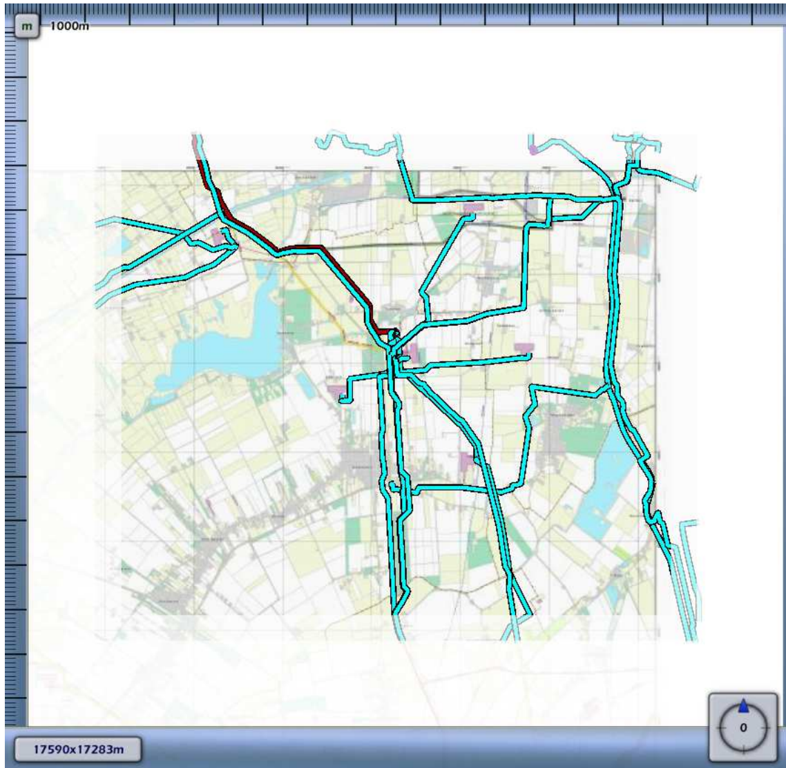
3.23 Figuur 3.23 Plaatsgebonden risico voor N-509-82 van N.V. Nederlandse Gasunie
