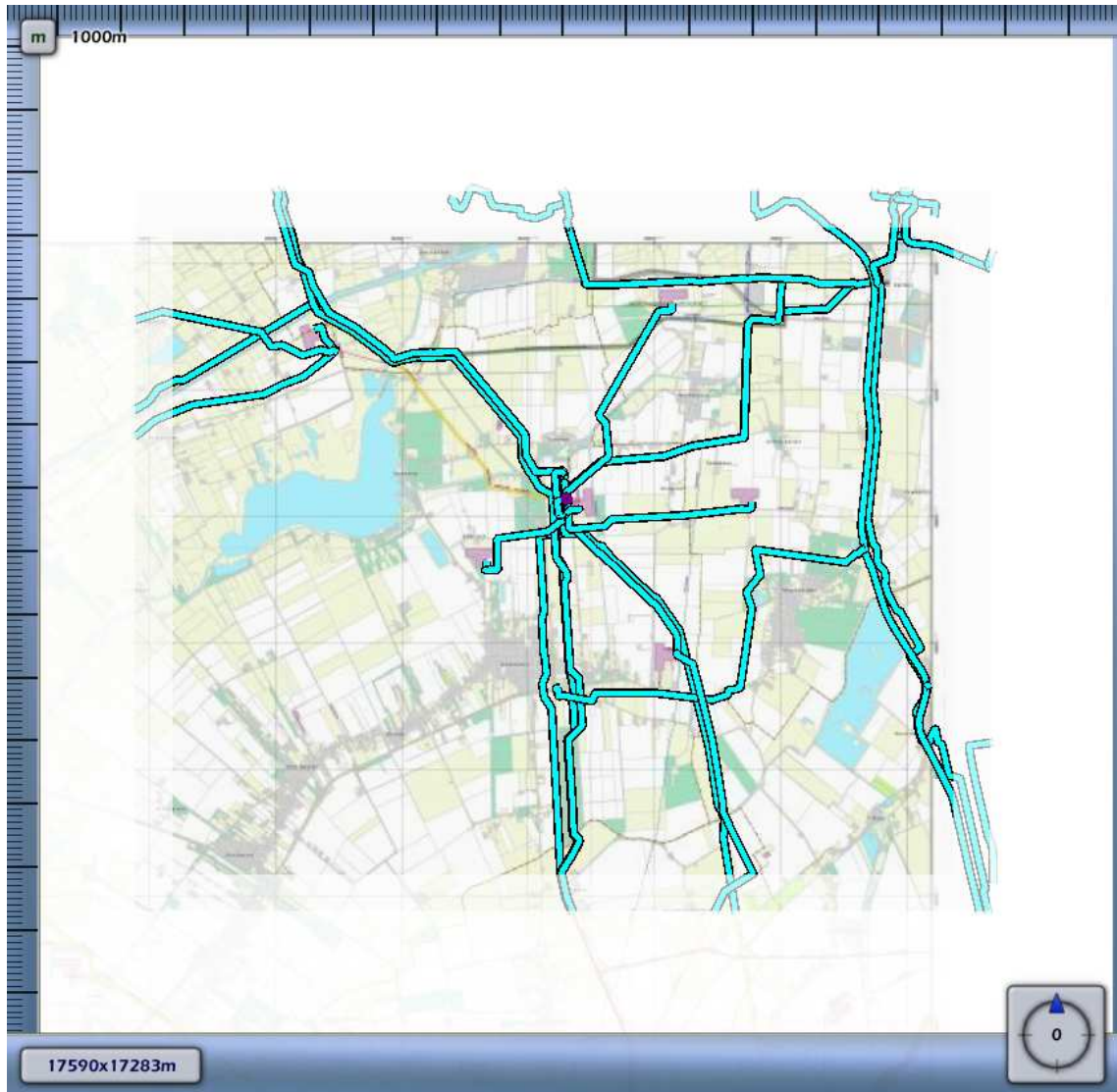
3.64 Figuur 3.64 Plaatsgebonden risico voor {E099BF5A-E453-4A9B-B3B7-392DC33A625A}_504113 van Nederlandse Aardolie Maatschappij BV
