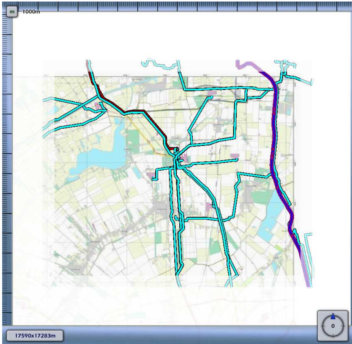
3.26 Figuur 3.26 Plaatsgebonden risico voor N-509-90 van N.V. Nederlandse Gasunie
