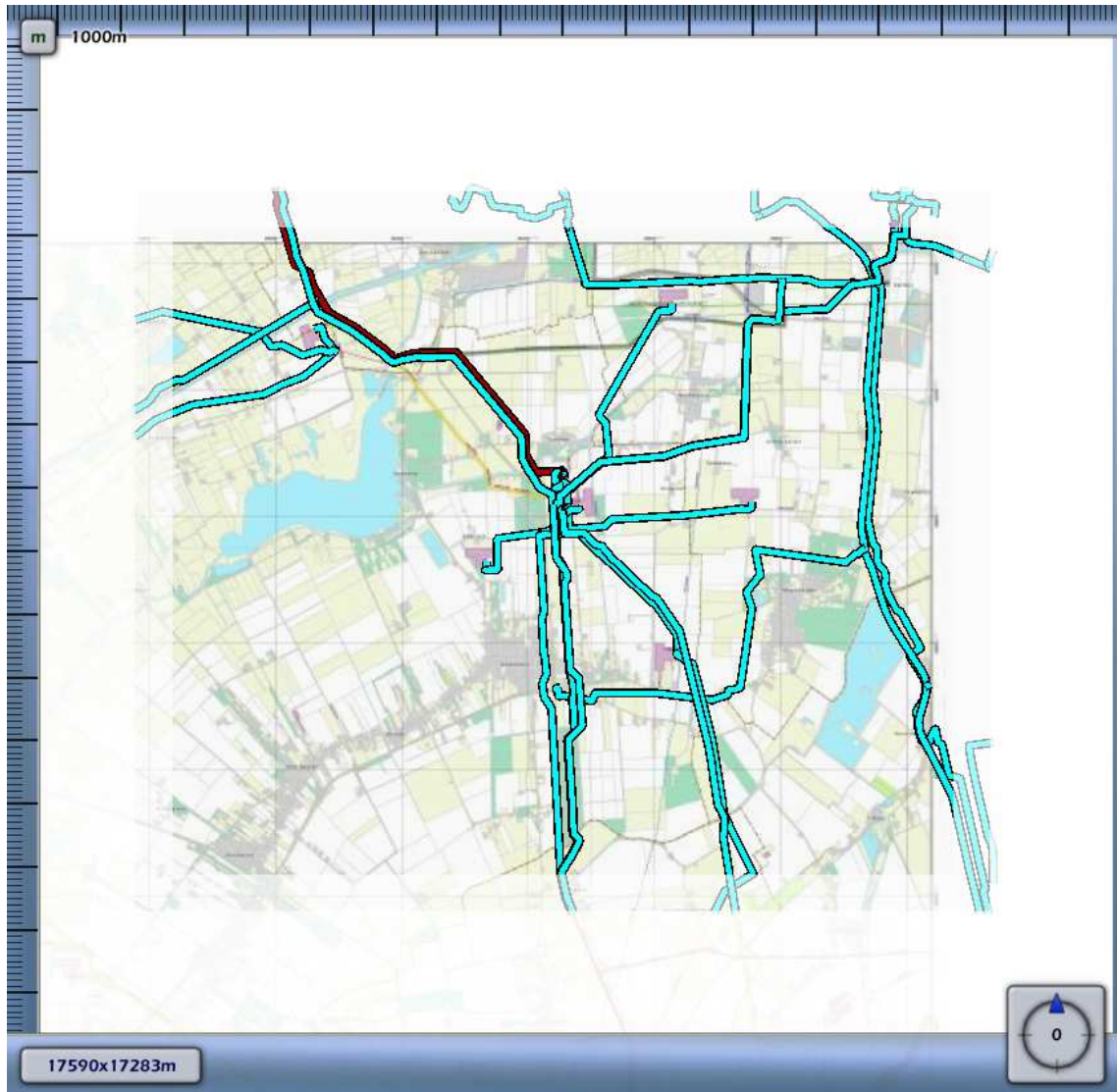
3.17 Figuur 3.17 Plaatsgebonden risico voor N-509-08 van N.V. Nederlandse Gasunie
