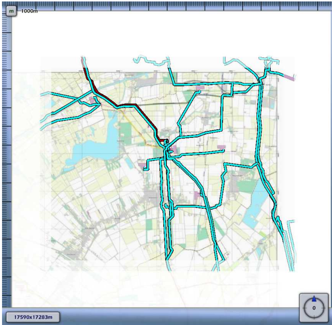
3.18 Figuur 3.18 Plaatsgebonden risico voor N-509-10 van N.V. Nederlandse Gasunie
