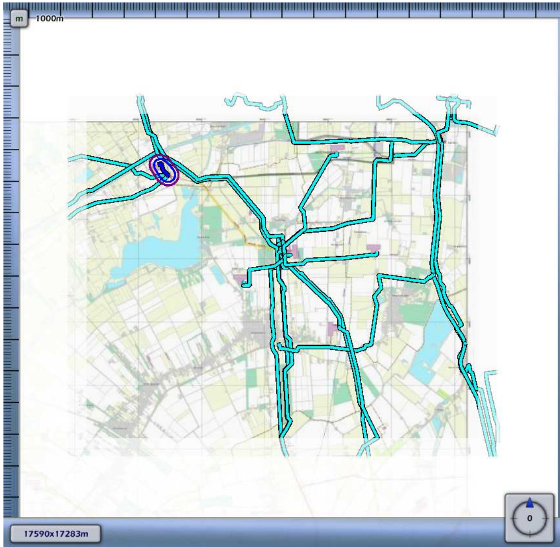
3.45 Figuur 3.45 Plaatsgebonden risico voor {E099BF5A-E453-4A9B-B3B7-392DC33A625A}_502240 van Nederlandse Aardolie Maatschappij BV
