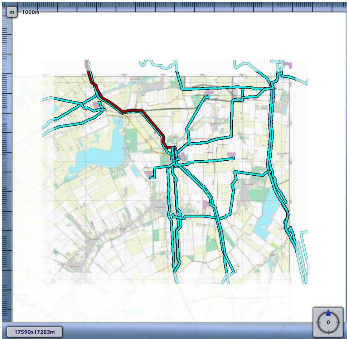
3.4 Figuur 3.4 Plaatsgebonden risico voor A-509-13 van N.V. Nederlandse Gasunie
