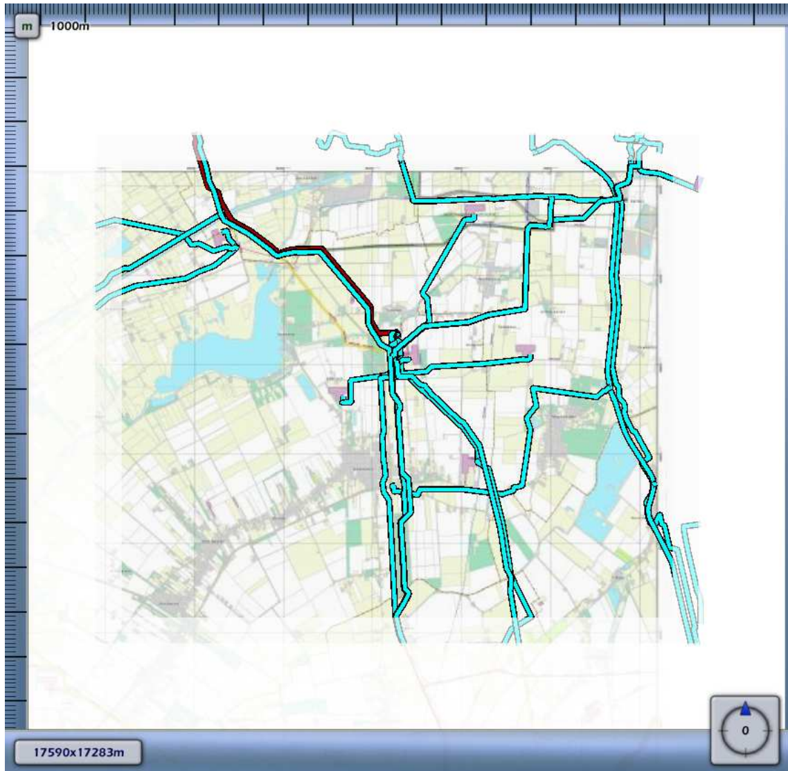
3.20 Figuur 3.20 Plaatsgebonden risico voor N-509-13 van N.V. Nederlandse Gasunie
