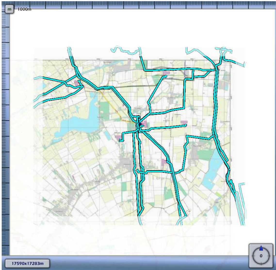
3.62 Figuur 3.62 Plaatsgebonden risico voor {E099BF5A-E453-4A9B-B3B7-392DC33A625A}_504111 van Nederlandse Aardolie Maatschappij BV
