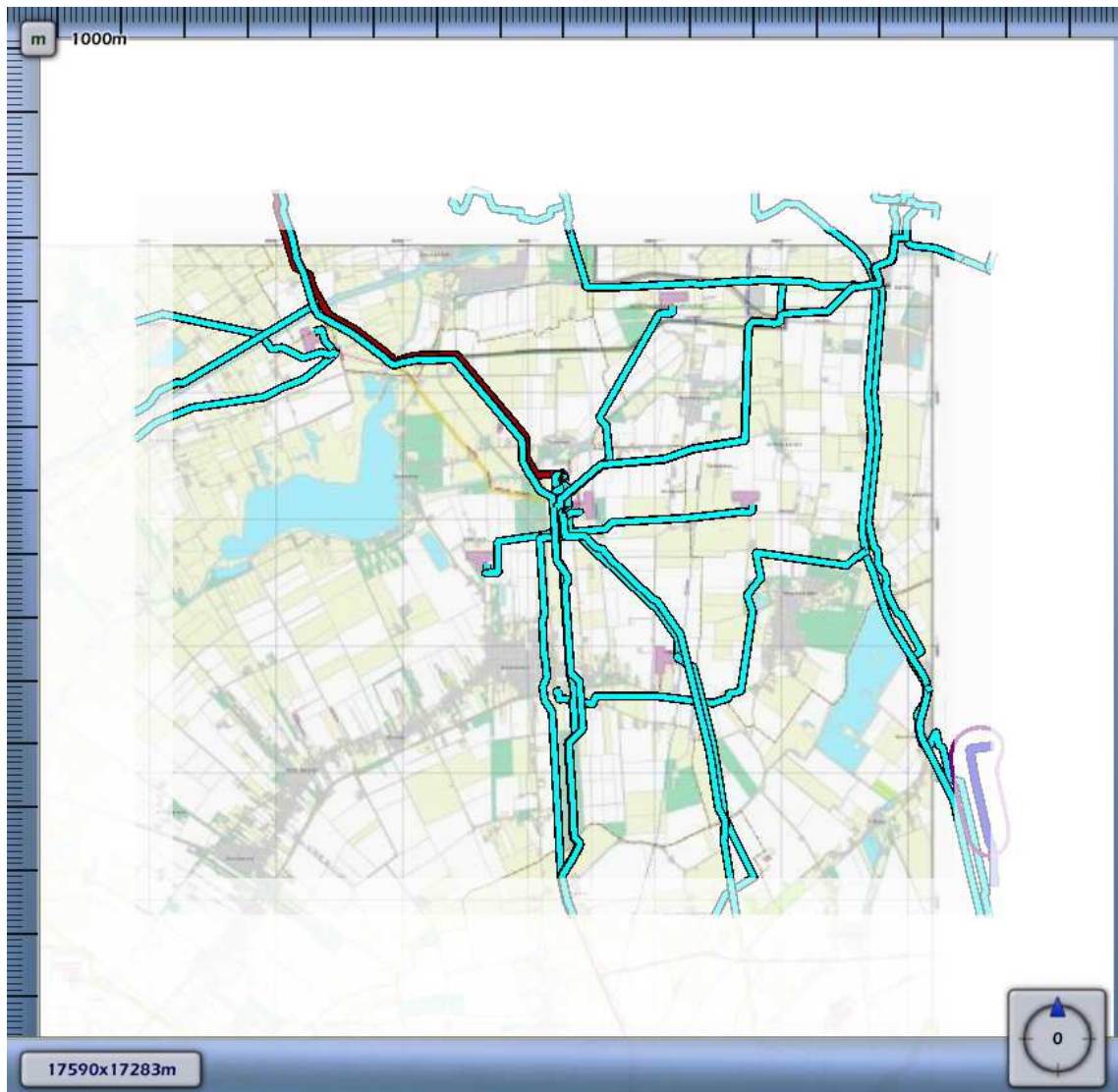
3.13 Figuur 3.13 Plaatsgebonden risico voor A-660 van N.V. Nederlandse Gasunie
