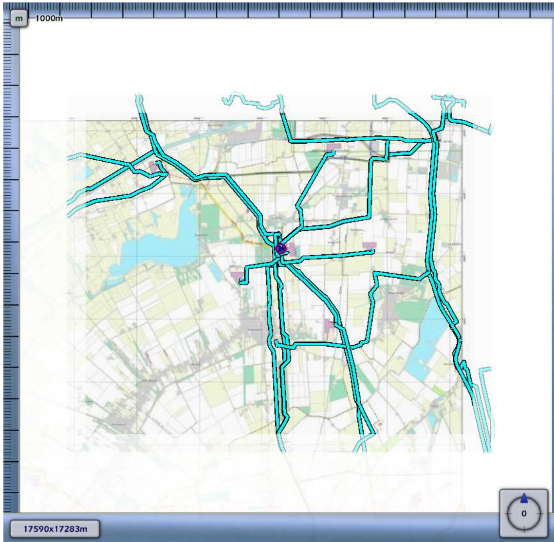
3.59 Figuur 3.59 Plaatsgebonden risico voor {E099BF5A-E453-4A9B-B3B7-392DC33A625A}_504108 van Nederlandse Aardolie Maatschappij BV
