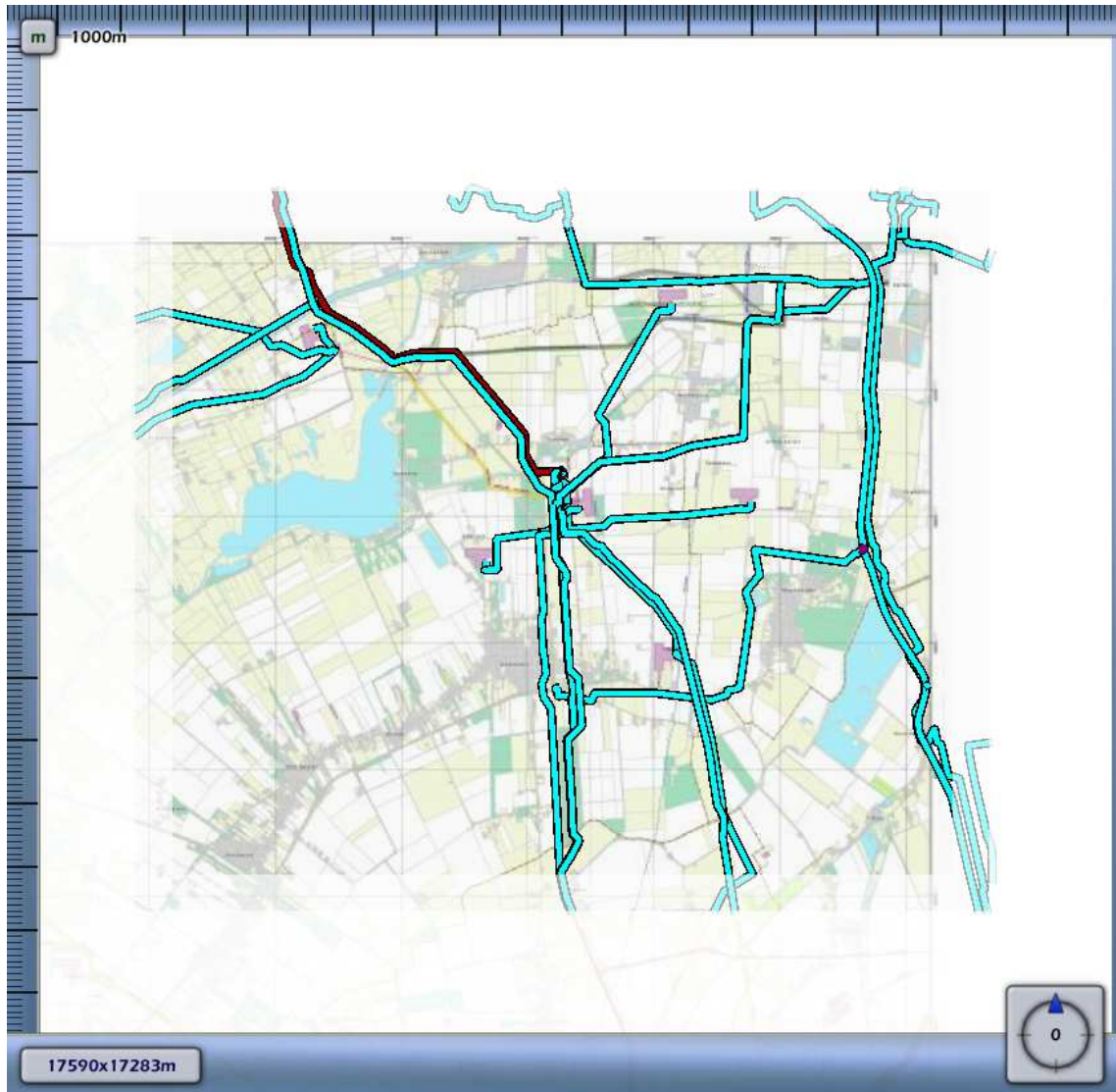
3.28 Figuur 3.28 Plaatsgebonden risico voor N-509-95 van N.V. Nederlandse Gasunie
