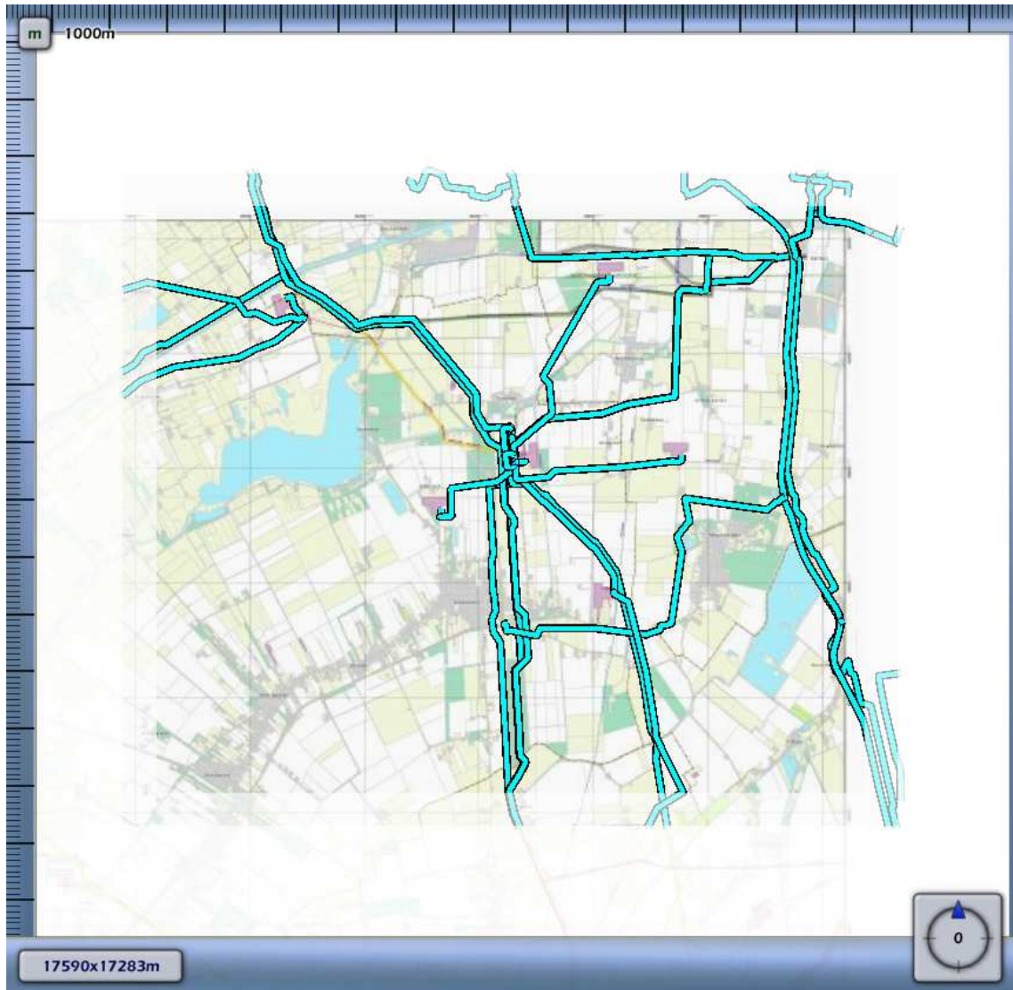
3.49 Figuur 3.49 Plaatsgebonden risico voor {E099BF5A-E453-4A9B-B3B7-392DC33A625A}_504063 van Nederlandse Aardolie Maatschappij BV
