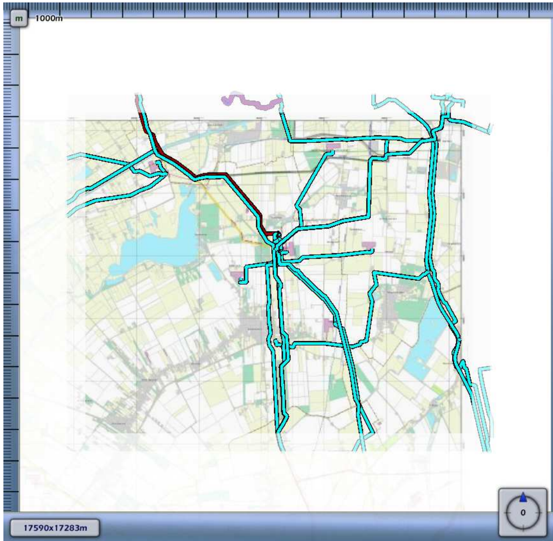
3.15 Figuur 3.15 Plaatsgebonden risico voor N-509-04 van N.V. Nederlandse Gasunie
