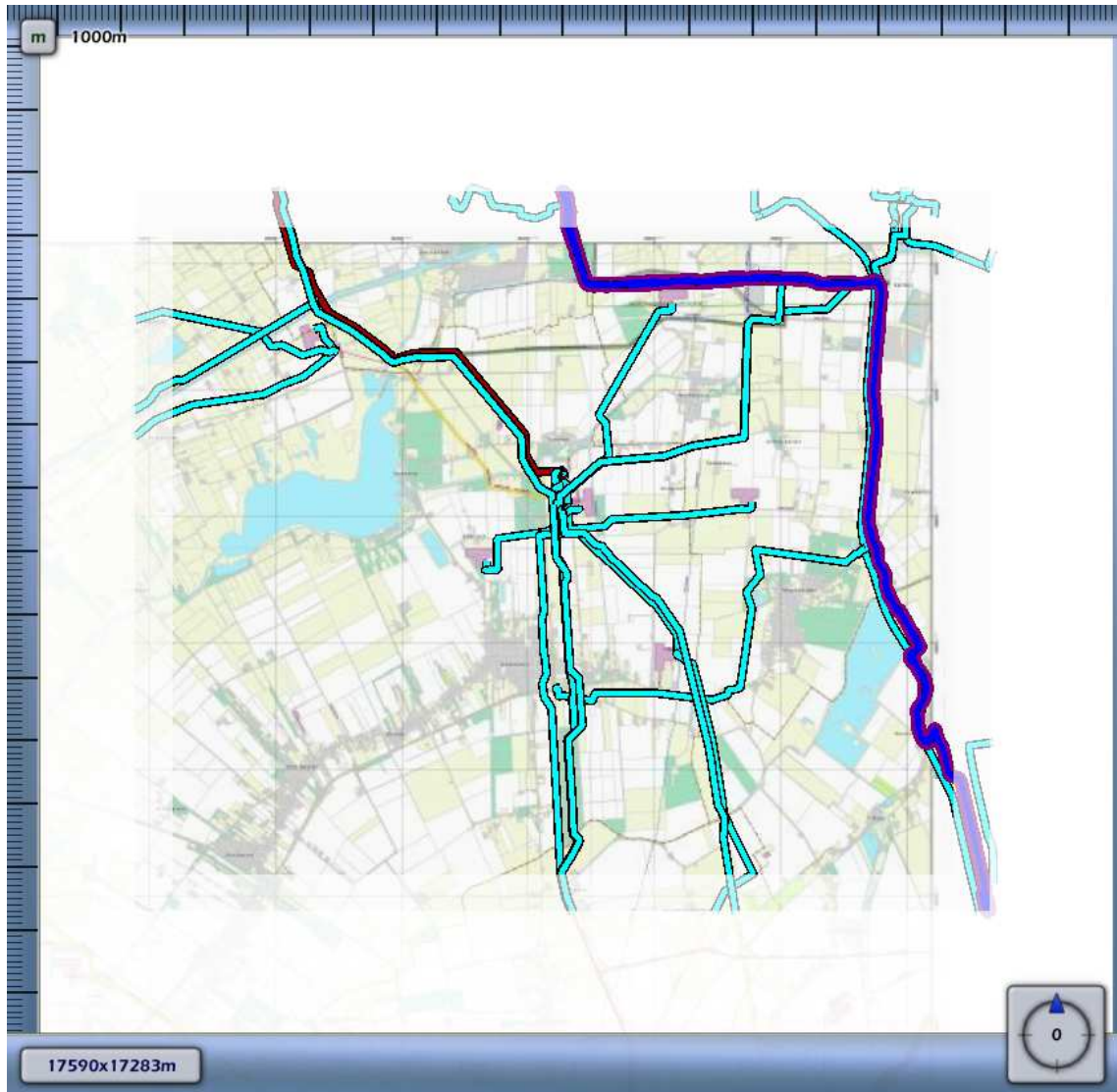
3.21 Figuur 3.21 Plaatsgebonden risico voor N-509-40 van N.V. Nederlandse Gasunie
