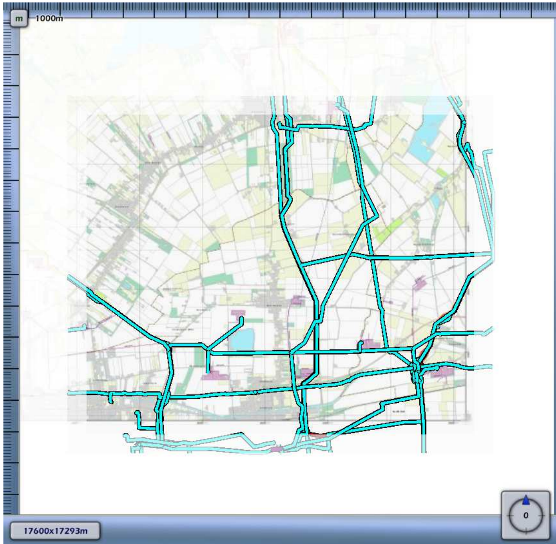
3.83 Figuur 3.83 Plaatsgebonden risico voor {80644C55-96F8-4492-9335-14F7A9767442}_505055 van Nederlandse Aardolie Maatschappij BV
