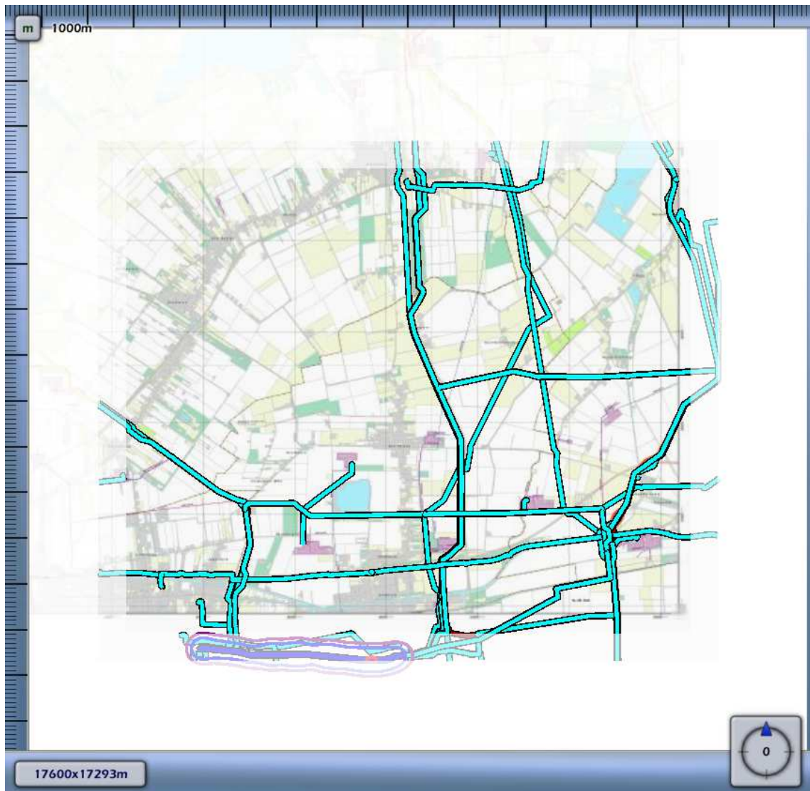
3.47 Figuur 3.47 Plaatsgebonden risico voor {80644C55-96F8-4492-9335-14F7A9767442}_501025 van Nederlandse Aardolie Maatschappij BV
