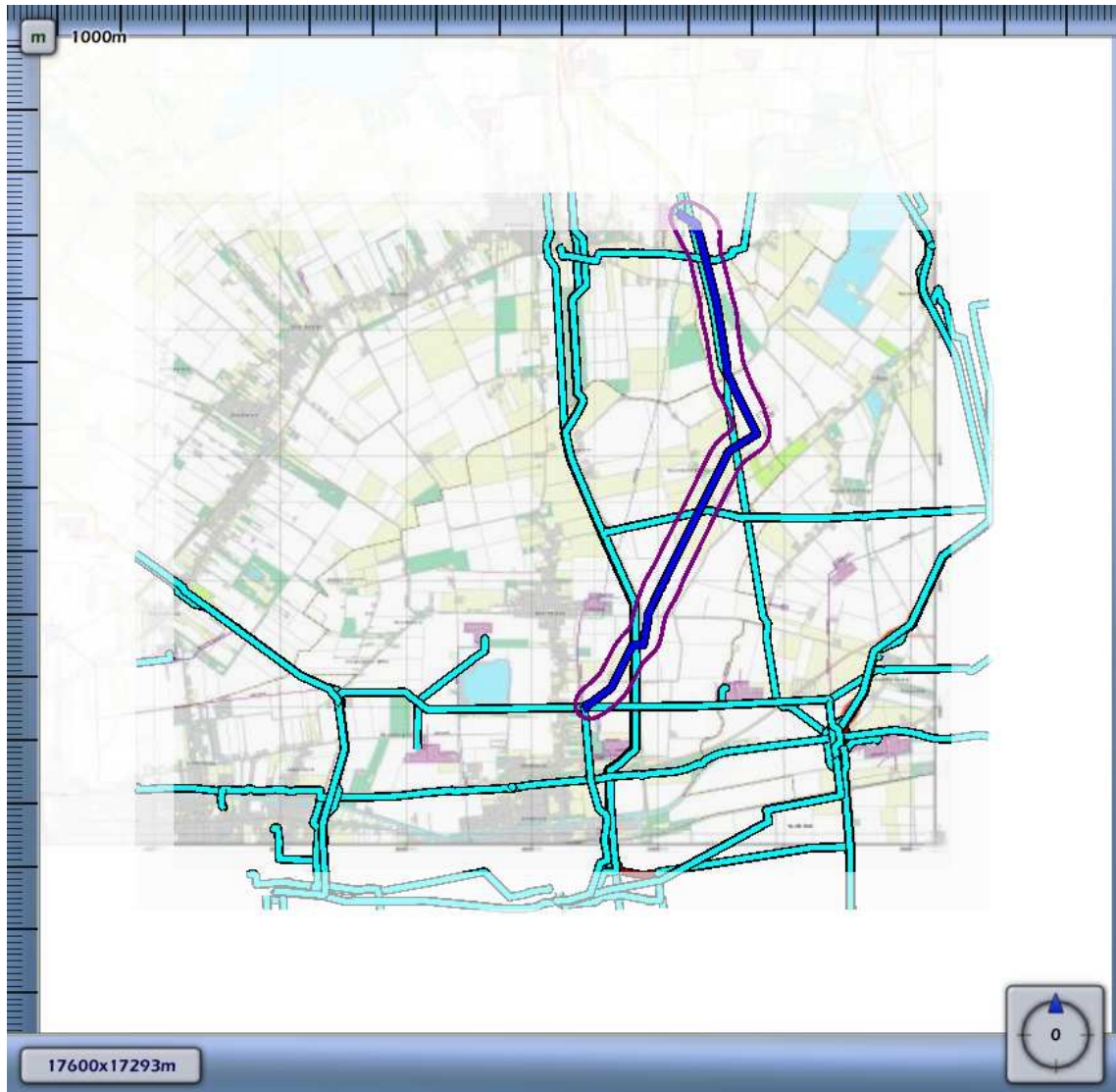
3.53 Figuur 3.53 Plaatsgebonden risico voor {80644C55-96F8-4492-9335-14F7A9767442}_501065 van Nederlandse Aardolie Maatschappij BV
