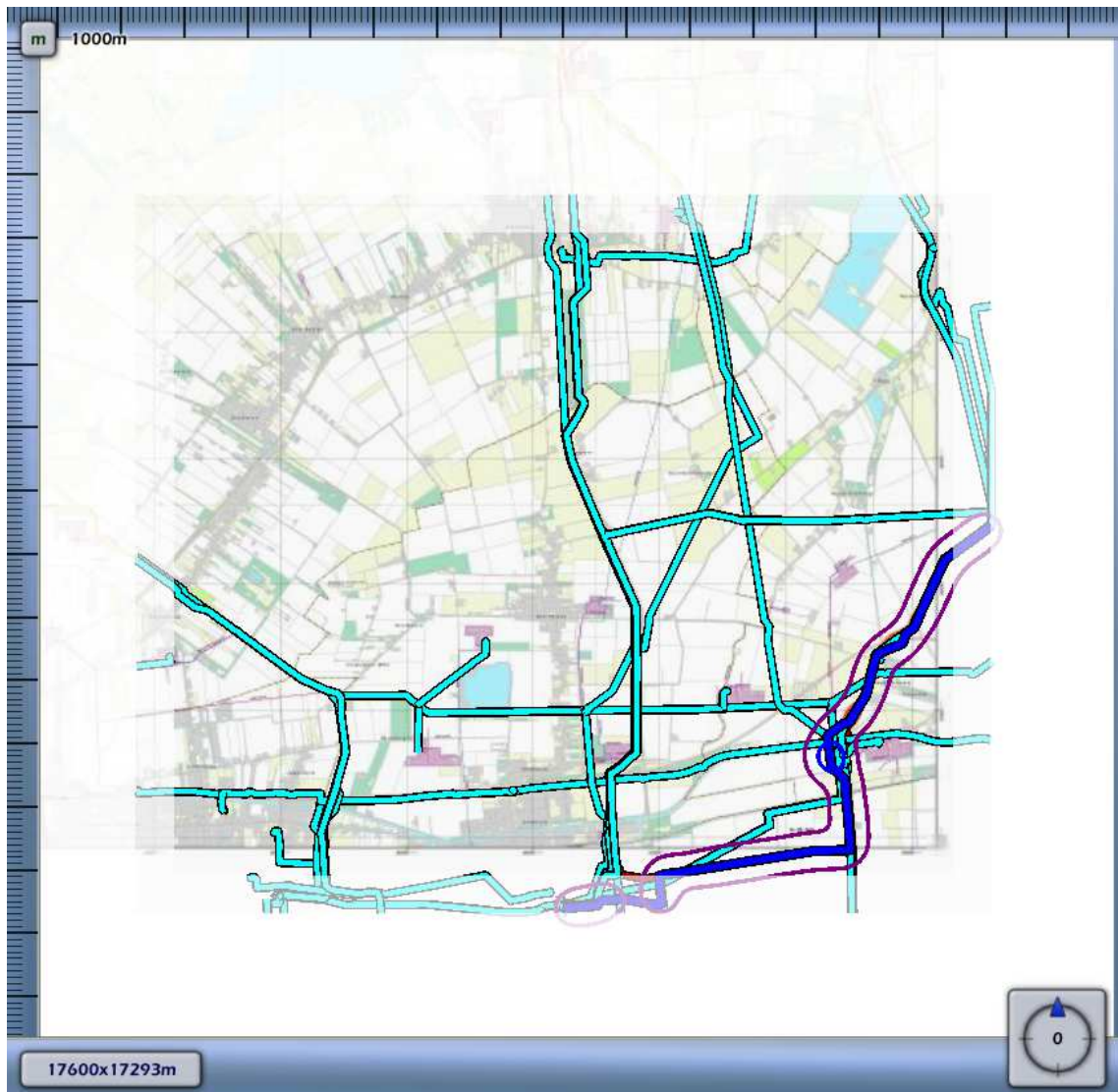
3.22 Figuur 3.22 Plaatsgebonden risico voor A-666 van N.V. Nederlandse Gasunie
