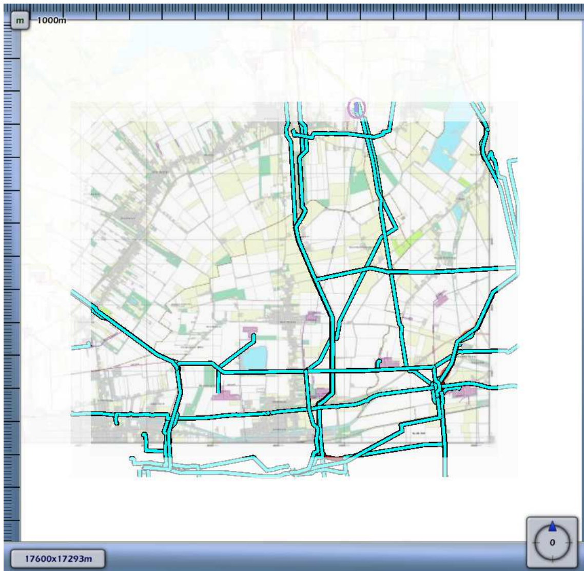
3.52 Figuur 3.52 Plaatsgebonden risico voor {80644C55-96F8-4492-9335-14F7A9767442}_501063 van Nederlandse Aardolie Maatschappij BV
