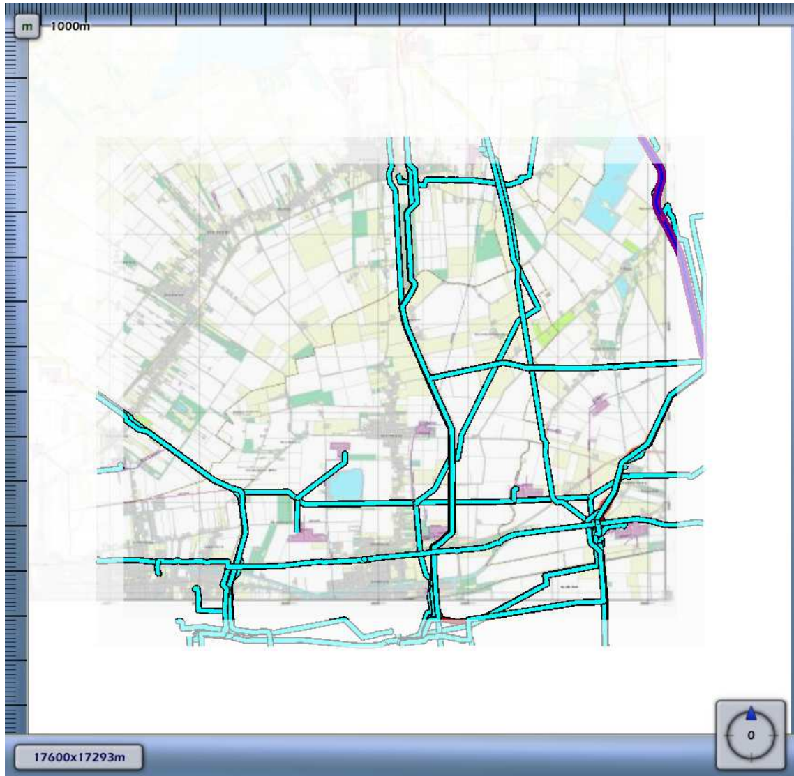
3.33 Figuur 3.33 Plaatsgebonden risico voor N-509-90 van N.V. Nederlandse Gasunie
