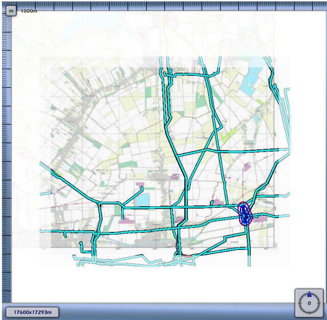
3.45 Figuur 3.45 Plaatsgebonden risico voor {80644C55-96F8-4492-9335-14F7A9767442}_501023 van Nederlandse Aardolie Maatschappij BV
