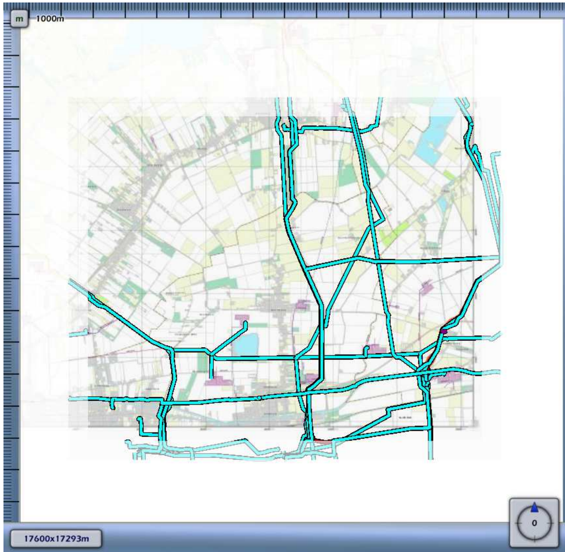
3.29 Figuur 3.29 Plaatsgebonden risico voor N-509-03 van N.V. Nederlandse Gasunie
