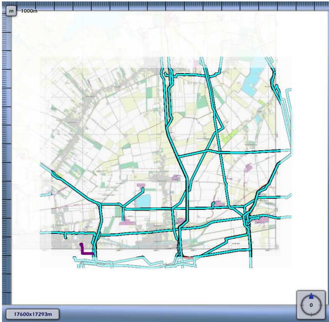
3.23 Figuur 3.23 Plaatsgebonden risico voor N-508-04 van N.V. Nederlandse Gasunie
