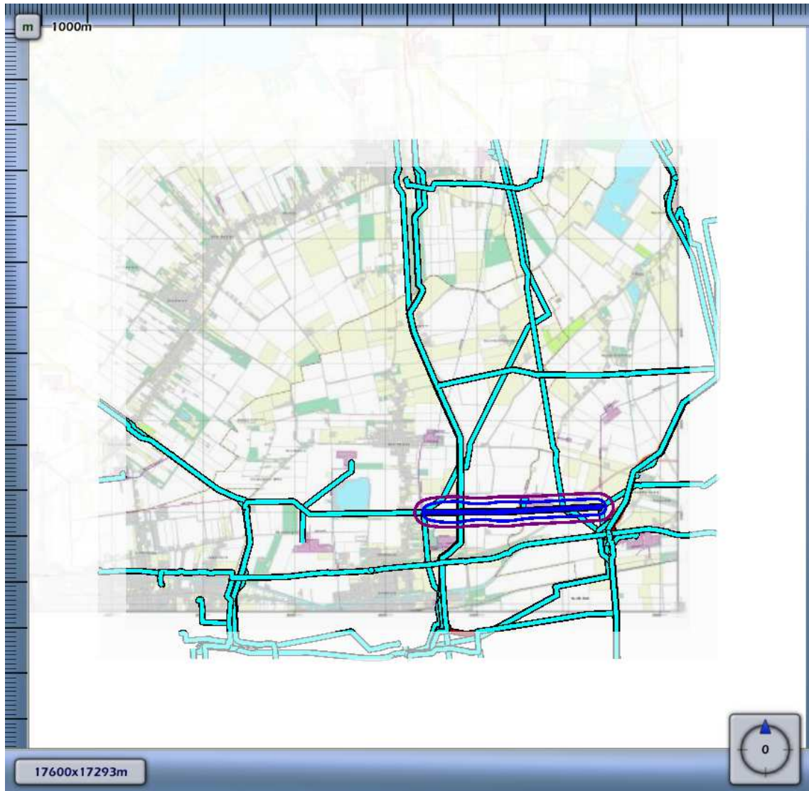
3.38 Figuur 3.38 Plaatsgebonden risico voor {80644C55-96F8-4492-9335-14F7A9767442}_501012 van Nederlandse Aardolie Maatschappij BV
