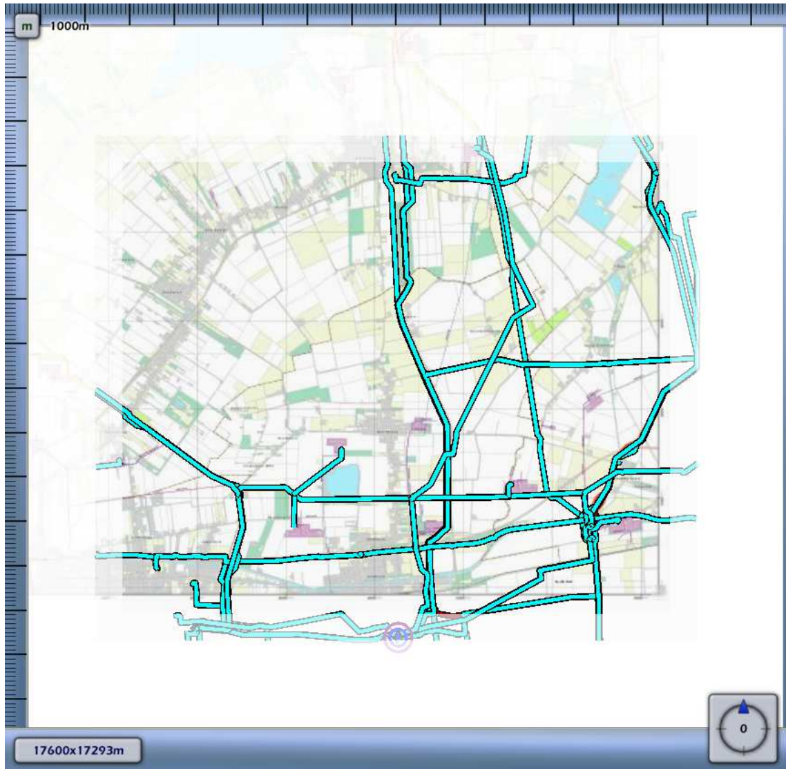
3.80 Figuur 3.80 Plaatsgebonden risico voor {80644C55-96F8-4492-9335-14F7A9767442}_504080 van Nederlandse Aardolie Maatschappij BV
