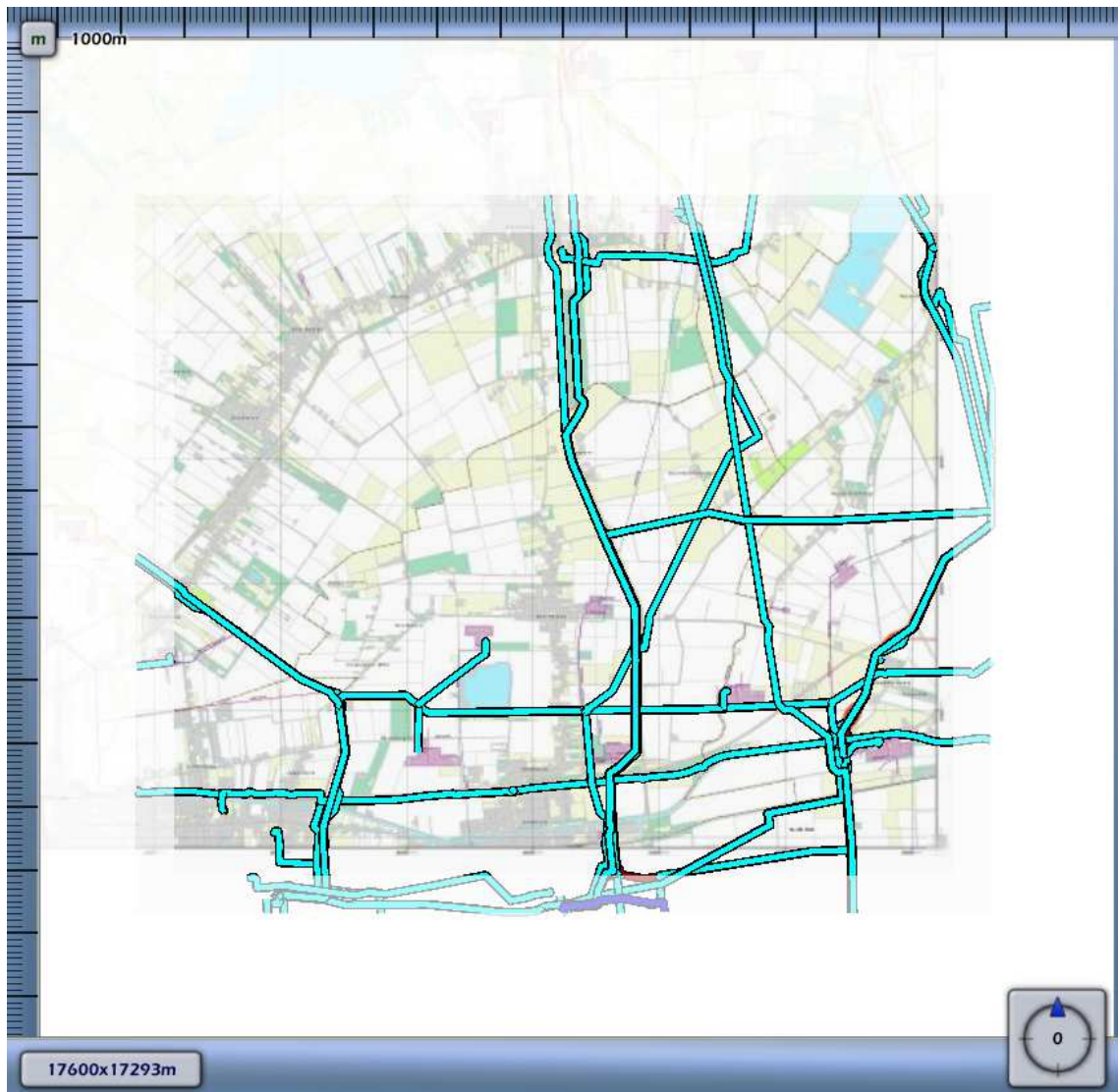
3.13 Figuur 3.13 Plaatsgebonden risico voor A-590 van N.V. Nederlandse Gasunie
