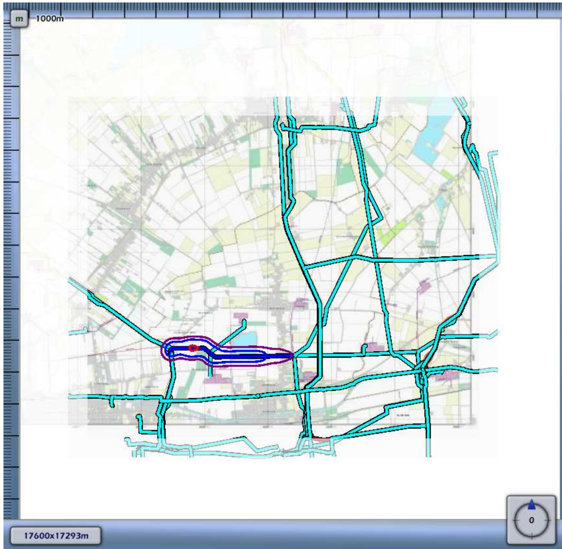
3.37 Figuur 3.37 Plaatsgebonden risico voor {80644C55-96F8-4492-9335-14F7A9767442}_501011 van Nederlandse Aardolie Maatschappij BV
