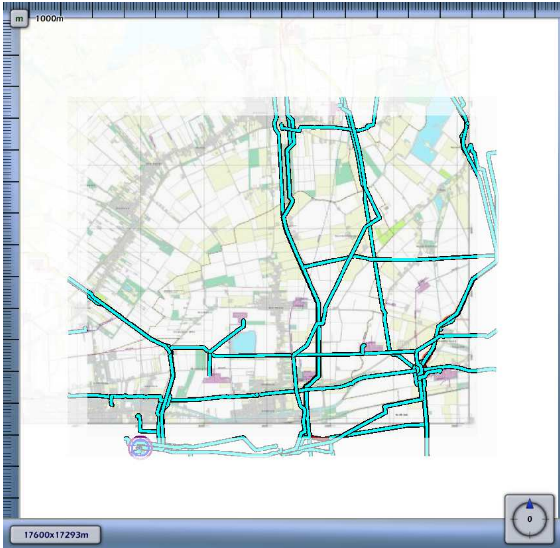
3.66 Figuur 3.66 Plaatsgebonden risico voor {80644C55-96F8-4492-9335-14F7A9767442}_504013 van Nederlandse Aardolie Maatschappij BV
