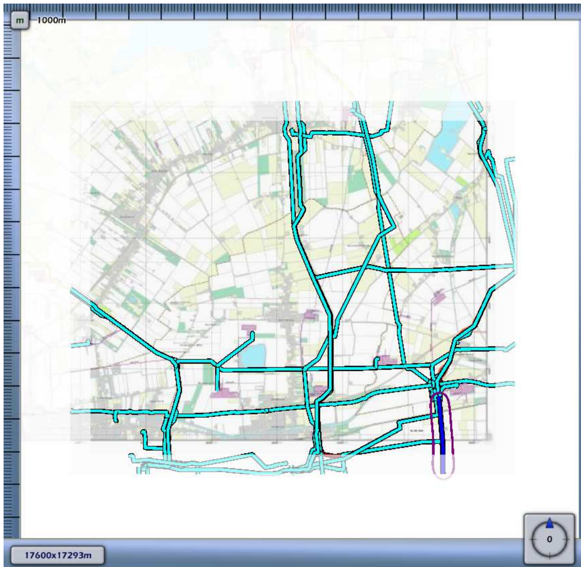
3.7 Figuur 3.7 Plaatsgebonden risico voor A-516 van N.V. Nederlandse Gasunie
