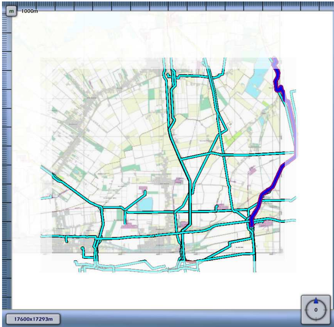
3.30 Figuur 3.30 Plaatsgebonden risico voor N-509-40 van N.V. Nederlandse Gasunie
