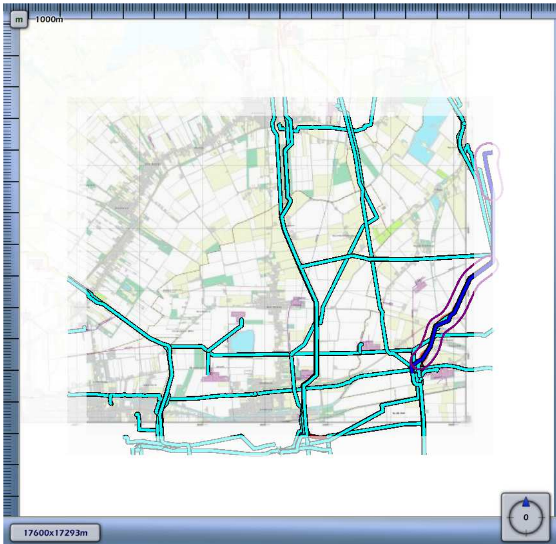
3.20 Figuur 3.20 Plaatsgebonden risico voor A-660 van N.V. Nederlandse Gasunie
