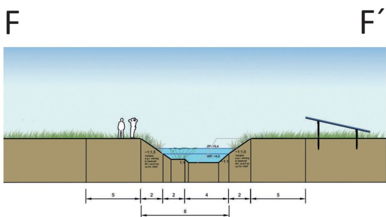
Profiel 5e wijk - noordrand 2e blok panelen.
