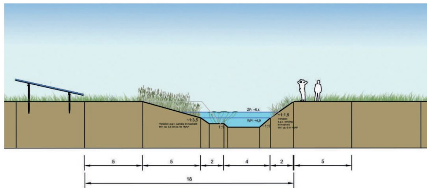
Profiel 6e wijk - zuidrand 2e blok panelen - brede oever
