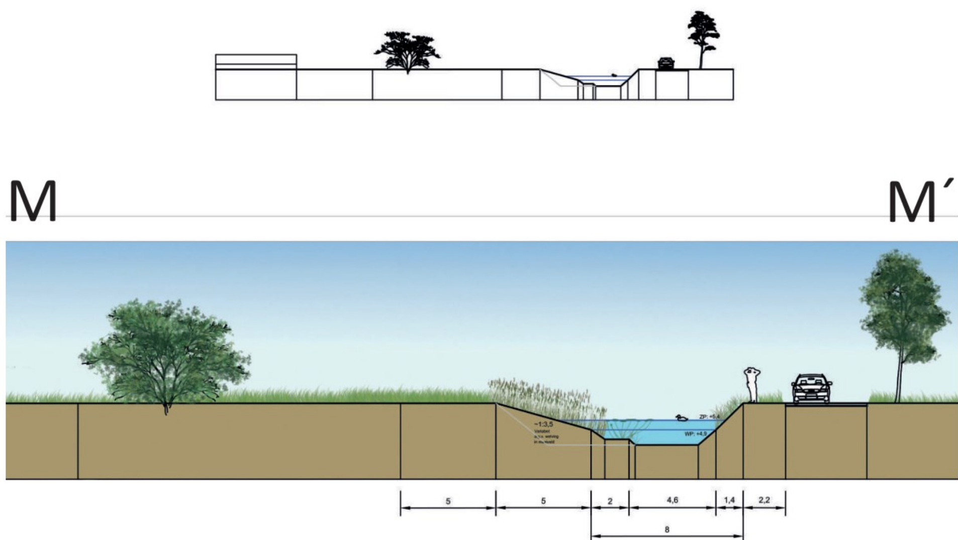
Profiel Zuiderkanaalweg noordelijke deel - brede watgang.
