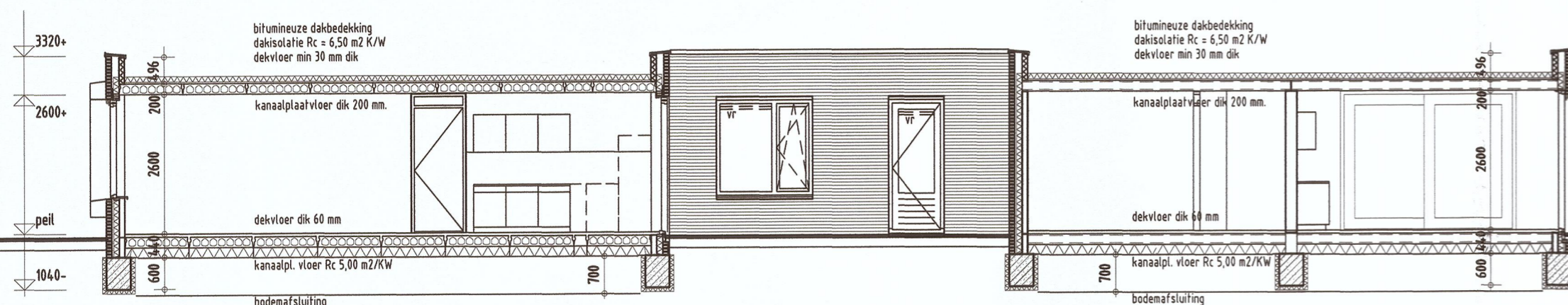
doorsnede A-A
