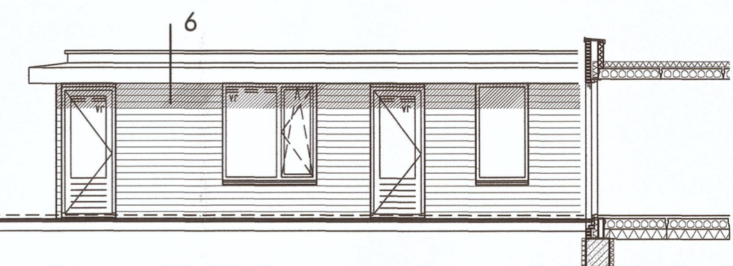
linker zijgevel woning - 1 noord-oostgevel
