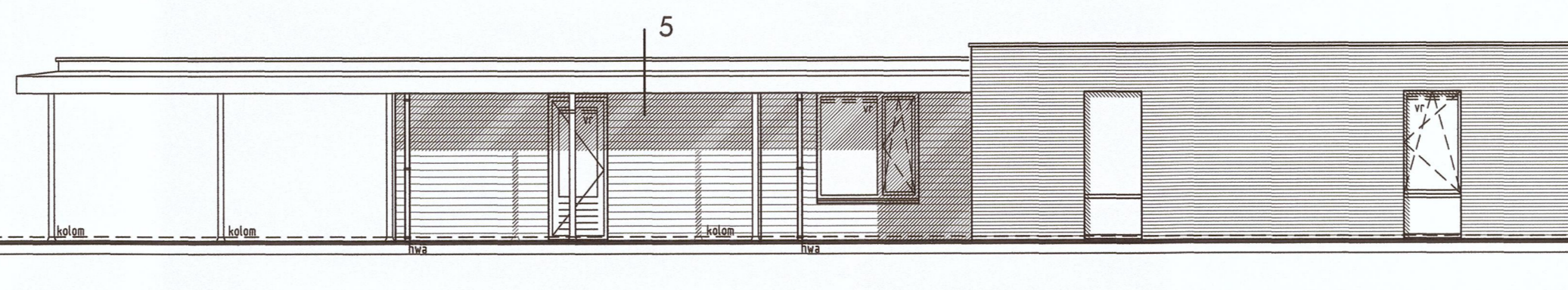
linker zijgevel woning - 2 noord-oostgevel
