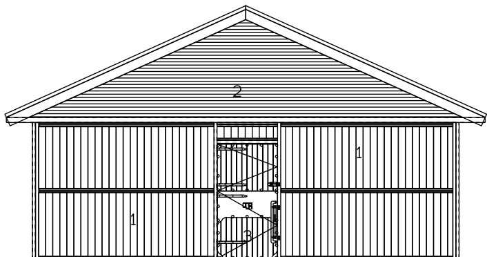
GEVEL A
