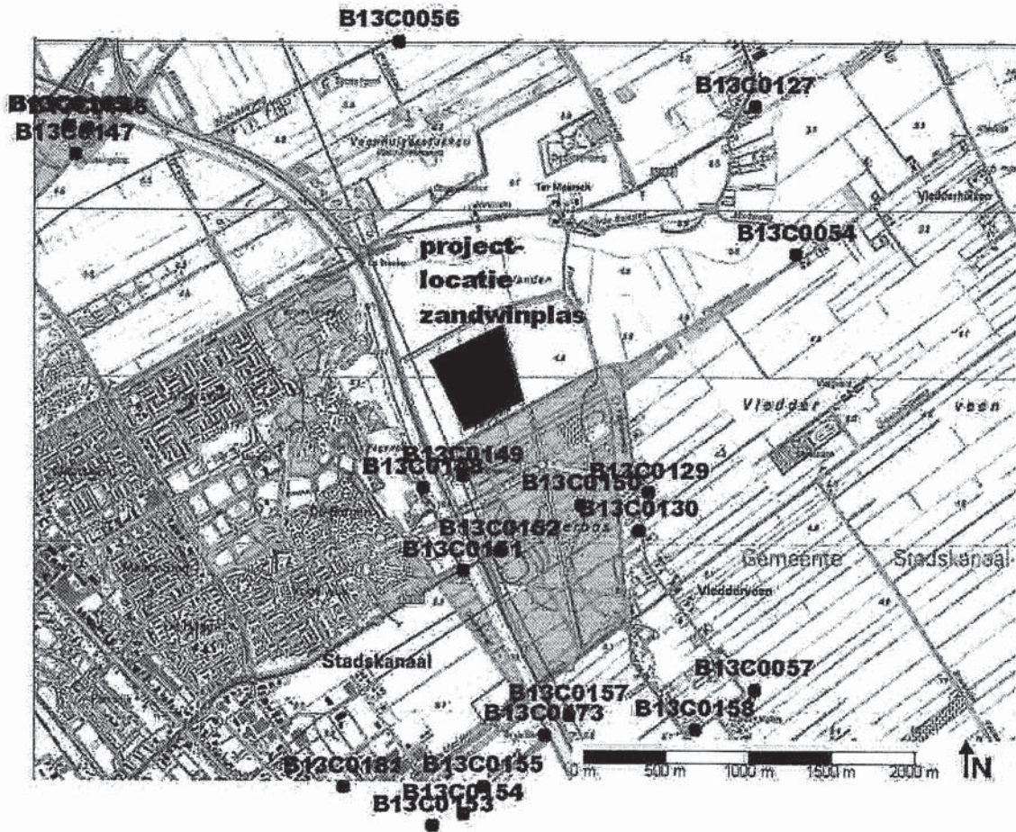
Figuur 1.1.1. Peilbuislocaties
