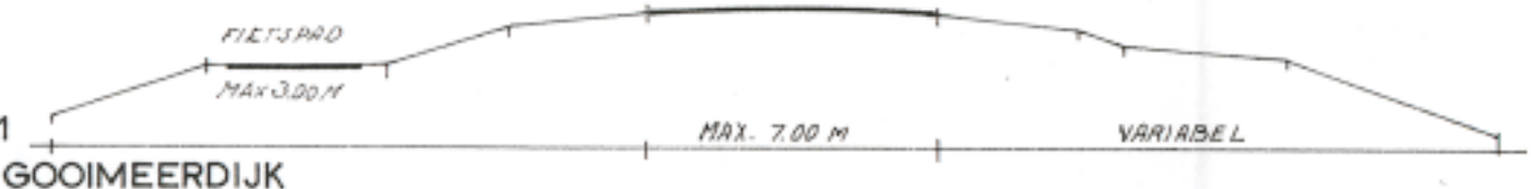
DWARSPROFIELEN 1 - 200
