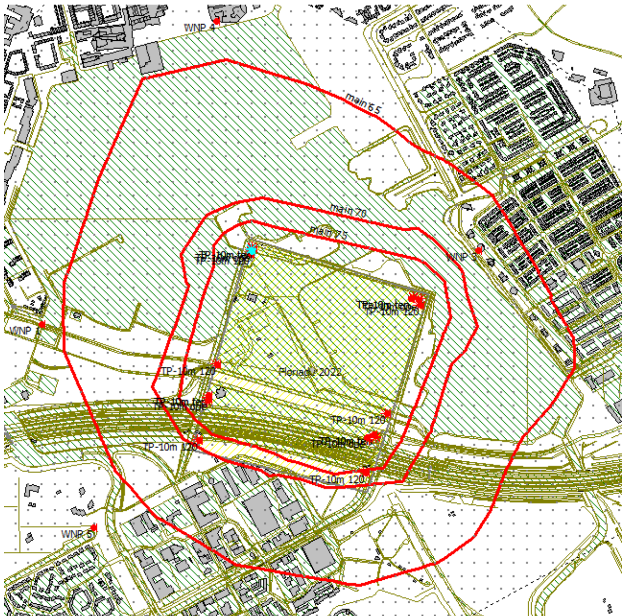
Figuur 2 – ligging 75, 70 en 65 dB(A) geluidscontour ten gevolge van een evenement met mainstage (open air)
