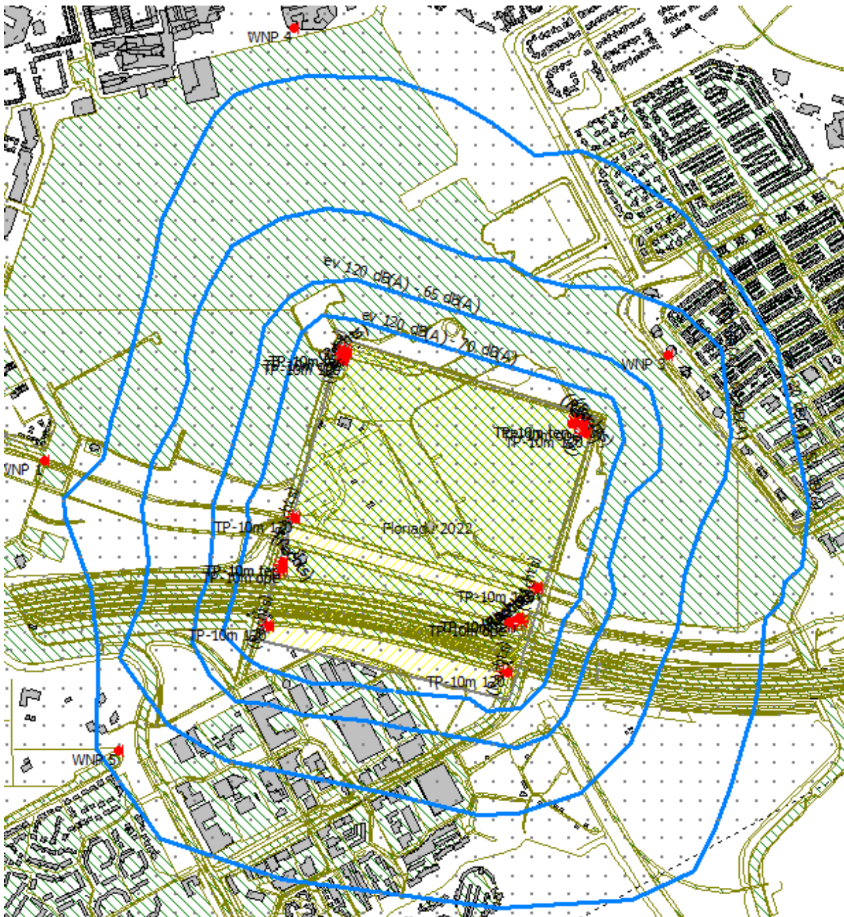
Figuur 1 – ligging 70, 65, 60 en 55 dB(A) geluidscontour ten gevolge van een niet geluidsdragend evenement
