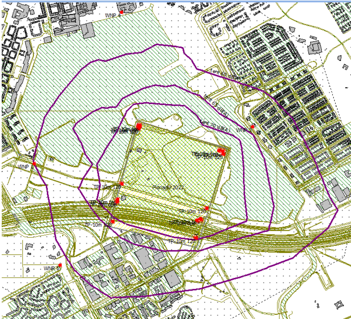
Figuur 3 – ligging 70, 65 en 60 dB(A) geluidscontour ten gevolge van een evenement met een tent (groot en gerichte uitstraling)
