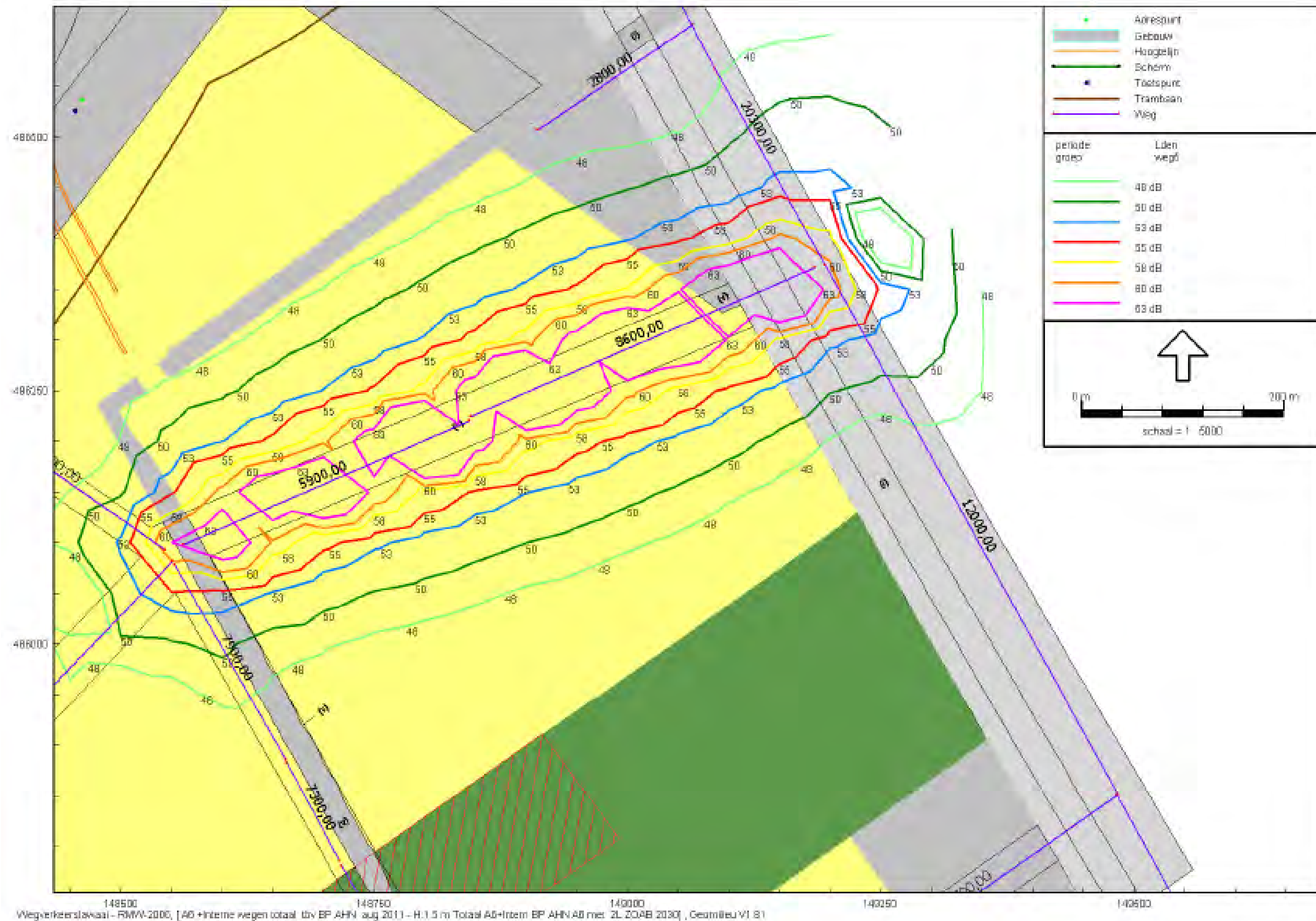
Figuur 5a: weg 5/1.5 m hoogte
