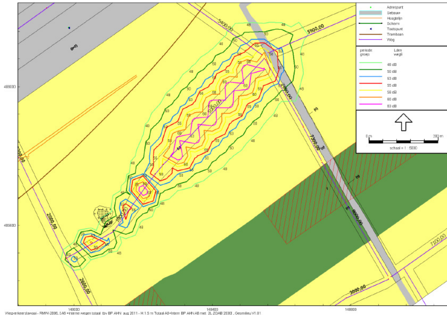
Figuur 9a: weg 9/1.5 m hoogte
