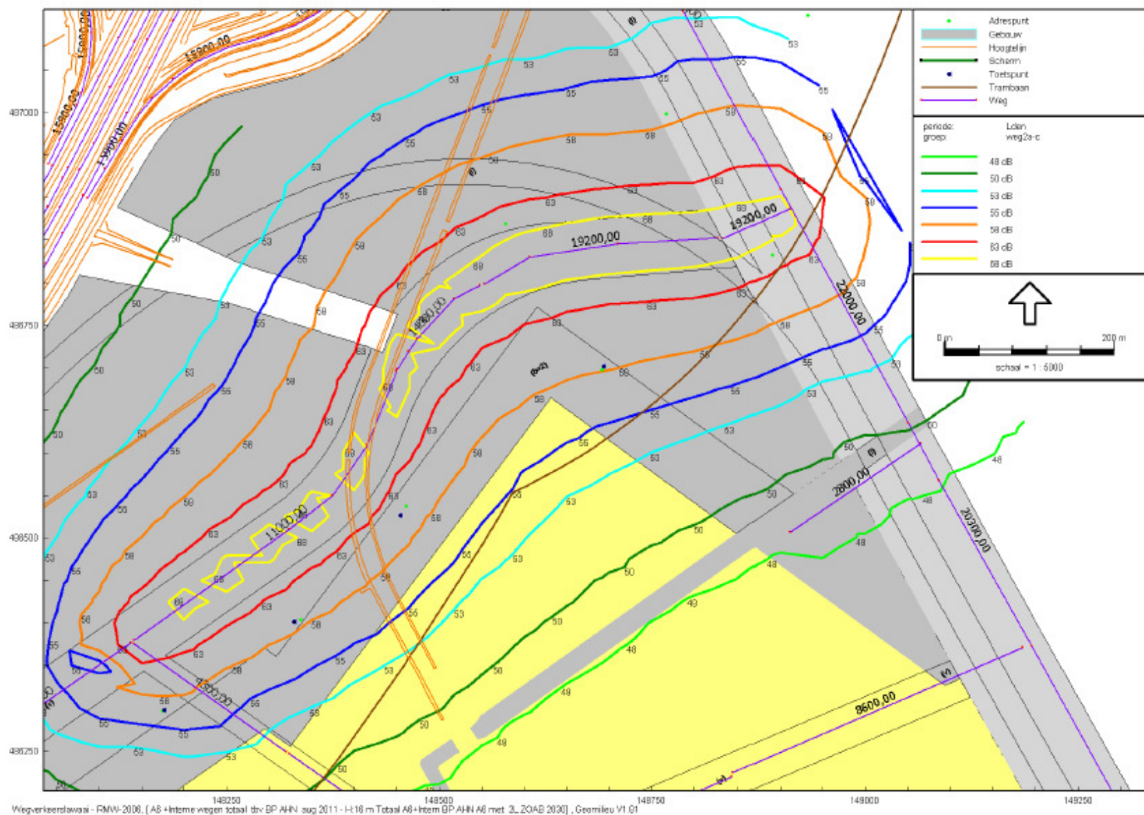
Figuur 2b: weg 2/16 m hoogte
