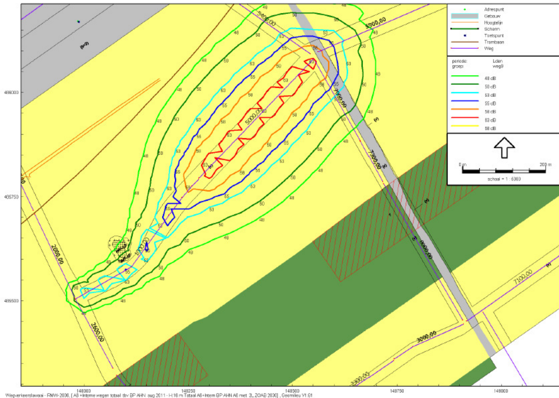
Figuur 9b: weg 9/16 m hoogte
