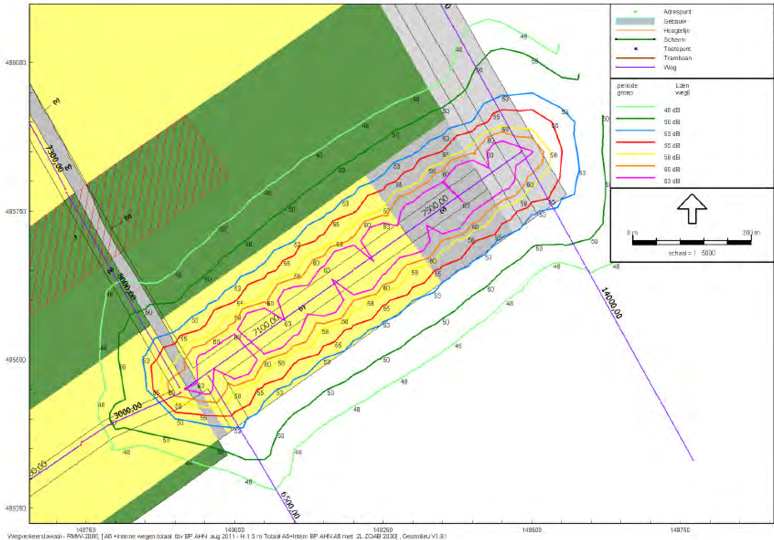
Figuur 6a: weg 6/1.5 m hoogte
