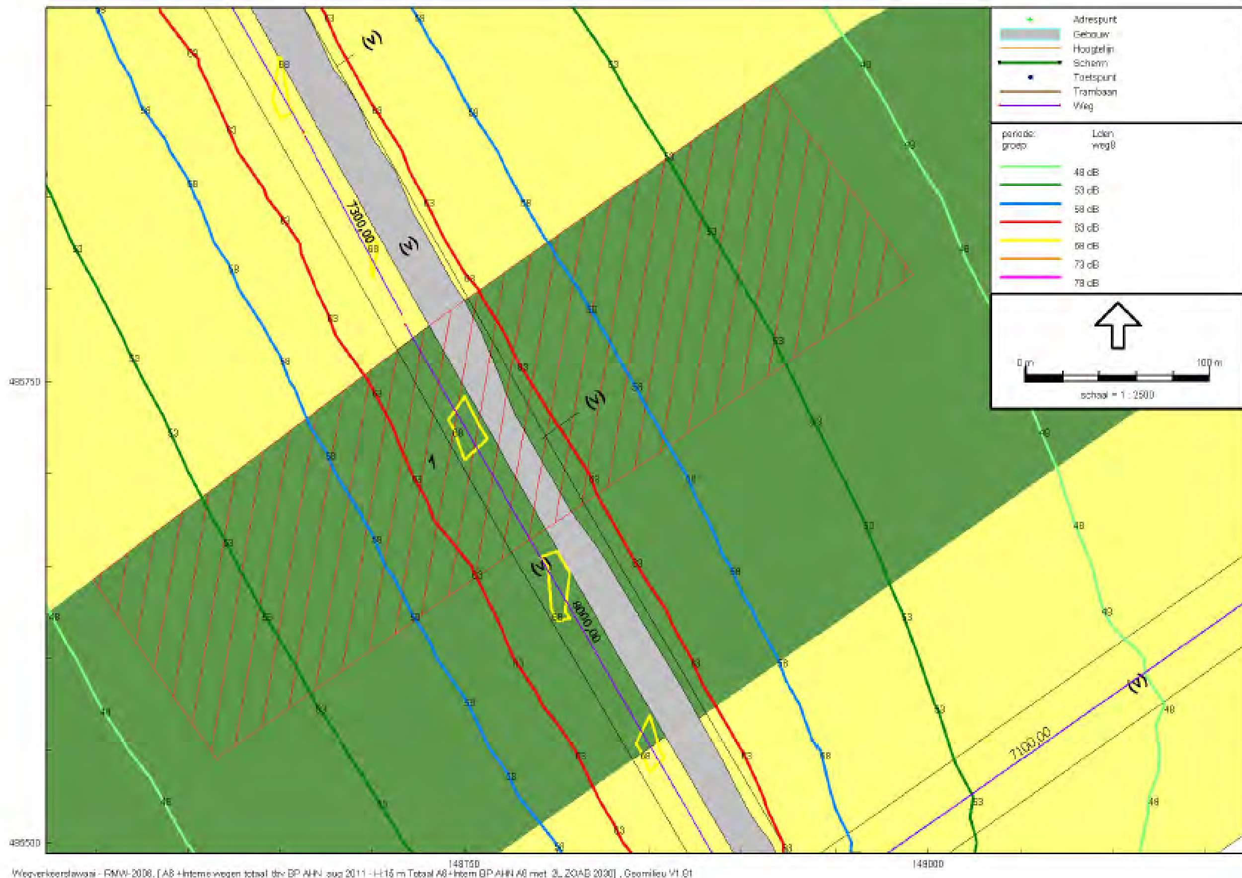
Figuur 8b: weg 8/15 m hoogte
