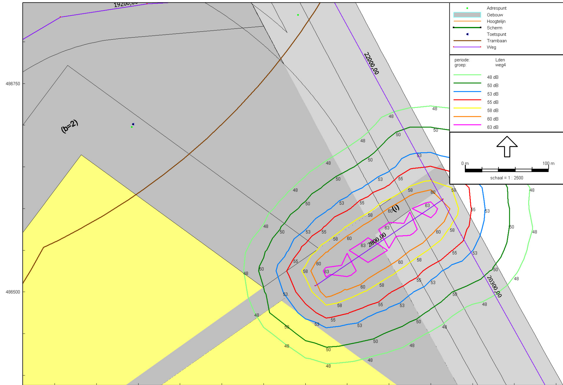
Figuur 4b: weg 4/12 m hoogte
