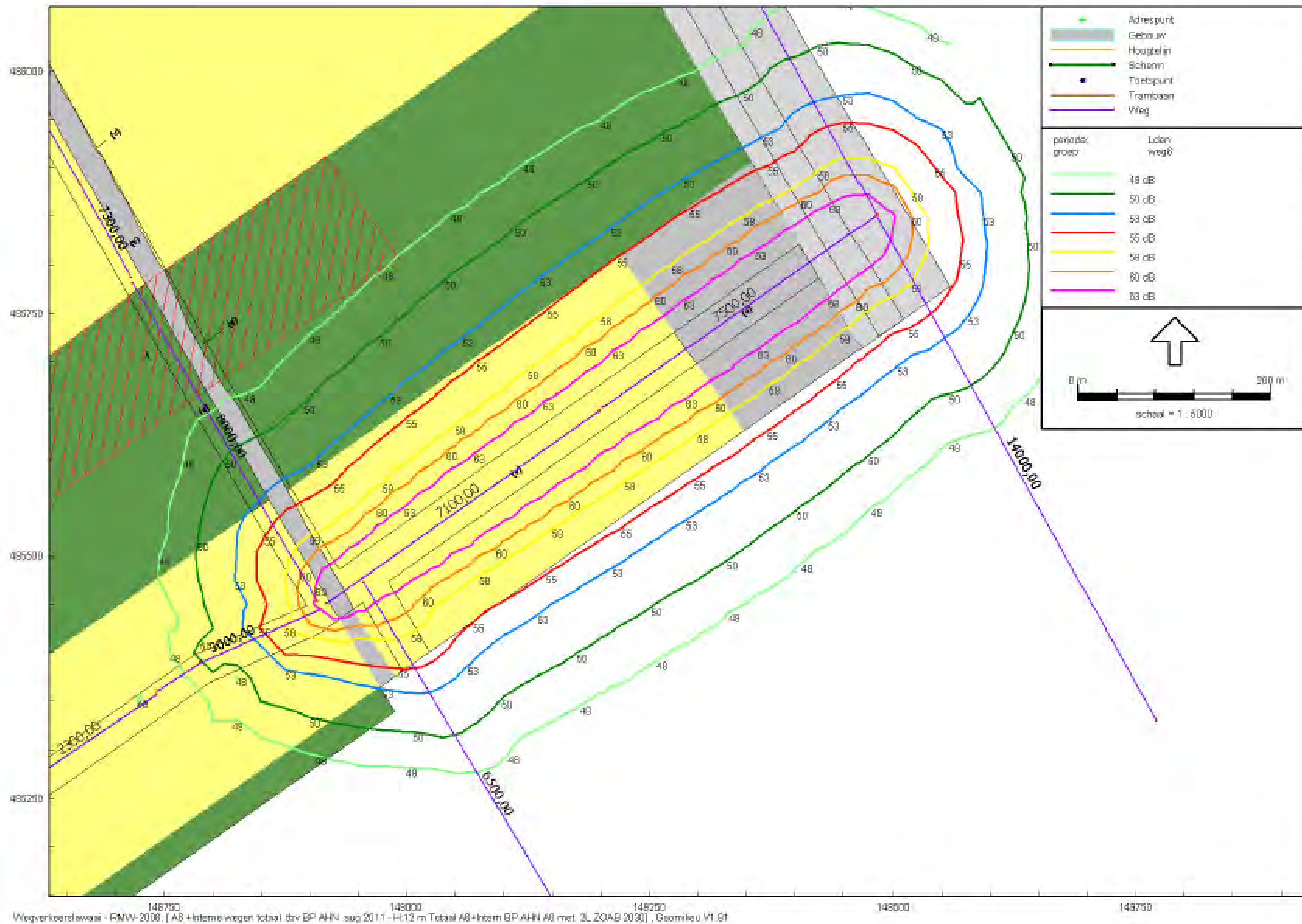
Figuur 6b: weg 6/12 m hoogte
