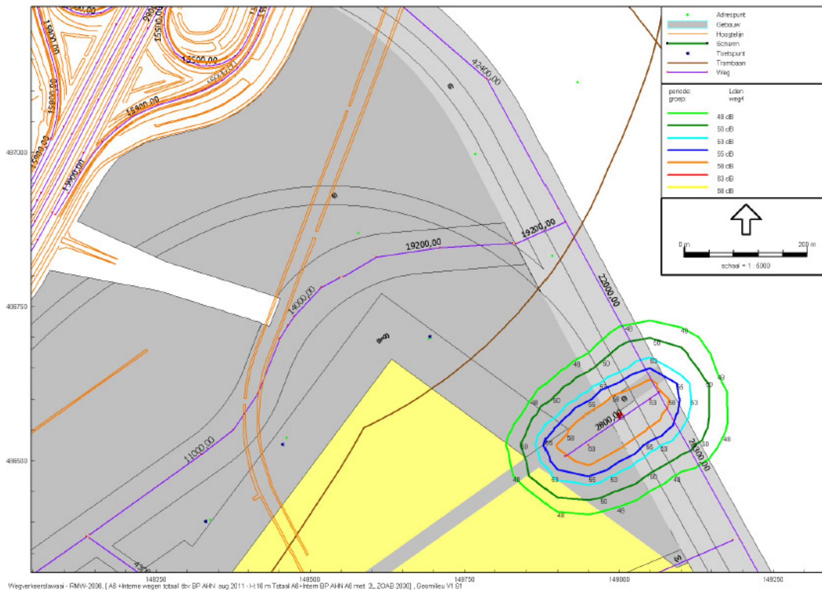
Figuur 4c: weg 4/16 m hoogte
