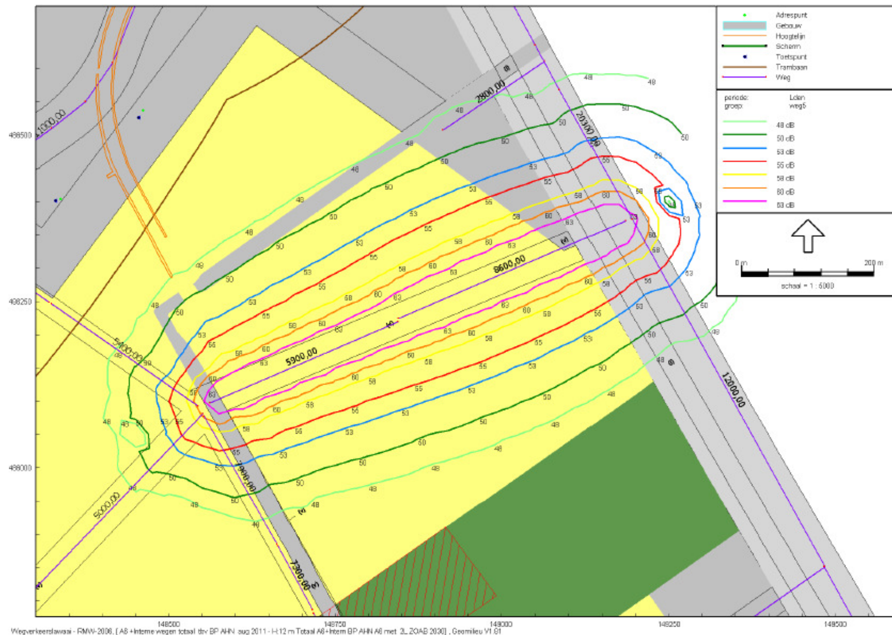
Figuur 5b: weg 5/12 m hoogte
