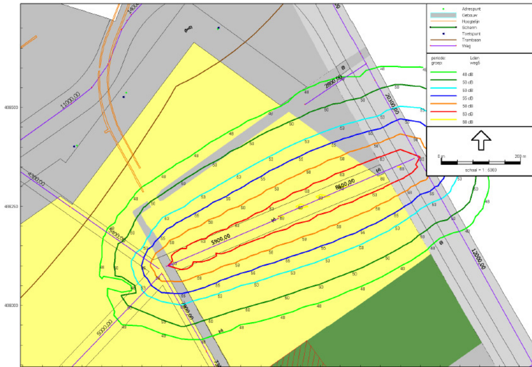
Figuur 5c: weg 5/16 m hoogte
