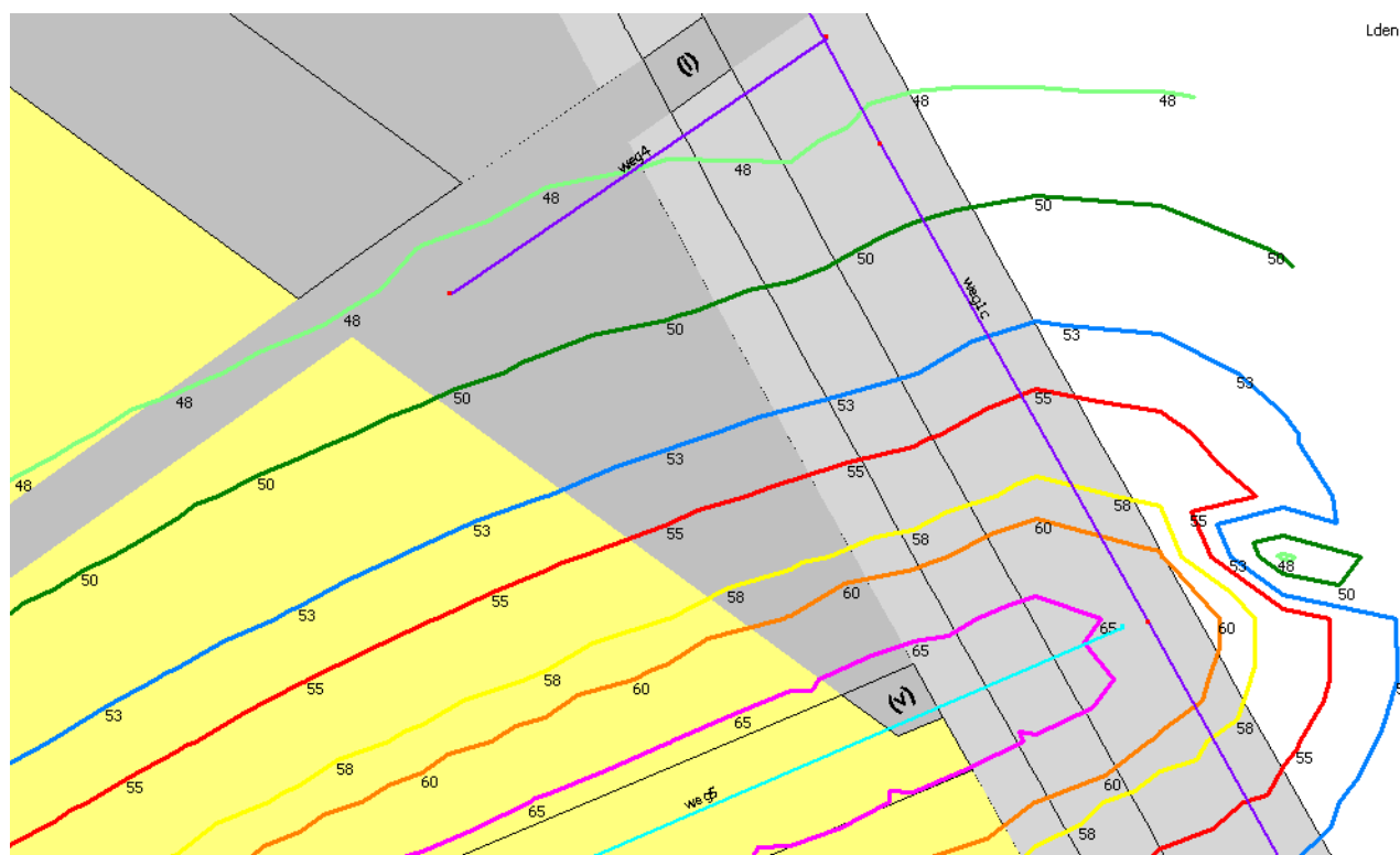
Figuur 3-9: 12 m excl. 5 dB aftrek (zie ook bijlage 13)
