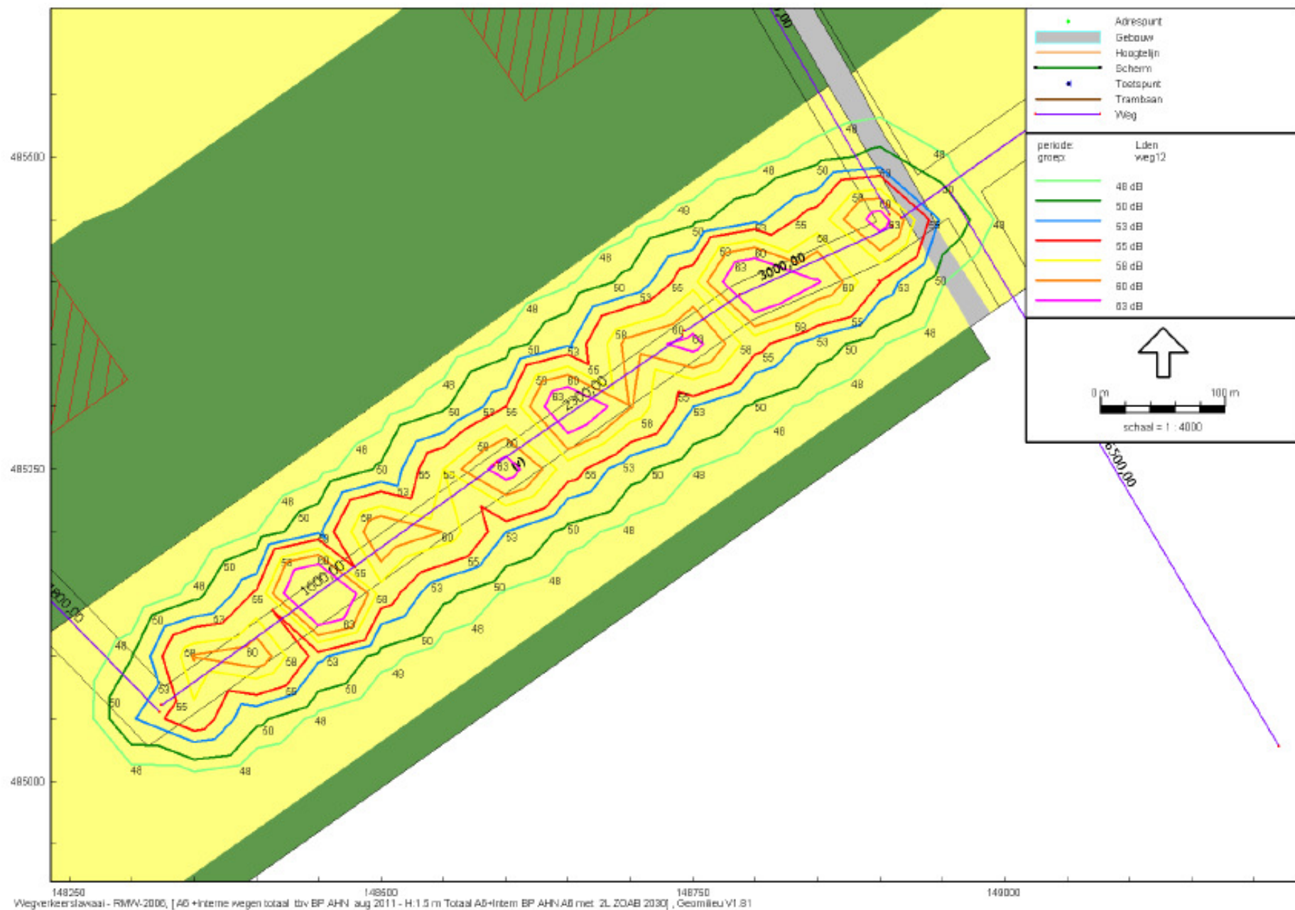
Figuur 12a: weg 12/1.5 m hoogte
