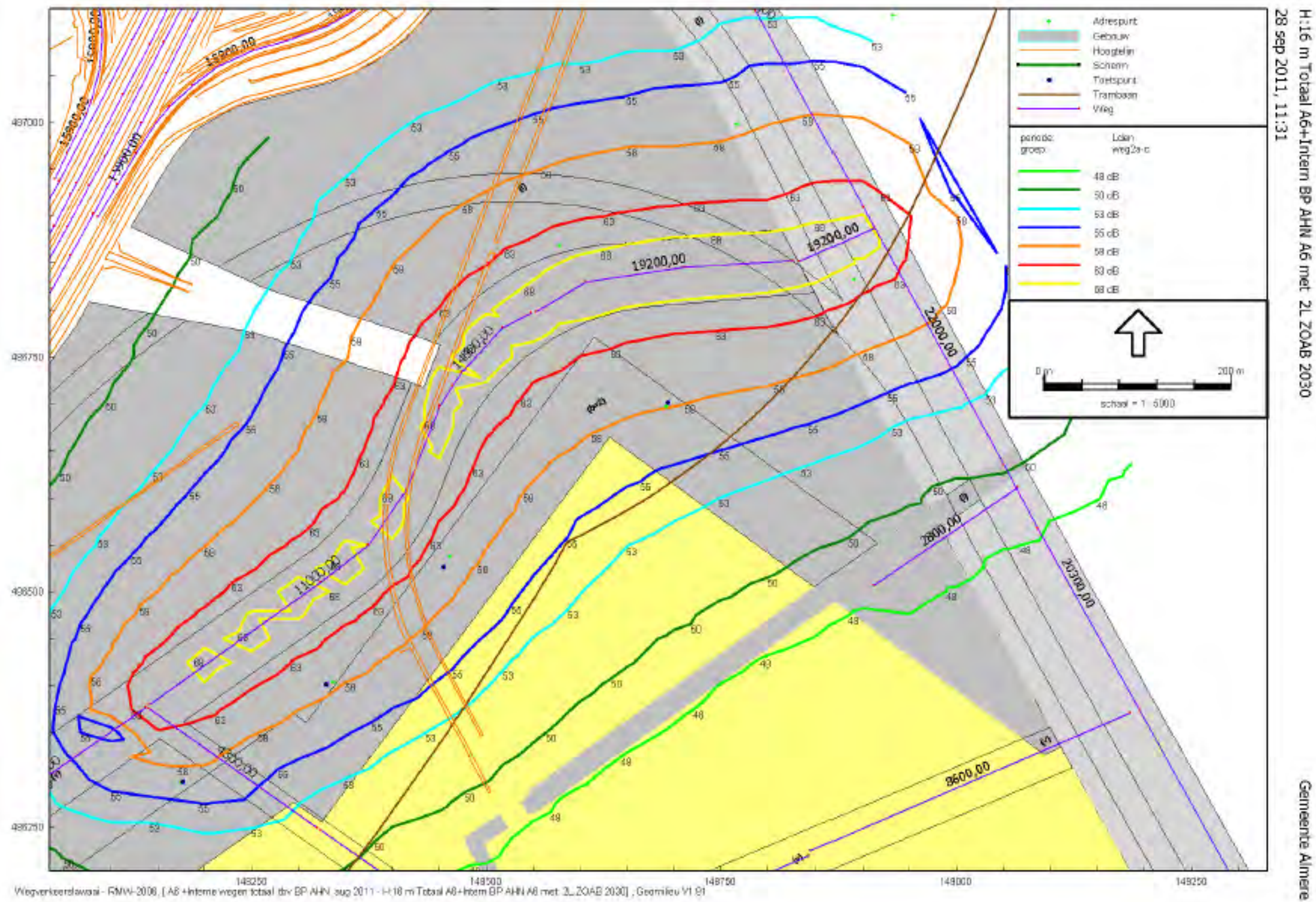
Figuur 2b: weg 2/16 m hoogte
