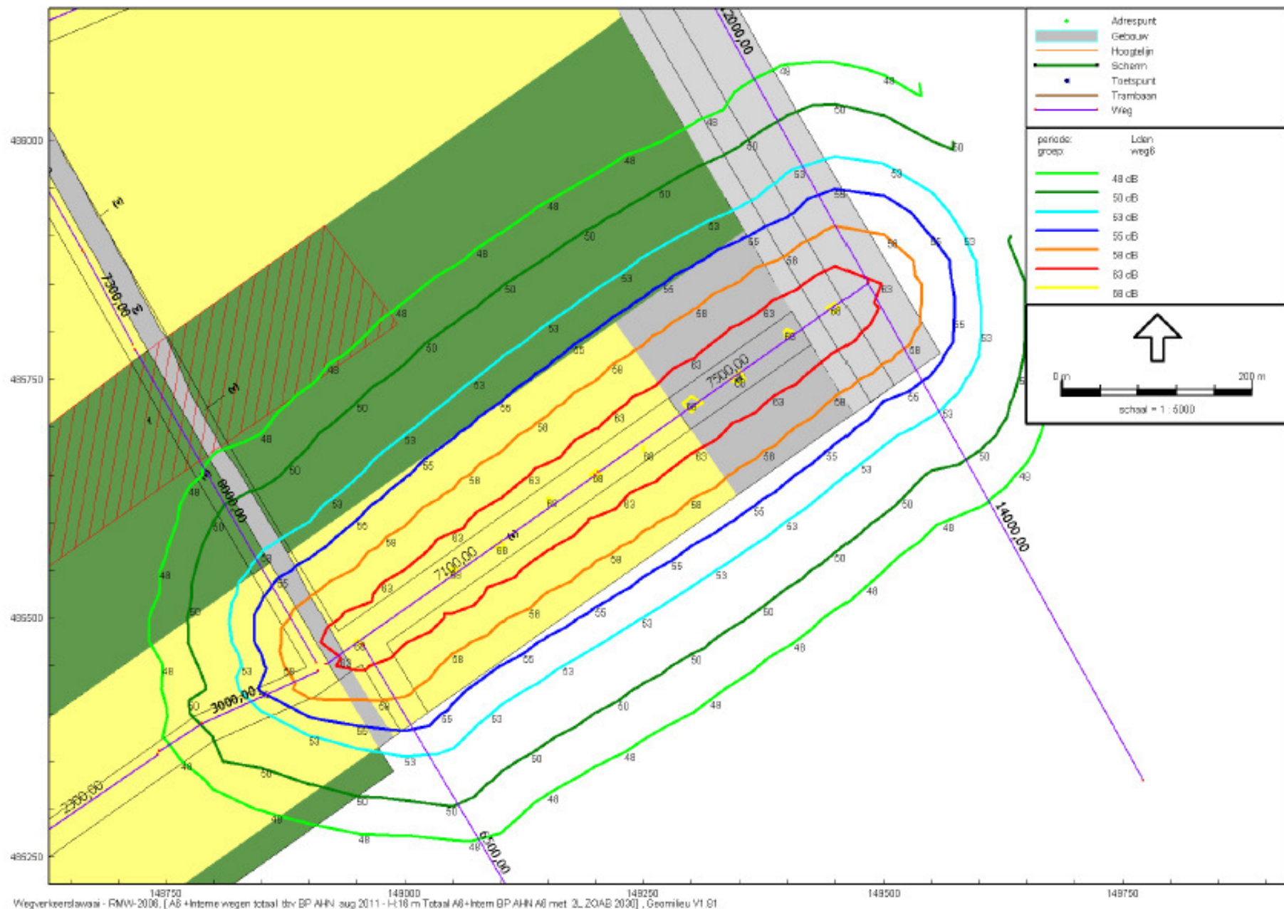
Figuur 6c: weg 6/16 m hoogte
