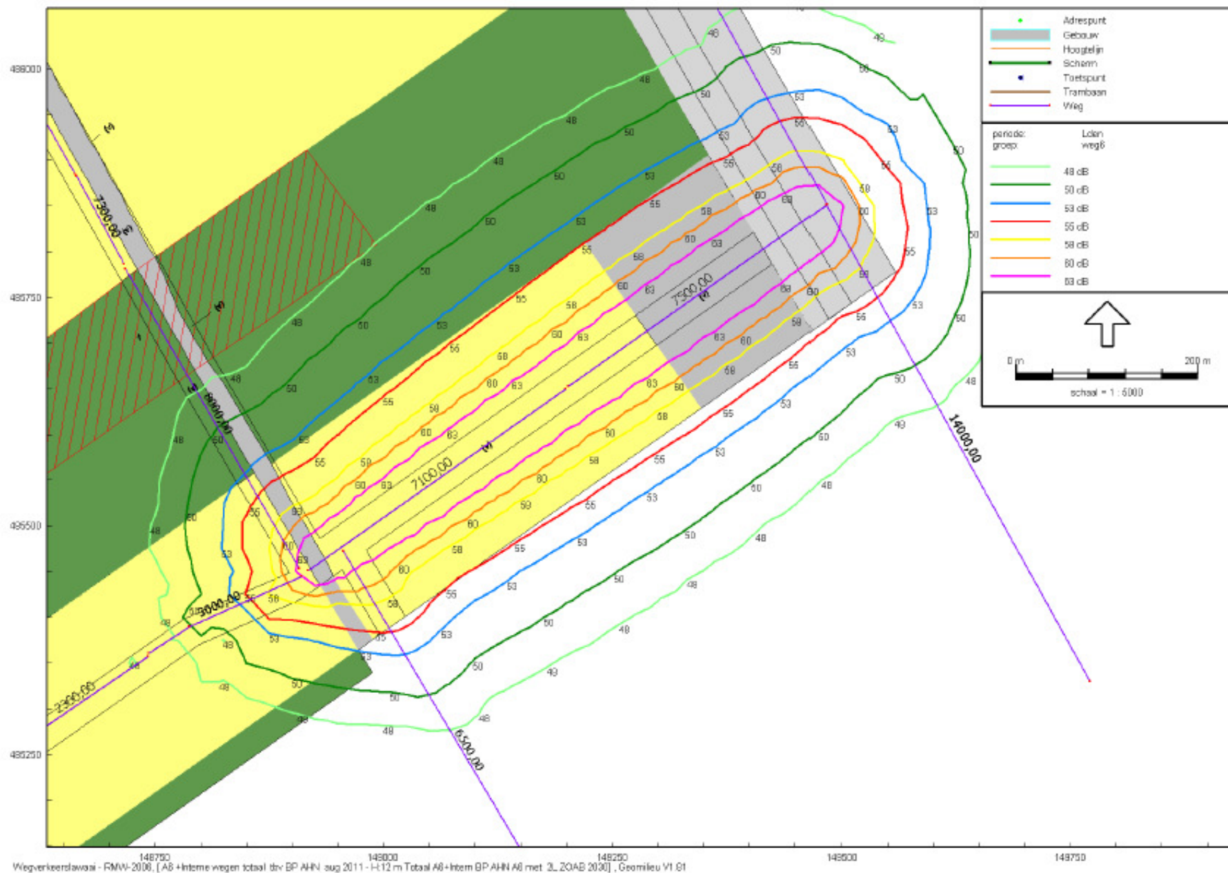
Figuur 6b: weg 6/12 m hoogte
