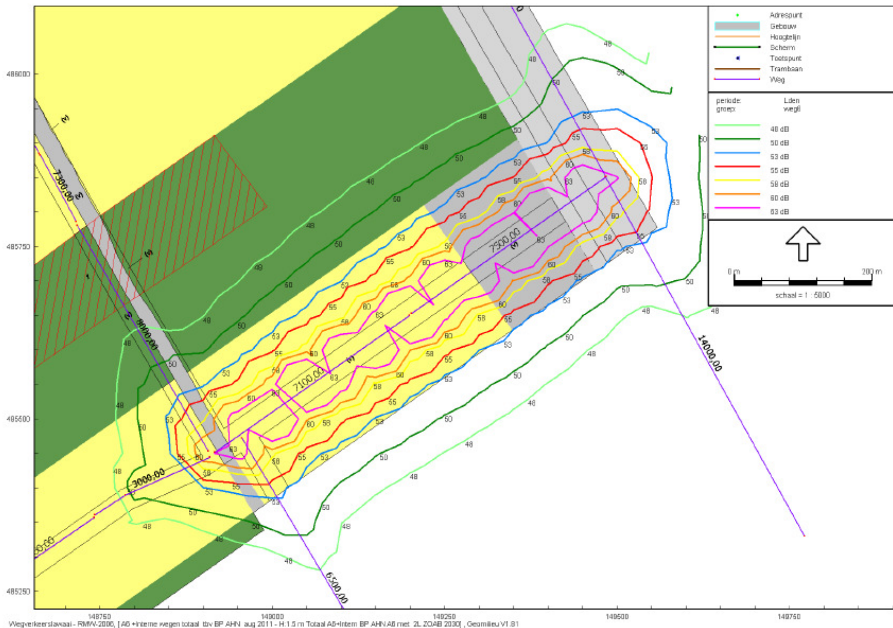
Figuur 6a: weg 6/1.5 m hoogte
