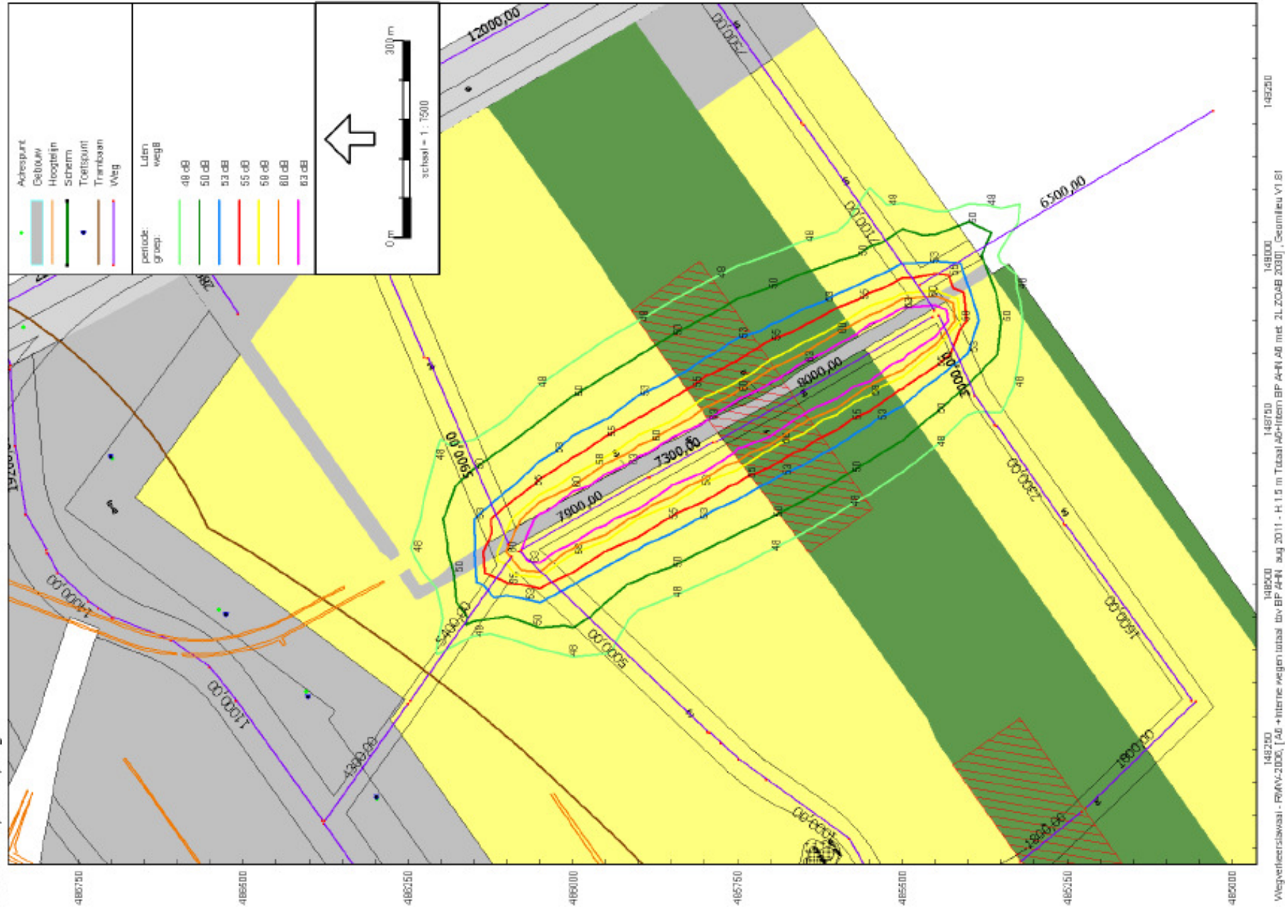
H:1.5 m Totaal A6+Intern BP AHN A6 met 2L ZOAB 2030 3 okt 2011, 09:27/weg 8
