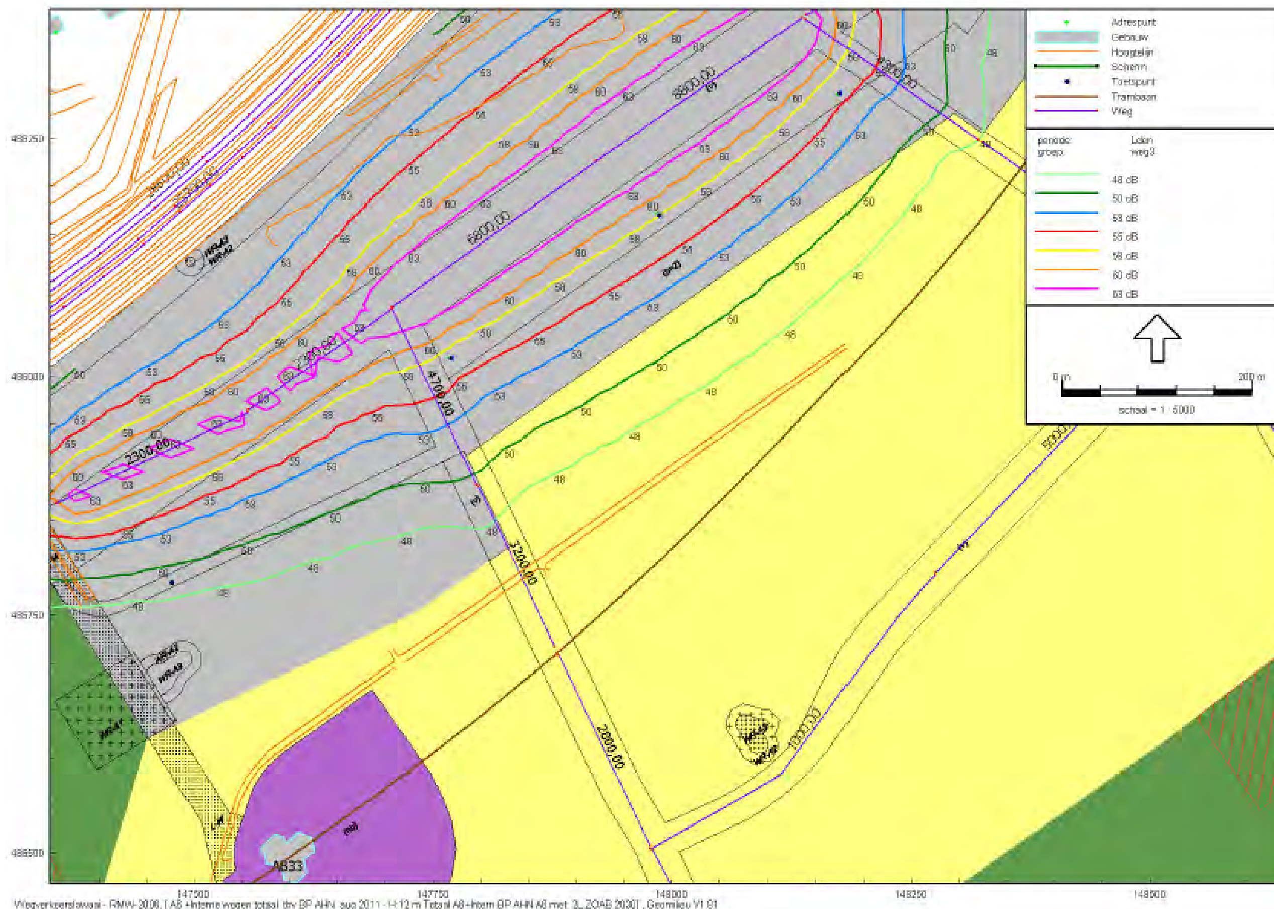
Figuur 3b: weg 3/12 m hoogte
