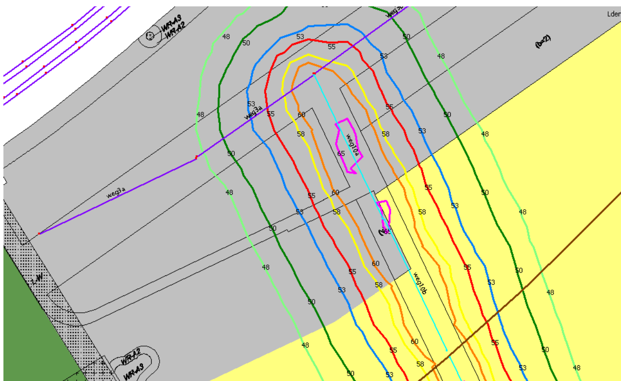
Figuur 3-6: Invloed interne wegen, 12 m excl. aftrek 5 dB (zie ook bijlage 13)
