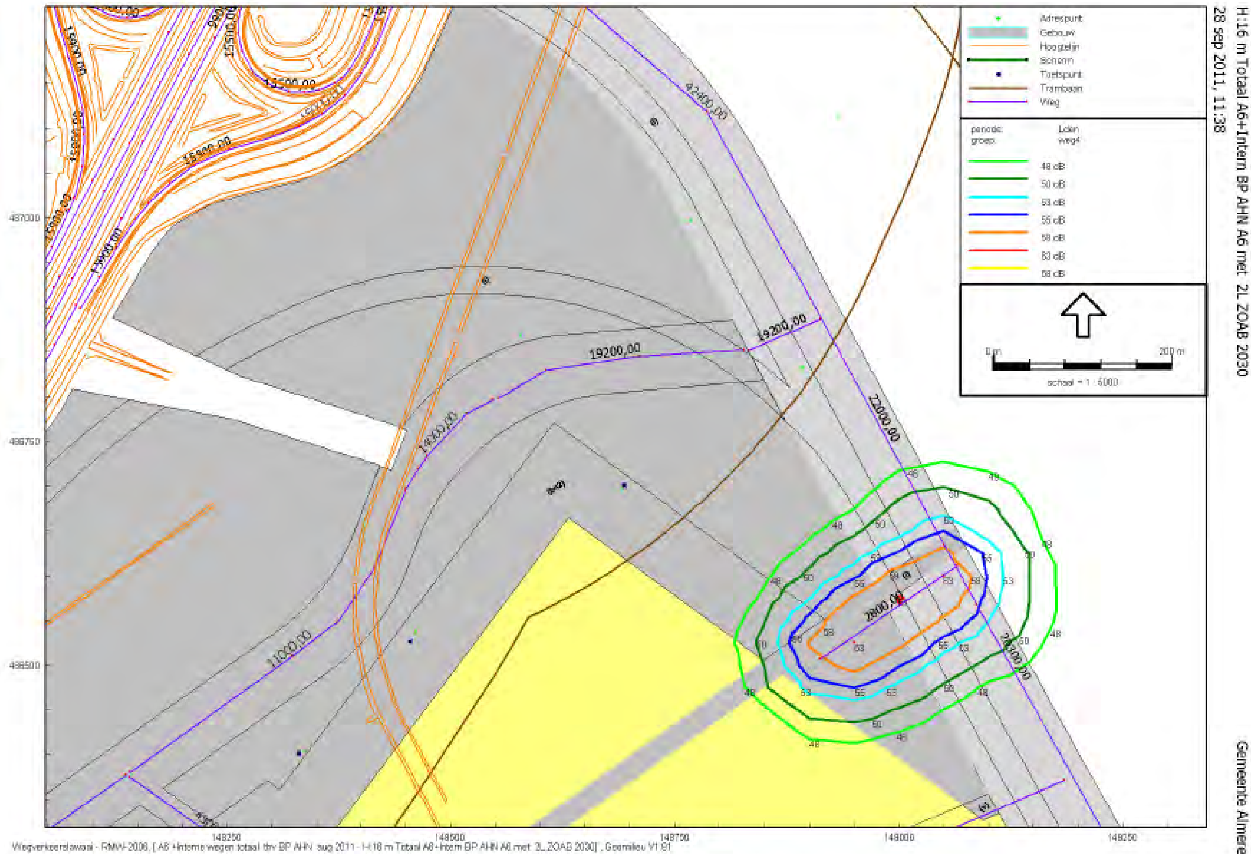
Figuur 4c: weg 4/16 m hoogte
