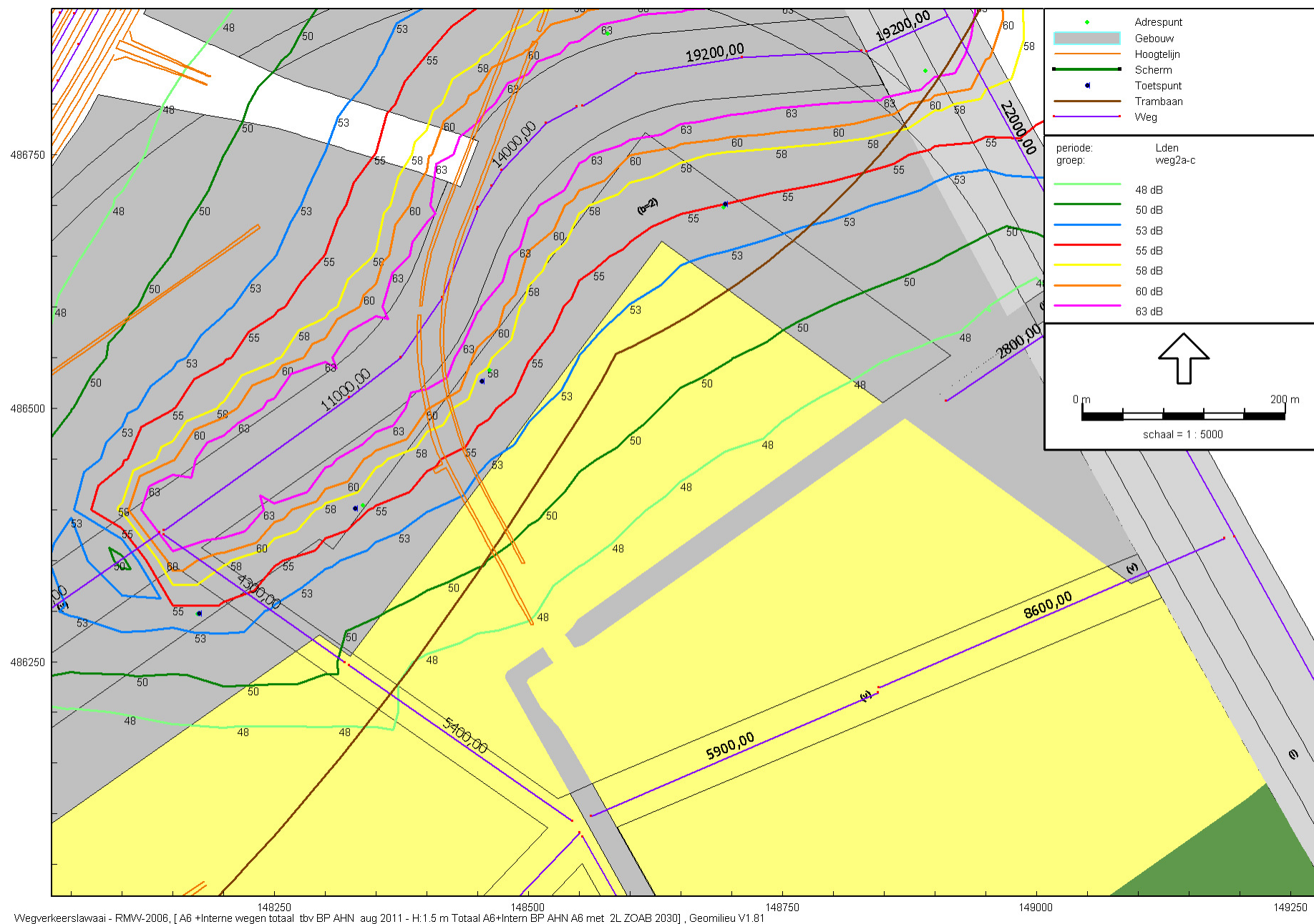
Figuur 2a: weg 2/1.5 m hoogte
