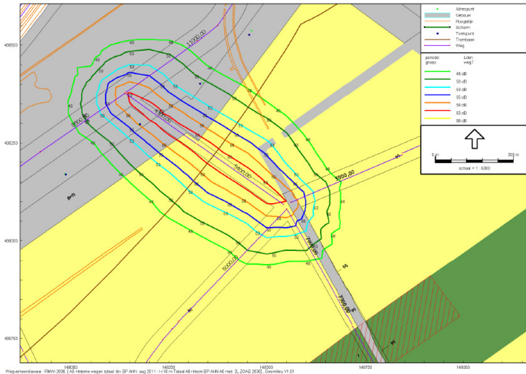
Figuur 7c: weg 7/16 m hoogte
