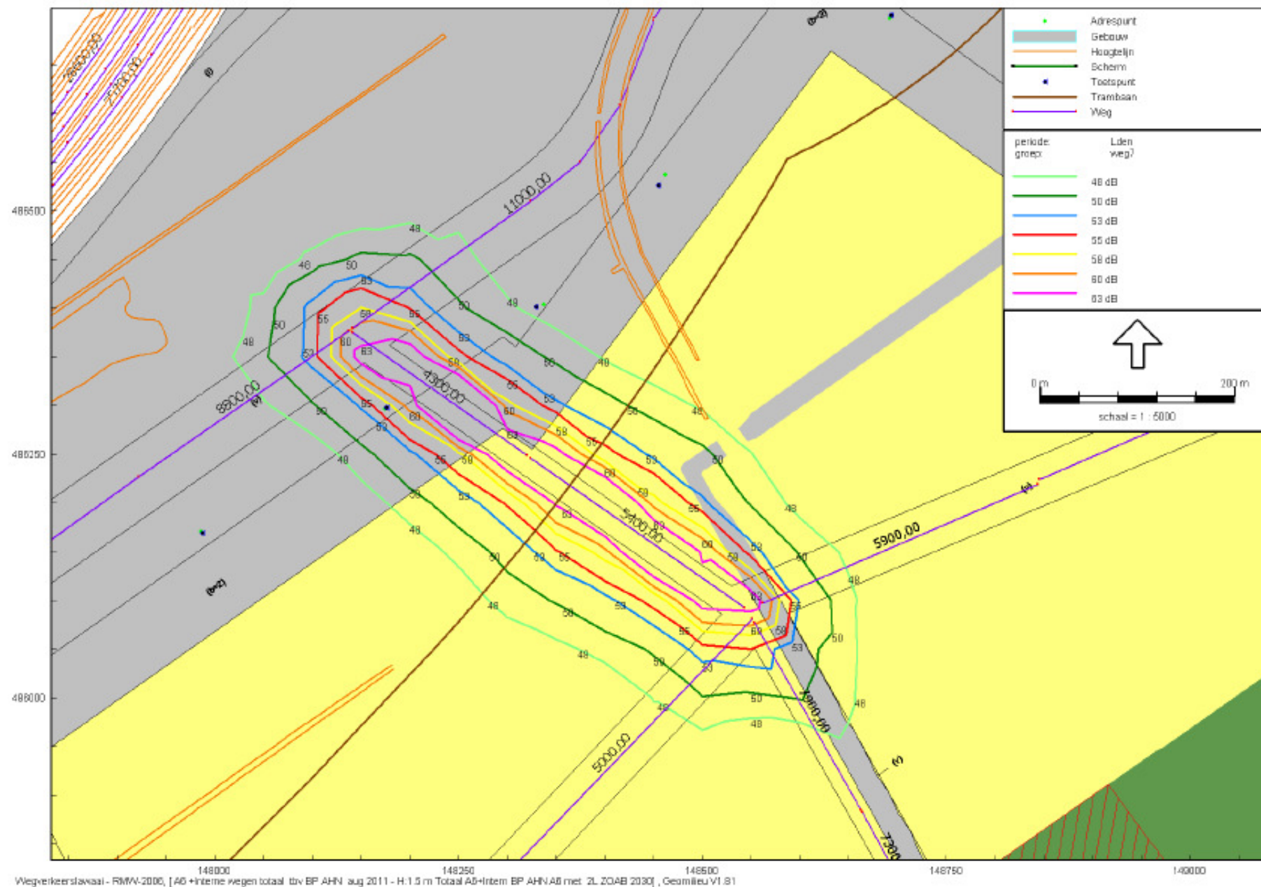
Figuur 7a: weg 7/1.5 m hoogte
