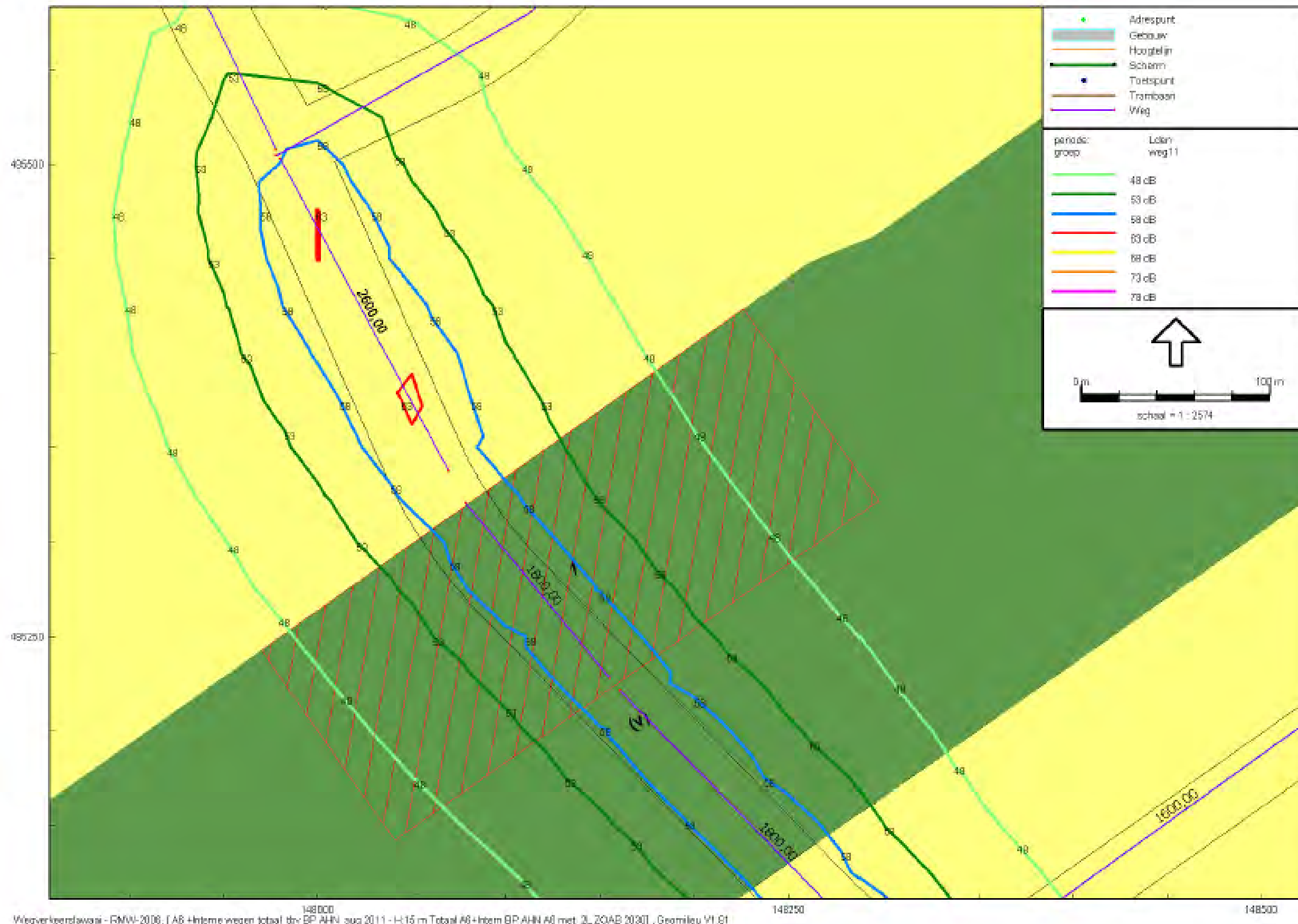
Figuur 11b: weg 11/15 m hoogte
