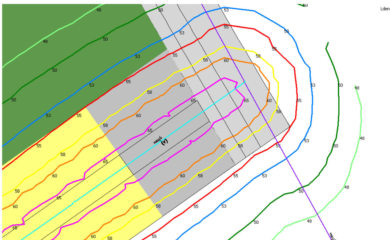
Figuur 3-11: 12 m excl. 5 dB aftrek (zie ook bijlage 13)
