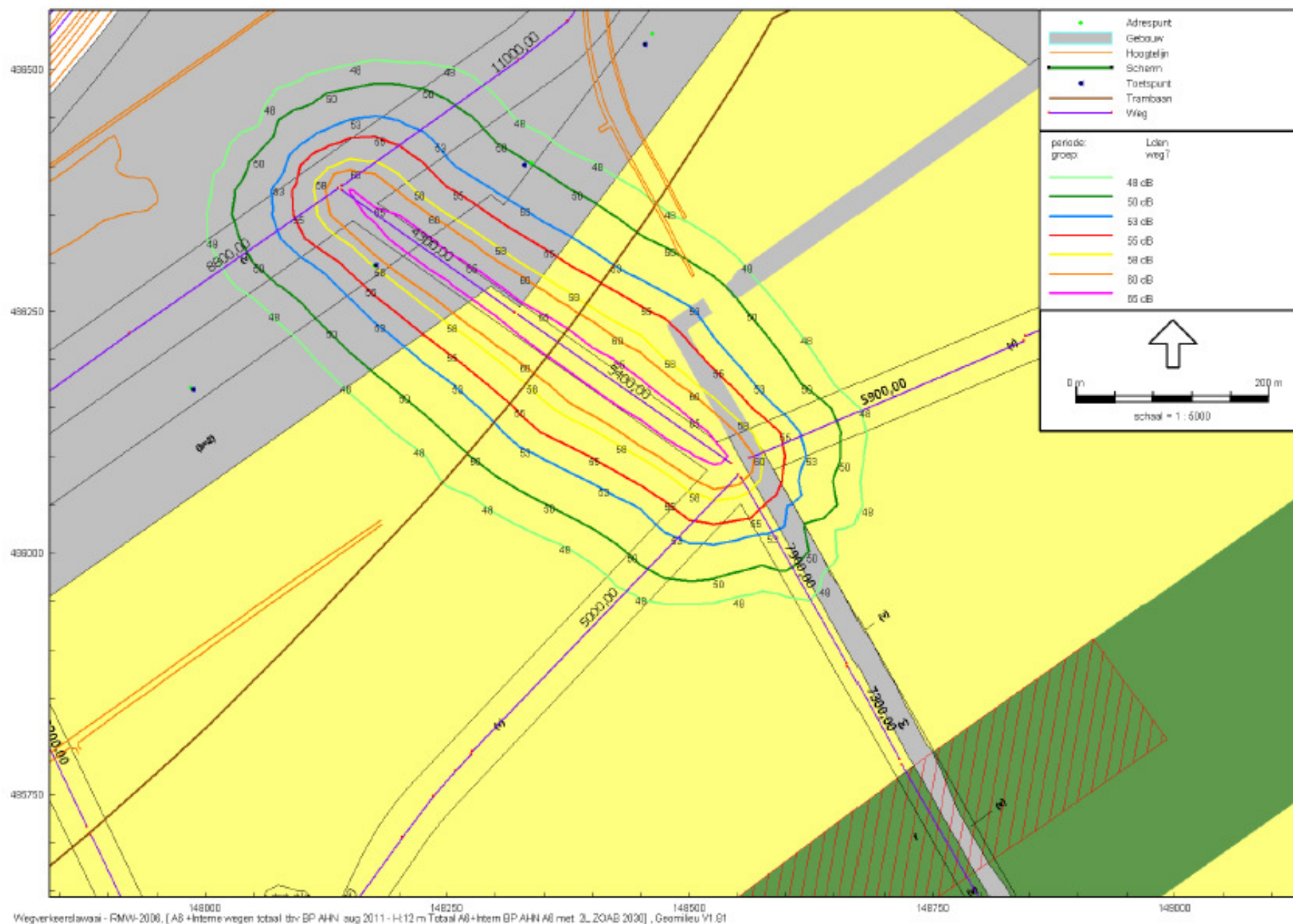
Figuur 7b: weg 7/12 m hoogte
