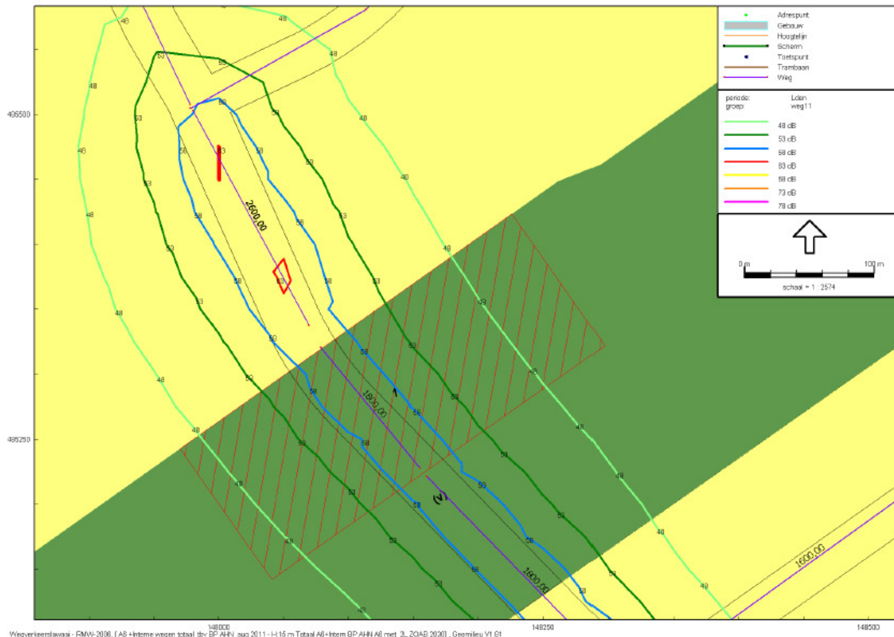
Figuur 11b: weg 11/15 m hoogte
