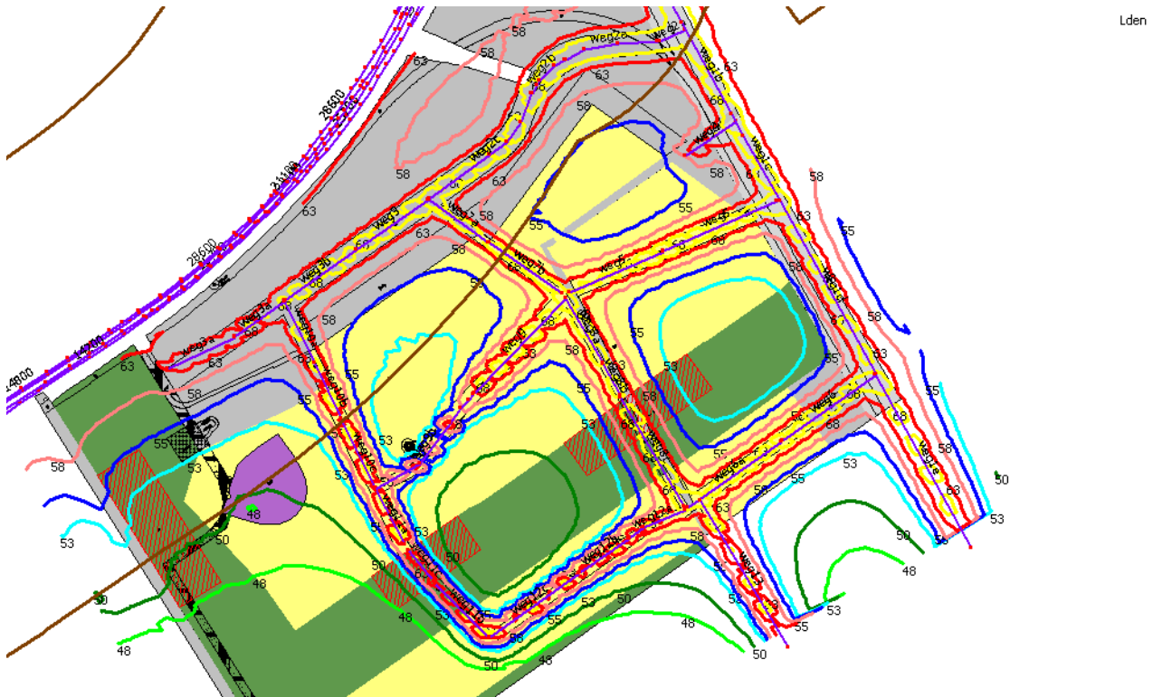
Figuur 3–12: GES 1.5 m excl. aftrek
