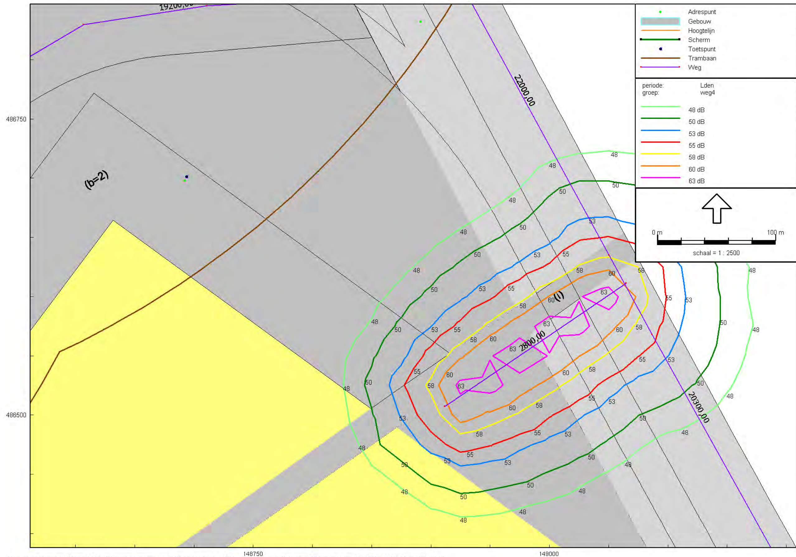
Figuur 4b: weg 4/12 m hoogte
