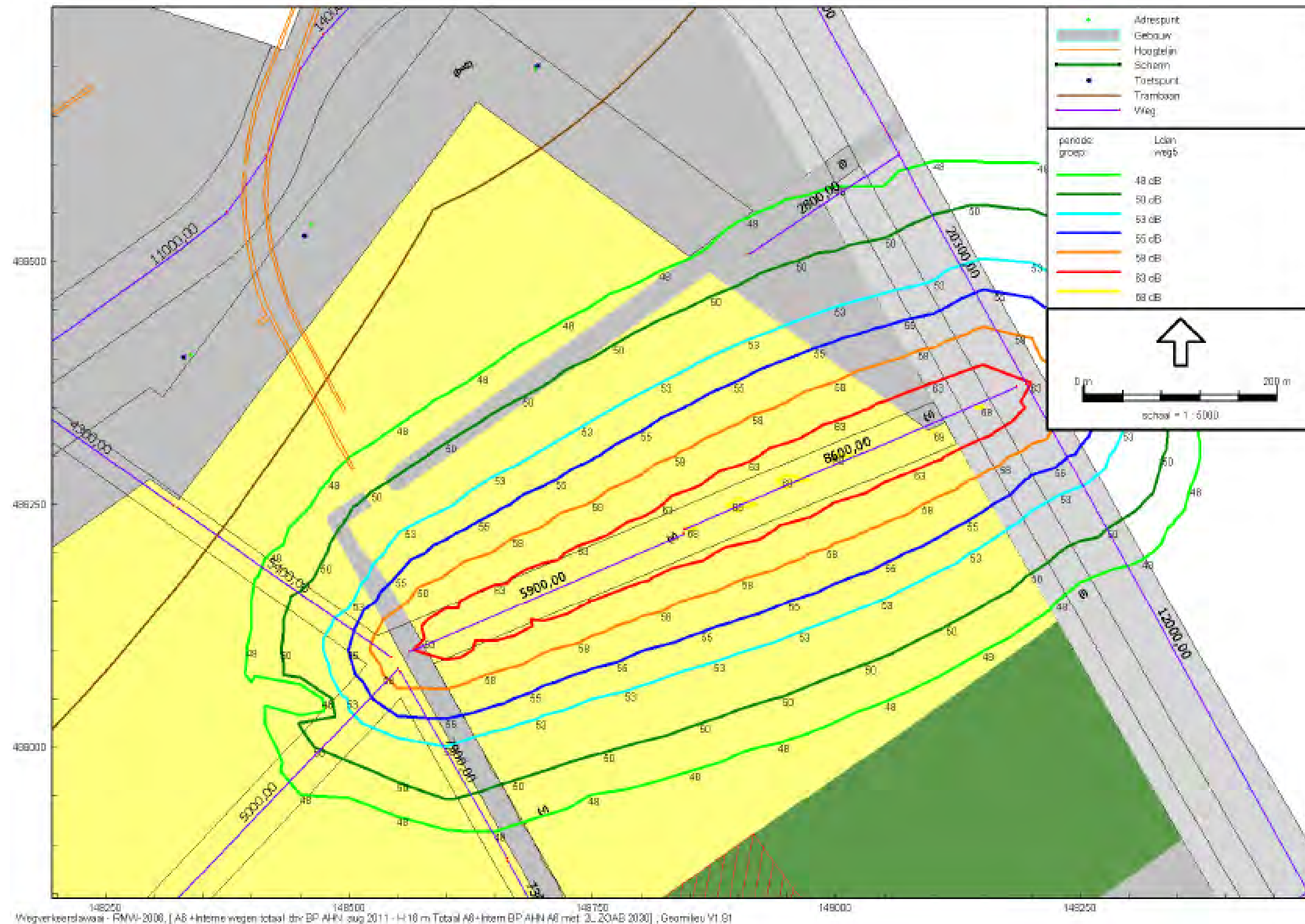
Figuur 5c: weg 5/16 m hoogte
