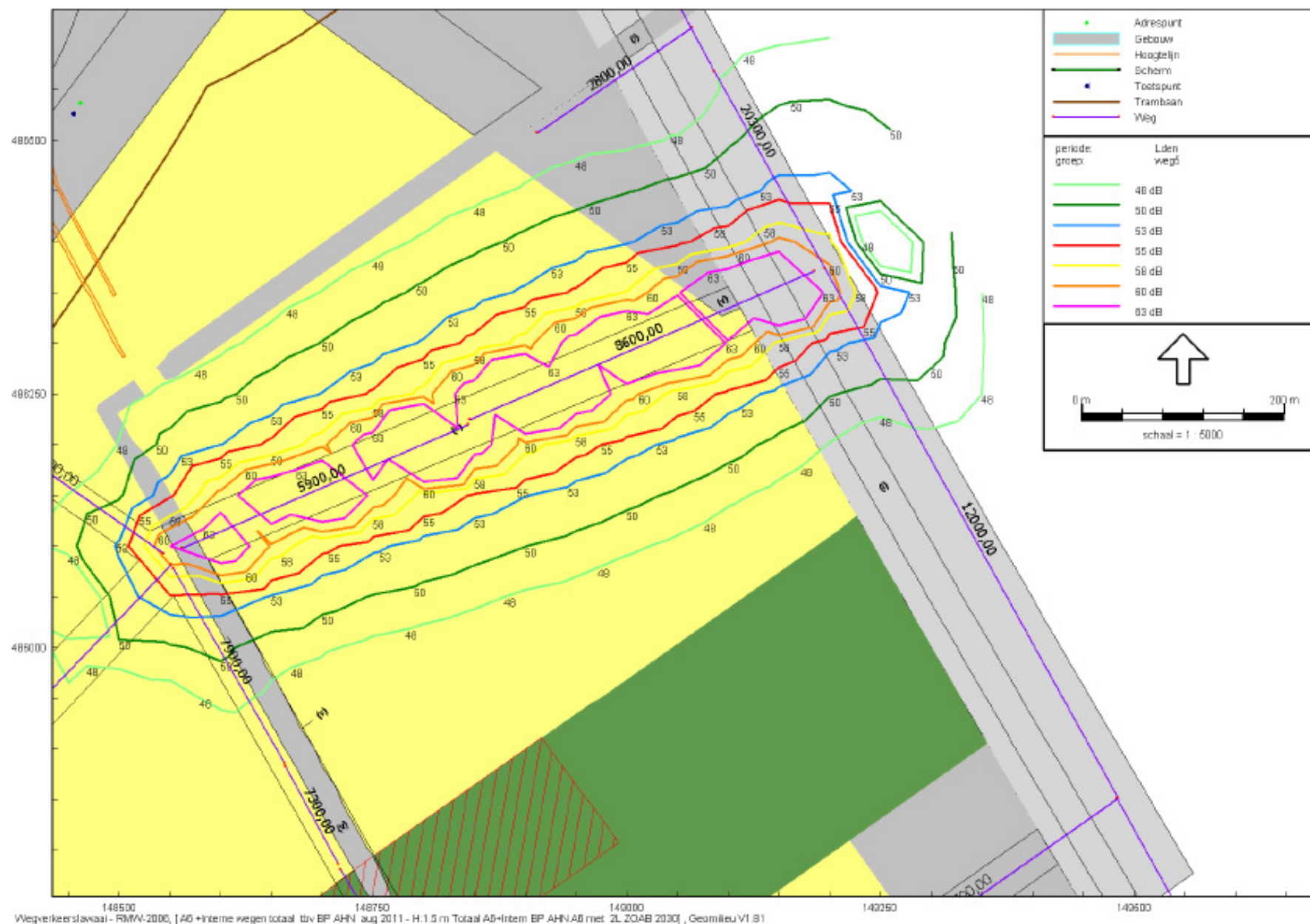
Figuur 5a: weg 5/1.5 m hoogte
