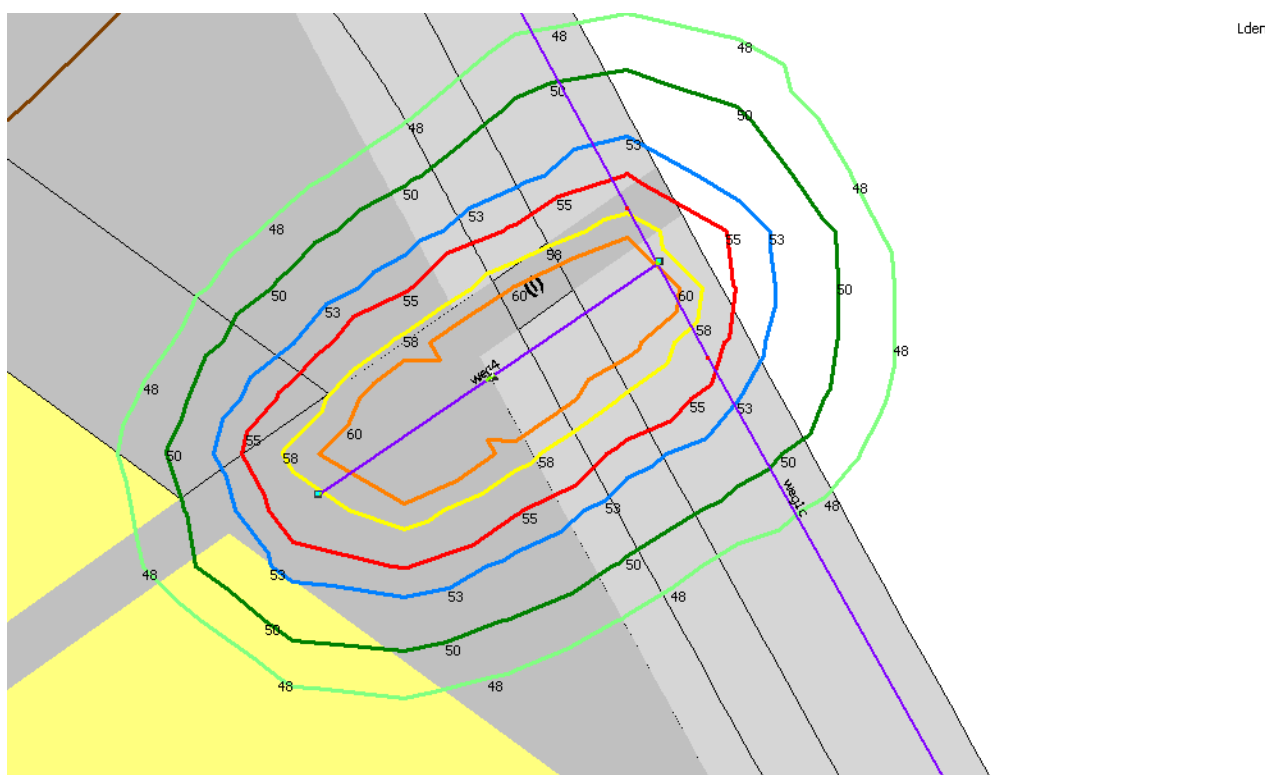
Figuur 3-7: 12 m/excl. 5 dB aftrek (zie ook bijlage 13)
