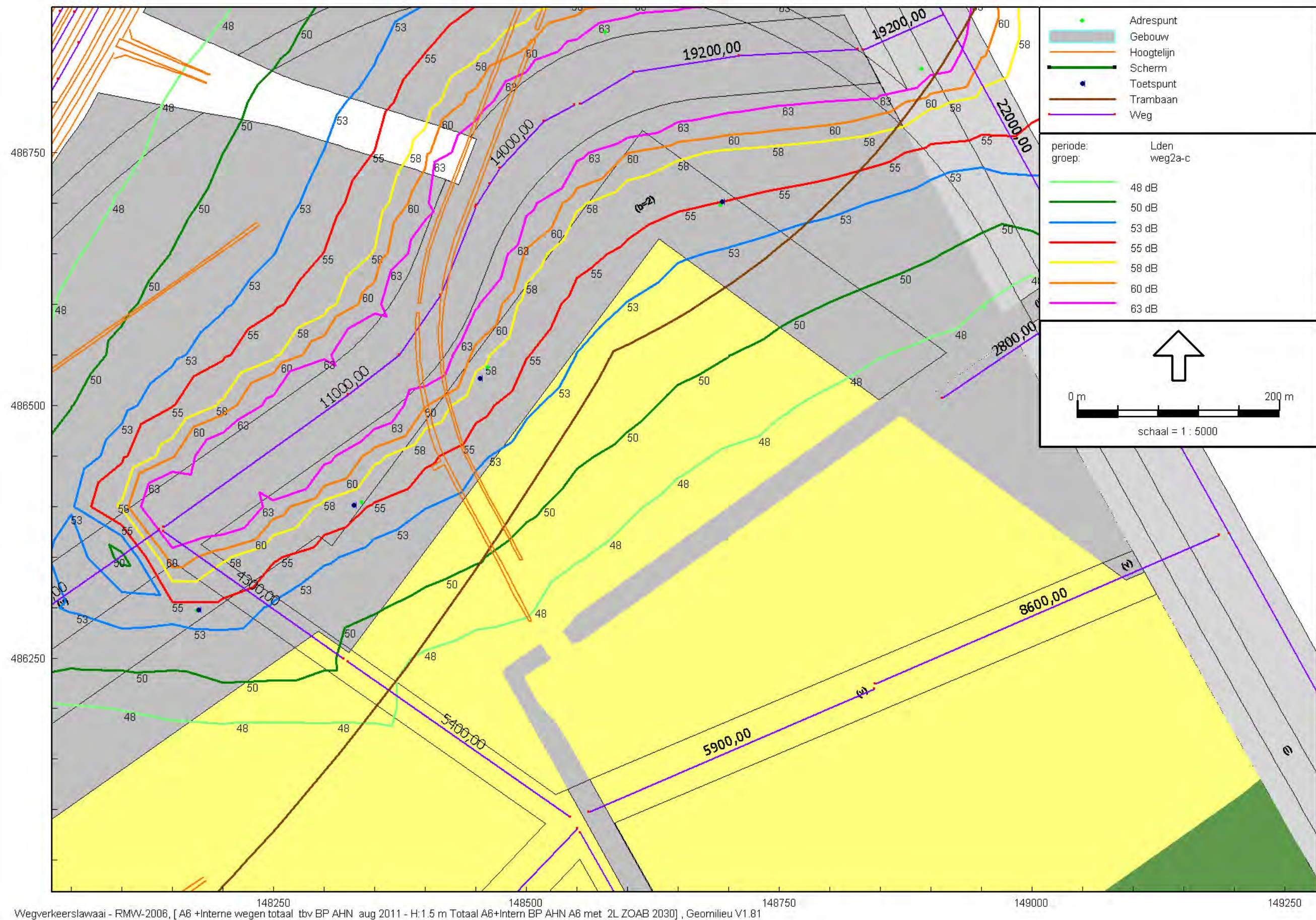
Figuur 2a: weg 2/1.5 m hoogte
