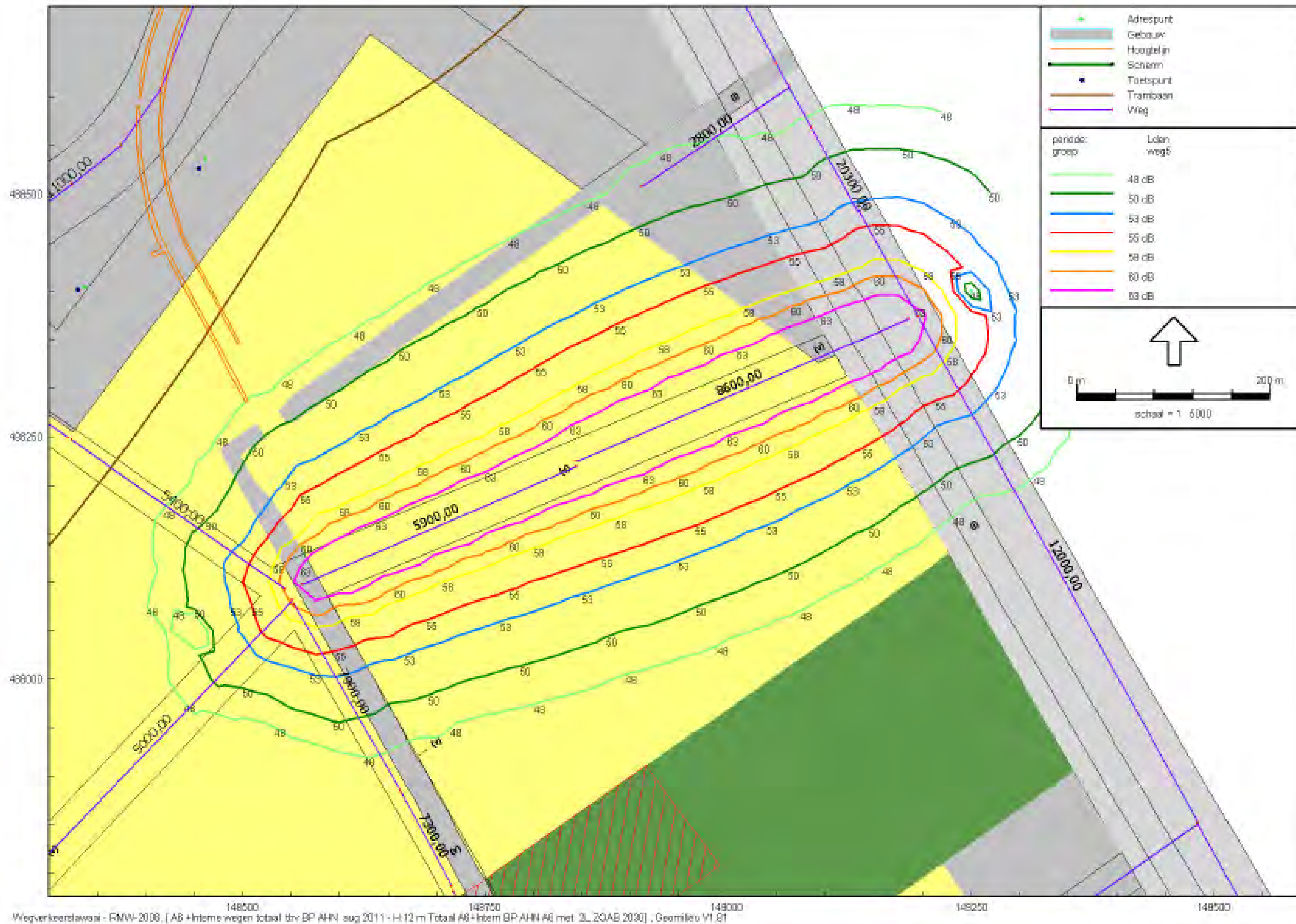
Figuur 5b: weg 5/12 m hoogte
