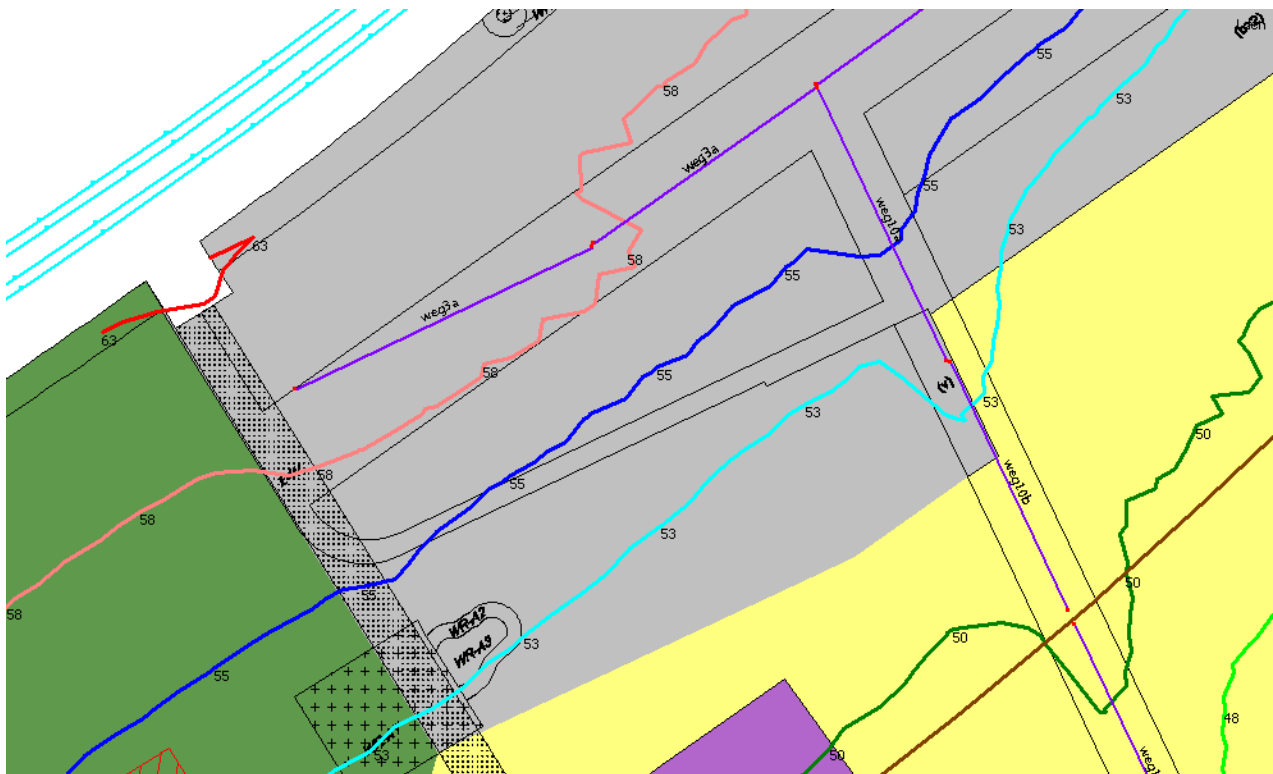
Figuur 3-4: Invloed A6 op 1.5 m hoogte (excl. aftrek 2 dB) (zie ook bijlage 13)
