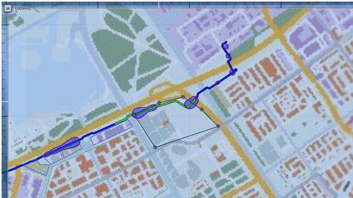
Figuur 4.4 Kilometer leiding behorende bij de maximale overschrijding van de FN-curve voor 2985_leiding-N-533-20-deel-1 van N.V. Nederlandse Gasunie
