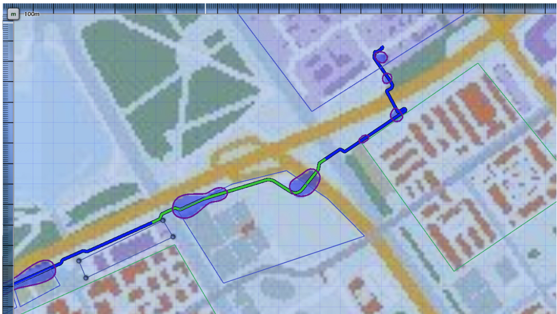
Figuur 3.1 Plaatsgebonden risico voor 2985_leiding-N-533-20-deel-1 van N.V. Nederlandse Gasunie
