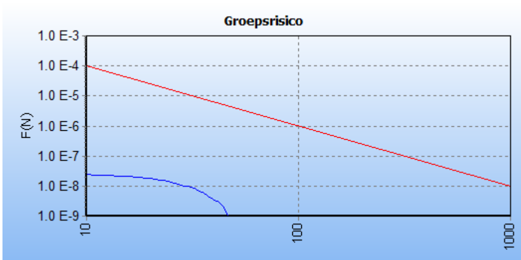
Figuur 5.2 FN curve voor 2985_leiding-N-533-20-deel-1 van N.V. Nederlandse Gasunie voor de kilometer tussen stationing 8320.00 en stationing 9320.00
