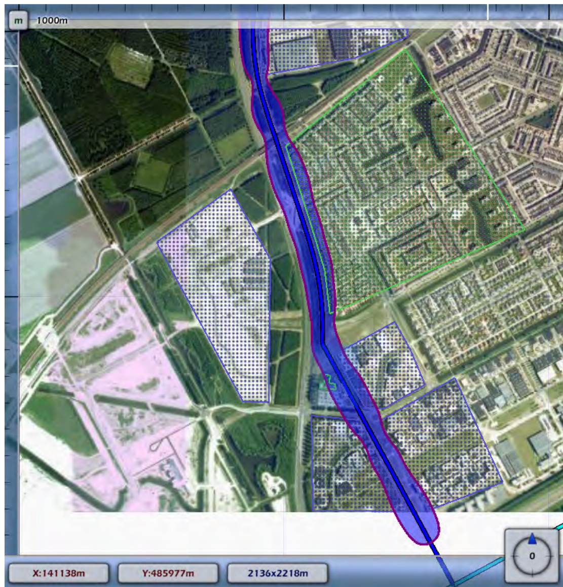
3.1 Figuur 3.2 Plaatsgebonden risico voor 1388_leiding-N-533-20-deel-1 van N.V. Nederlandse Gasunie
