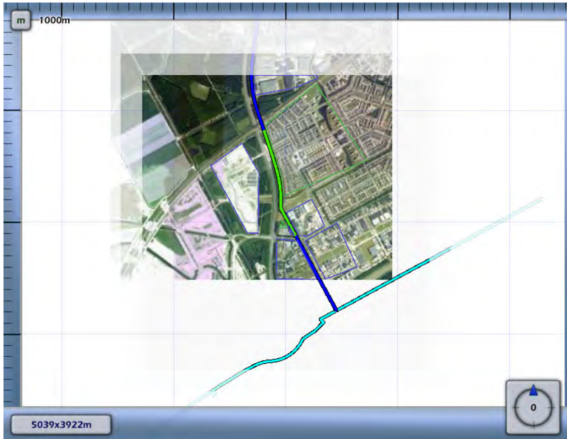
Figuur 4.2 Kilometer leiding behorende bij de maximale overschrijding van de FN-curve voor 1388_leiding-N-533-20-deel-1 van N.V. Nederlandse Gasunie
