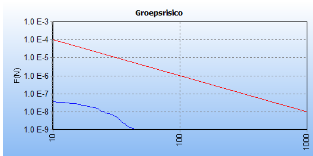
5.2 Figuur 5.2 FN curve voor 1752_leiding-N-533-20-deel-1 van N.V. Nederlandse Gasunie voor de kilometer tussen stationing 1850.00 en stationing 2850.00
