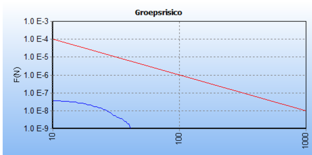
5.1 Figuur 5.2 FN curve voor 1752_leiding-N-533-20-deel-1 van N.V. Nederlandse Gasunie voor de kilometer tussen stationing 1850.00 en stationing 2850.00
