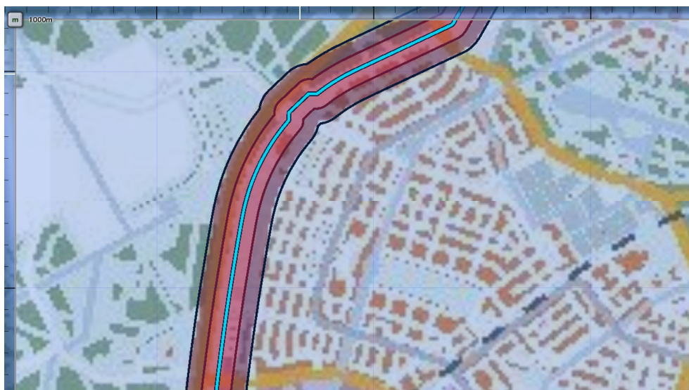
Figuur : invloedsgedebieden buisleidingen, invloedsgedebied (zwart) en 100%-letaliteitsgrens (bruin) [bron: rekenpakket voor buisleidingen CAROLA].
