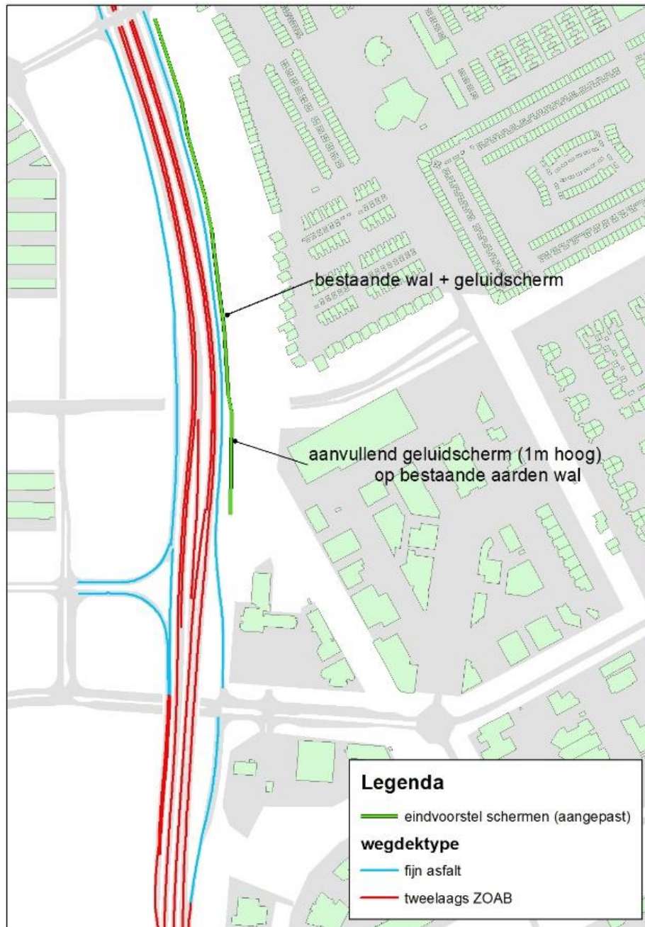
Figuur 3: Detailoverzicht geoptimaliseerde maatregelen
