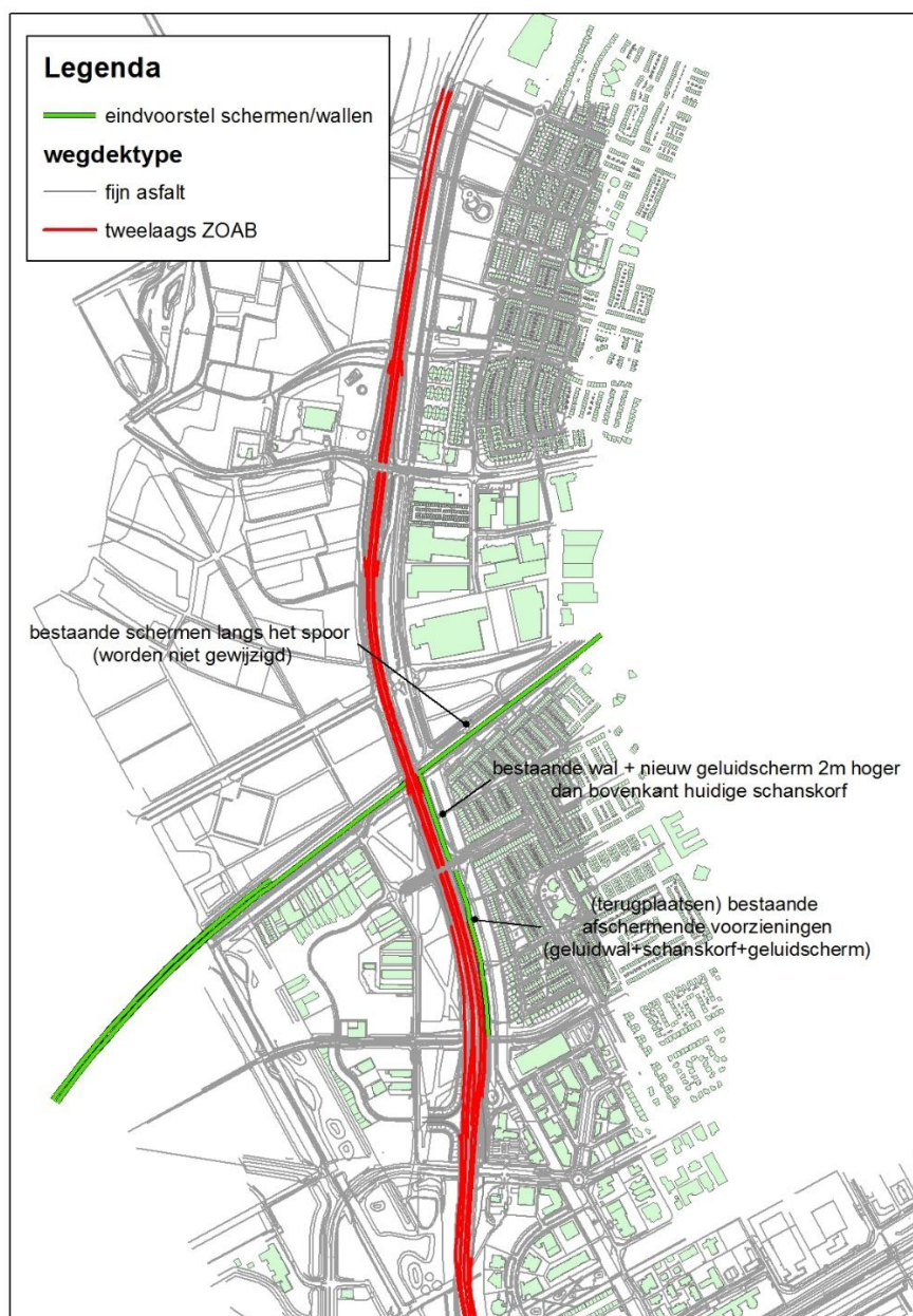
Figuur 8: Overzicht geadviseerde maatregelen Hogering
