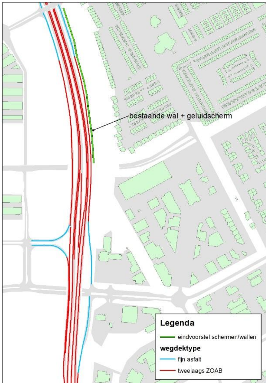
Figuur 2: Detailoverzicht geadviseerde maatregelen Hogering (rapport 'Capaciteitsuitbreiding Hogering Almere, Akoestisch onderzoek' d.d. 29 augustus 2017)
