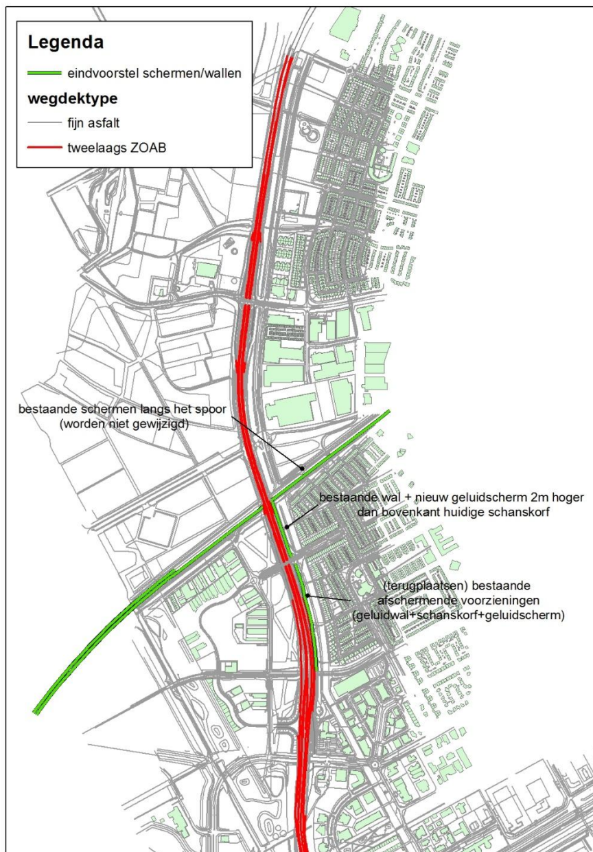
Figuur 1: Overzicht geadviseerde maatregelen Hogering (rapport 'Capaciteitsuitbreiding Hogering Almere, Akoestisch onderzoek' d.d. 29 augustus 2017)
