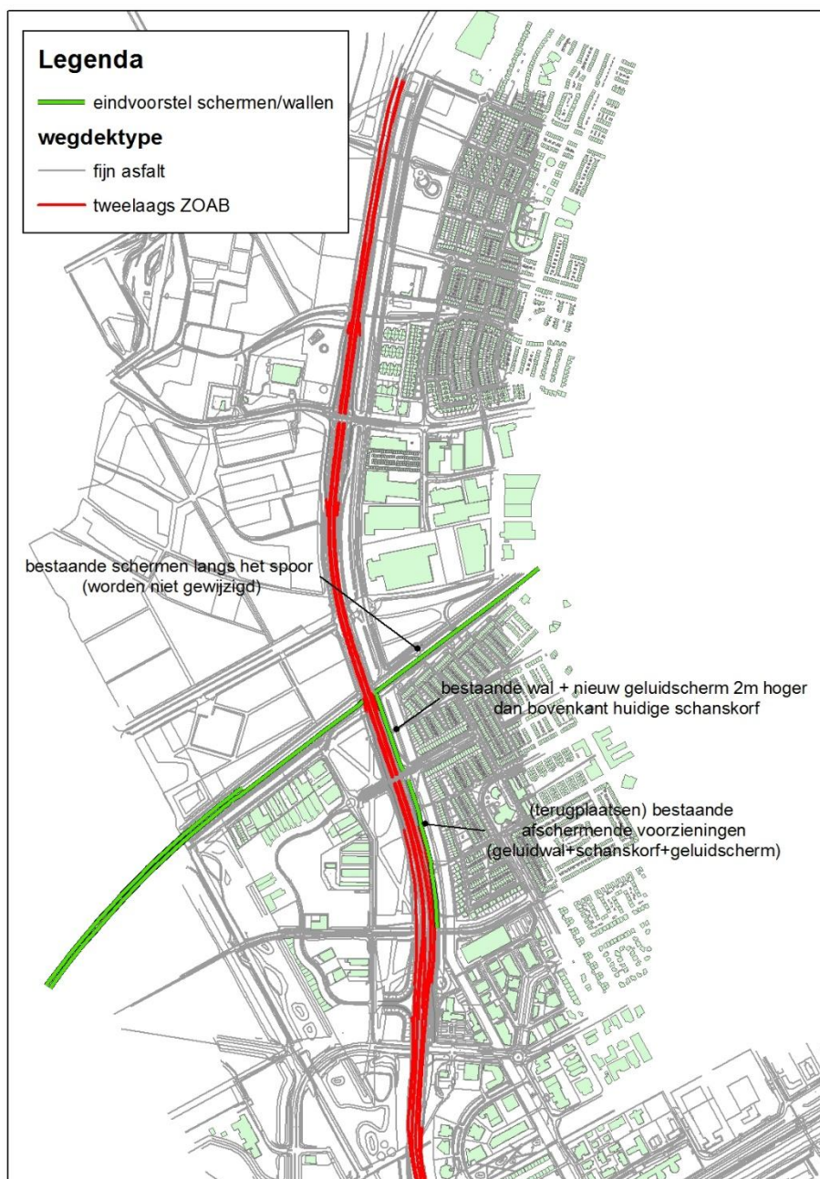
Figuur 9: Overzicht geadviseerde maatregelen Hogering
