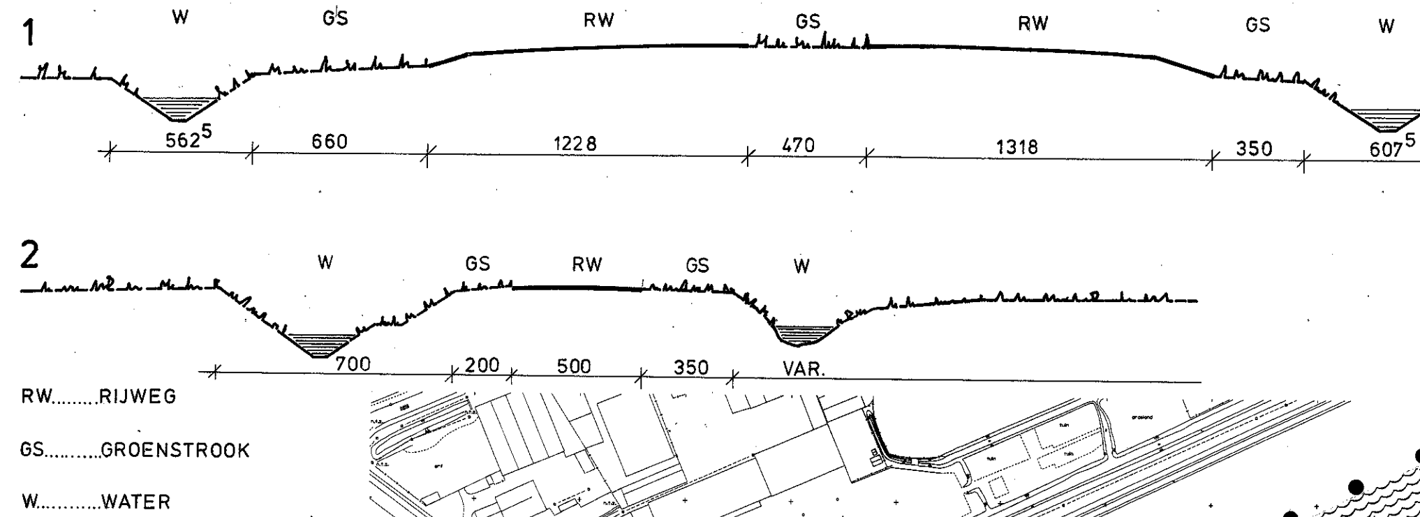
DWARSPROFIELEN SCHAAL 1:200
