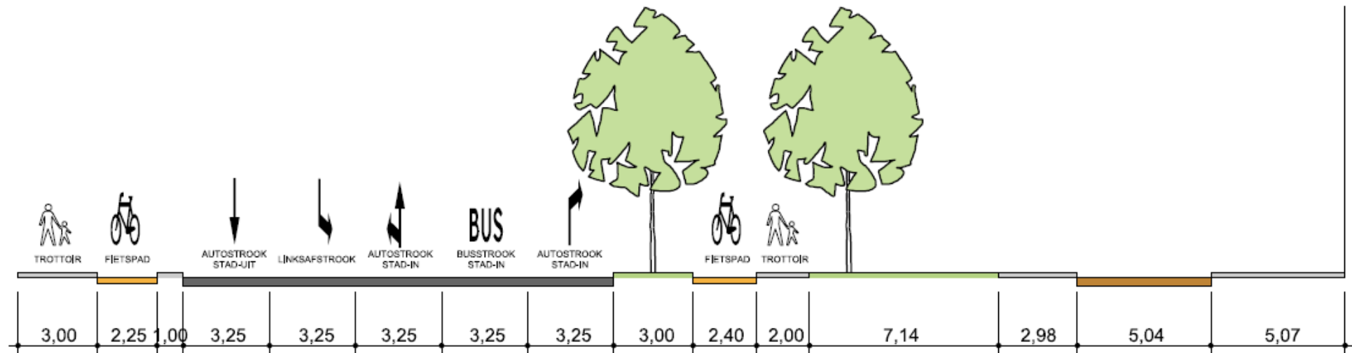
dwarsprofiel 1: Sontweg
