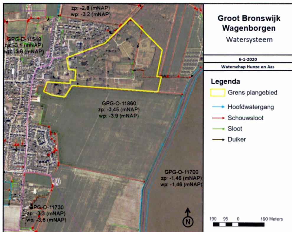
Figuur 1: Watersysteem
