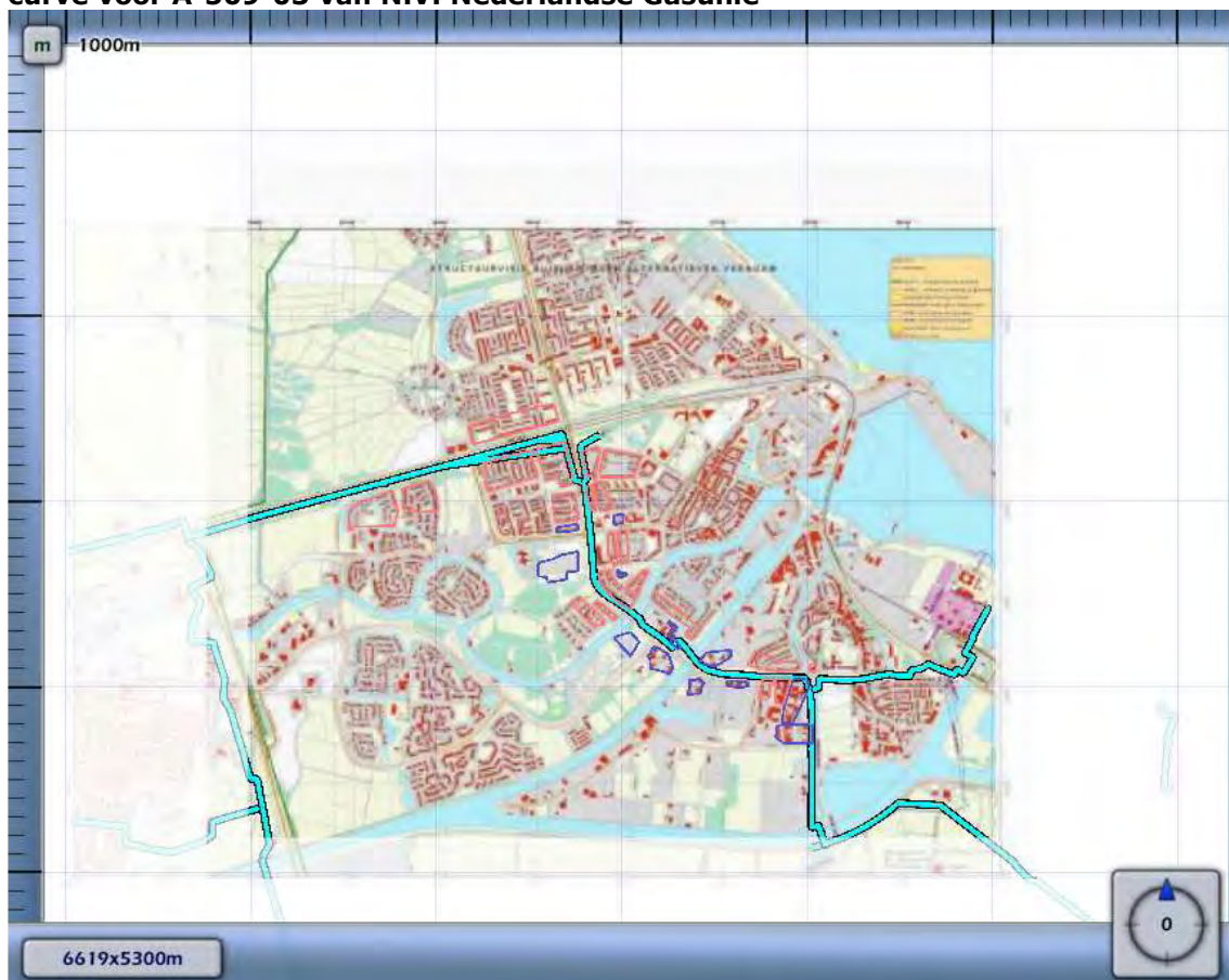
Figuur 4.2 Kilometer leiding behorende bij de maximale overschrijding van de FN-curve voor A-509-03 van N.V. Nederlandse Gasunie
