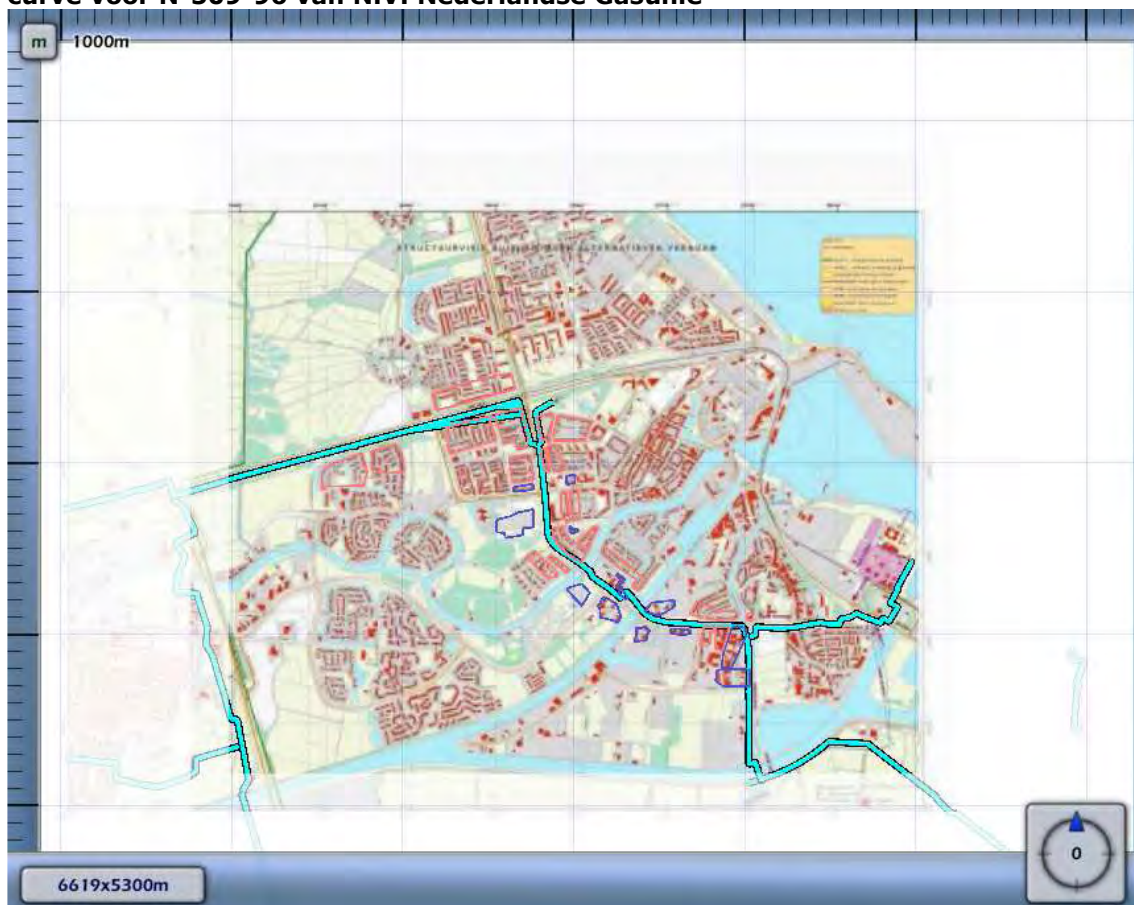
Figuur 4.4 Kilometer leiding behorende bij de maximale overschrijding van de FN-curve voor N-509-96 van N.V. Nederlandse Gasunie
