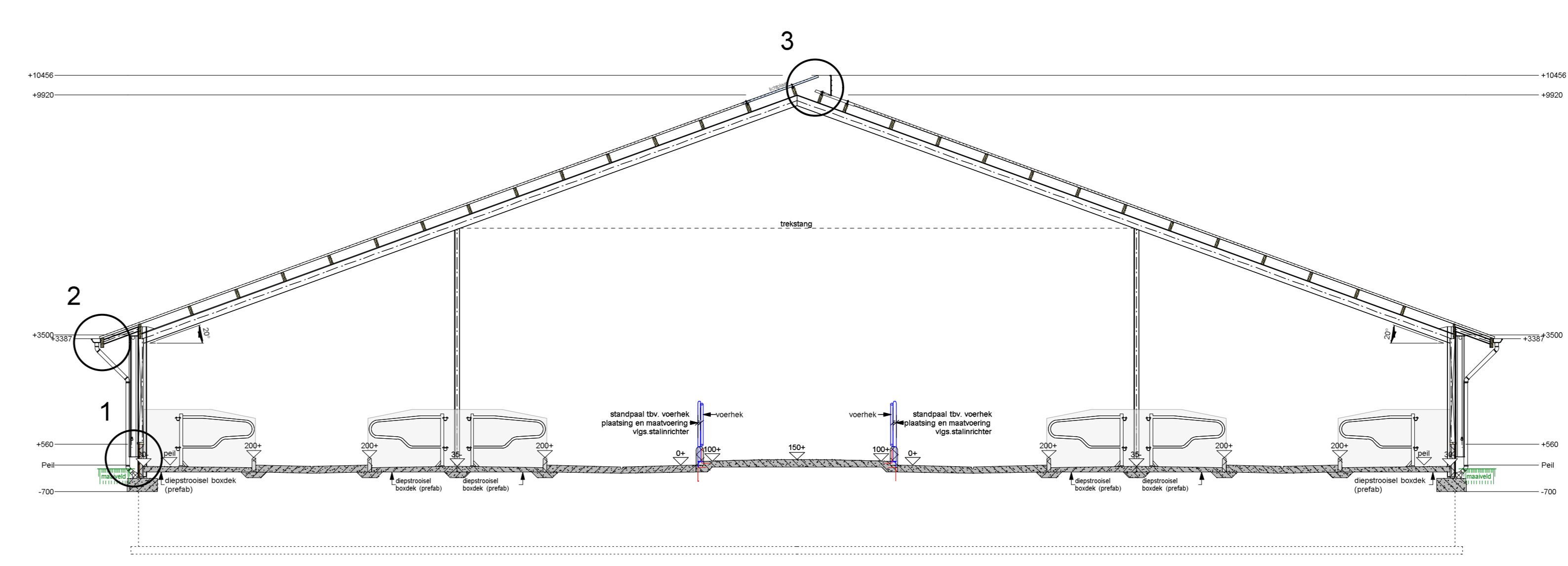
DOORSNEDE A-A
