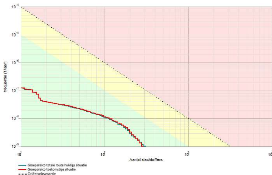
Figuur 4.4 Groepsrisico totale route huidige en toekomstige situatie voor de weg N33
