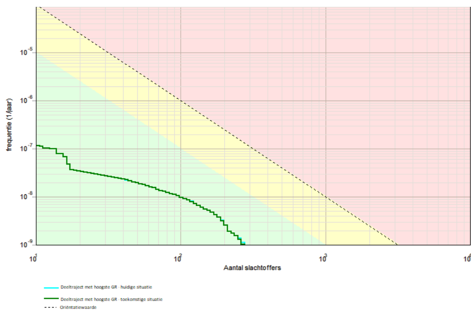
Figuur 4.5 Deeltraject met hoogste groepsrisico voor de huidige en toekomstige situatie voor de weg N33
