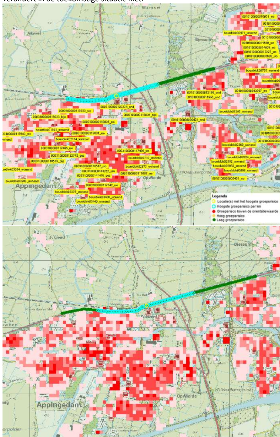
Figuur 4.10 Deeltraject voor de weg met het hoogste GR in de huidige situatie (boven) en toekomstige situatie (onder).
