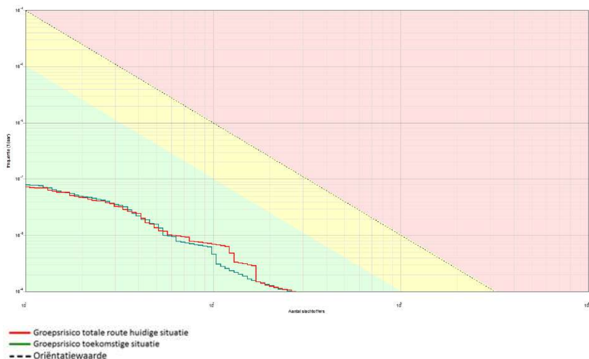
Figuur 4.6 Groepsrisico totale route huidige en toekomstige situatie voor de weg N360
