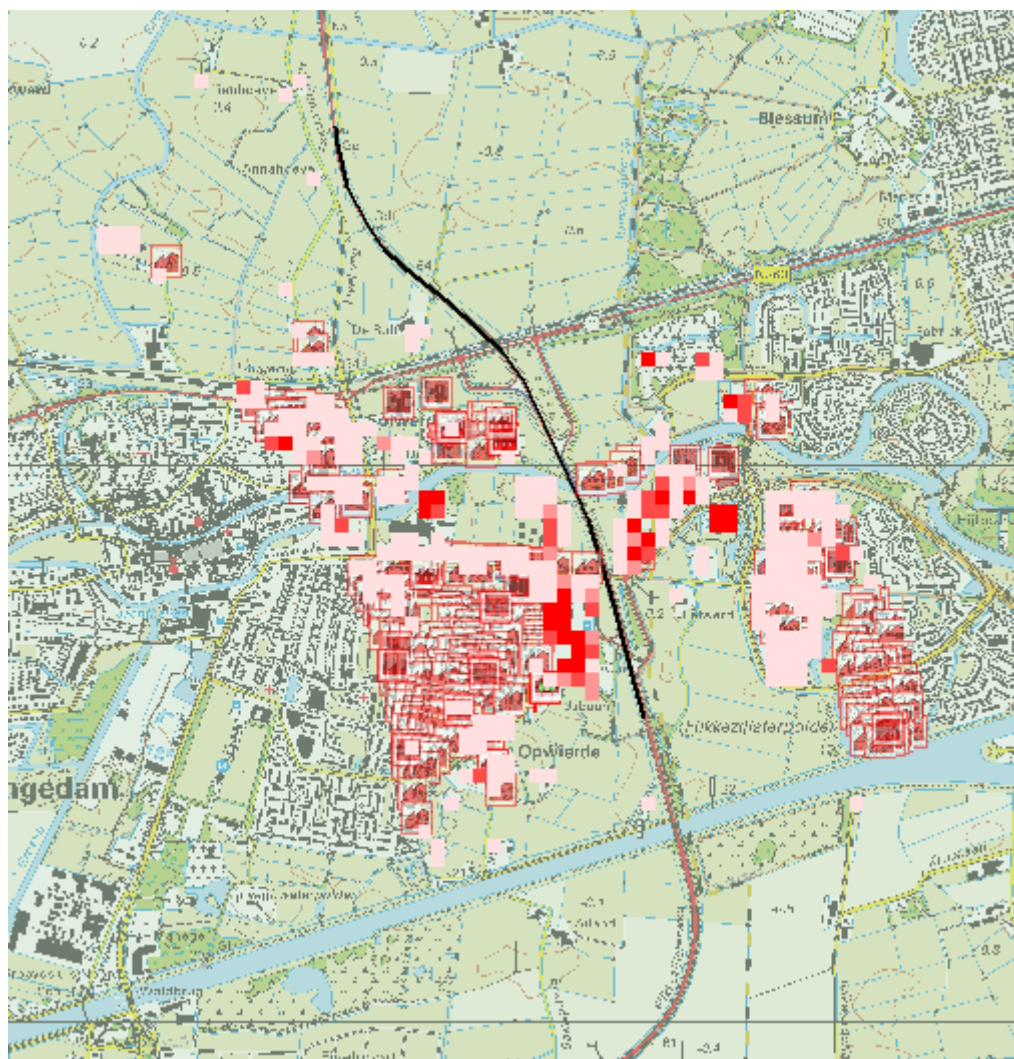
Figuur 3.2 Geïnvventariseerde personendichtheid rondom het wegtraject N33 (bron: uitsnede RBM II berekening)
