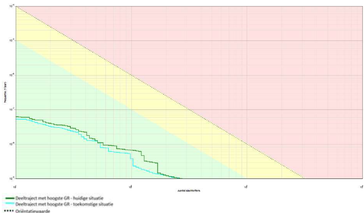
Figuur 4.7 Deeltraject met hoogste groepsrisico voor de huidige en toekomstige situatie voor de weg N360
