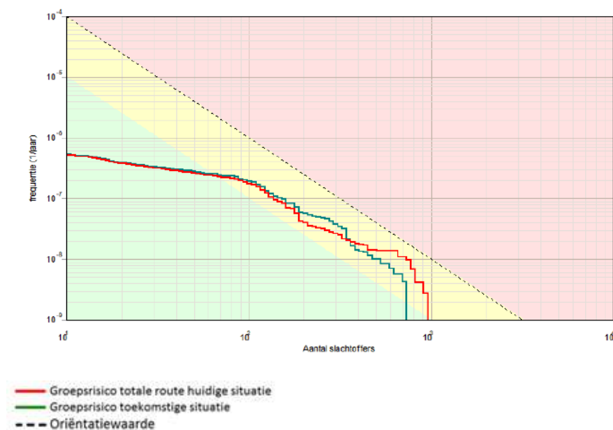
Figuur 4.2 Groepsrisico totale route huidige en toekomstige situatie voor het spoor
