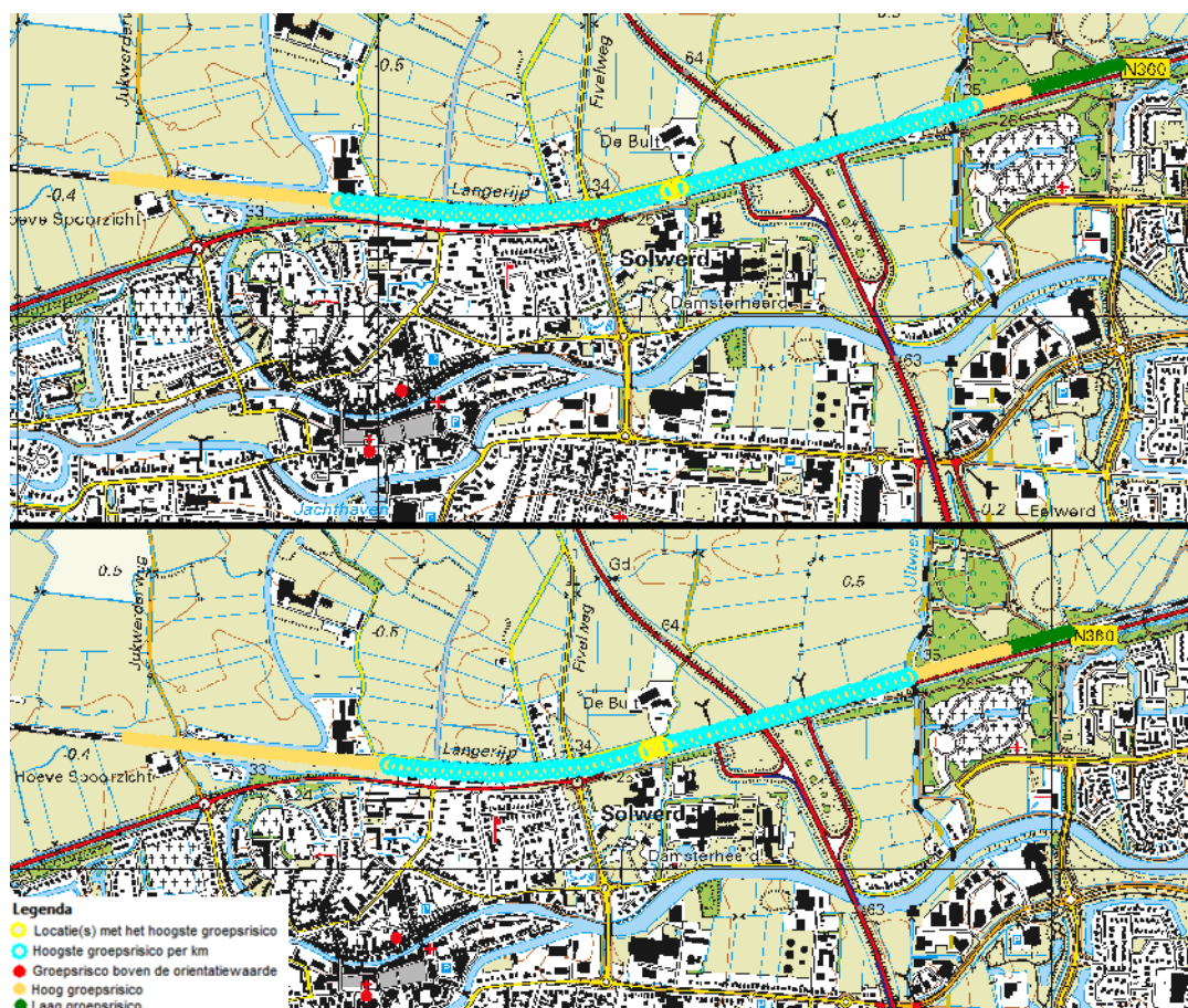
Figuur 4.8 Deeltraject voor het spoor met het hoogste GR in de huidige situatie (boven) en toekomstige situatie (onder).
