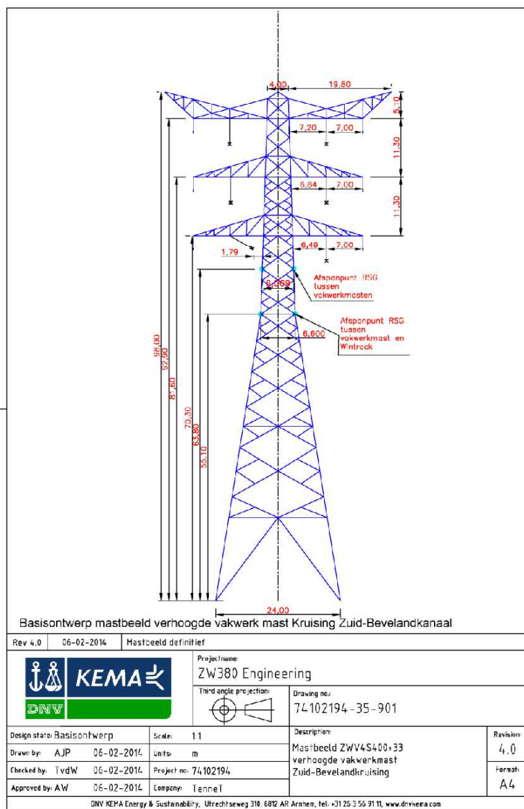
Afbeelding N11, mastbeeld ZWV4S400+33
