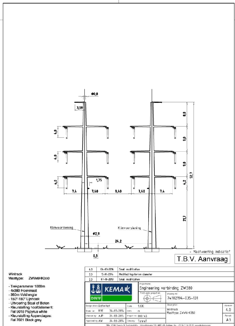
Afbeelding M12, mastbeeld ZWW6HK350
