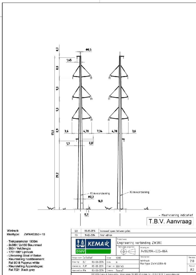
Afbeelding N7, mastbeeld ZWW4S350+10
