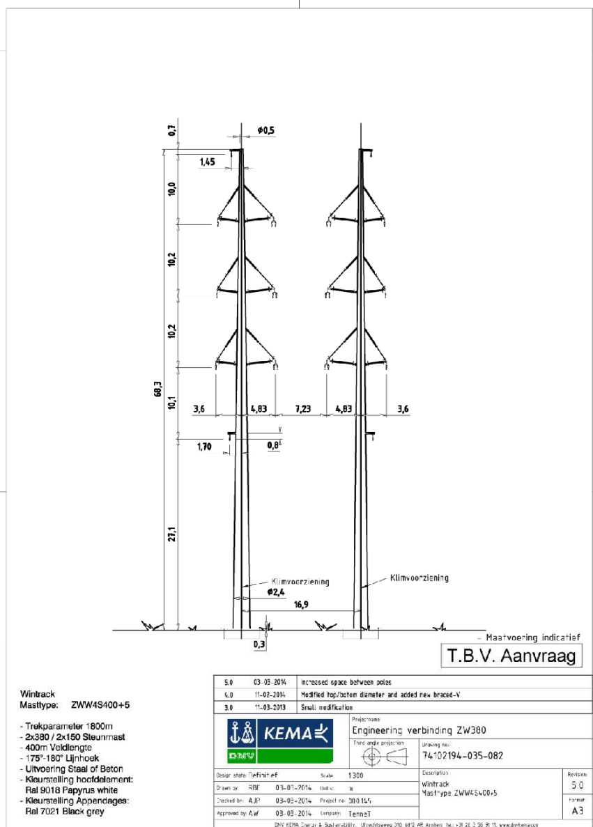
Afbeelding N9, mastbeeld ZWW4S400+5
