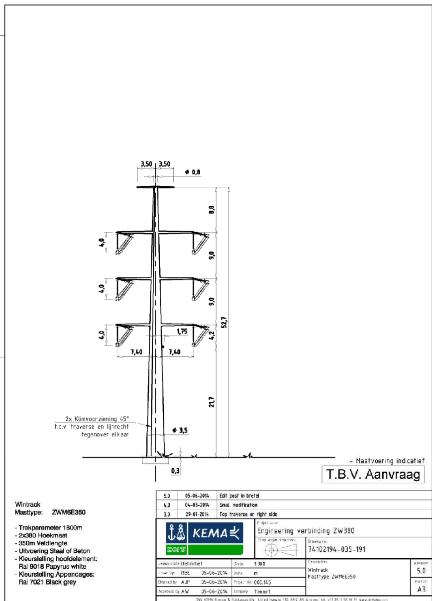
Afbeelding M2, mastbeeld ZWM6E350
