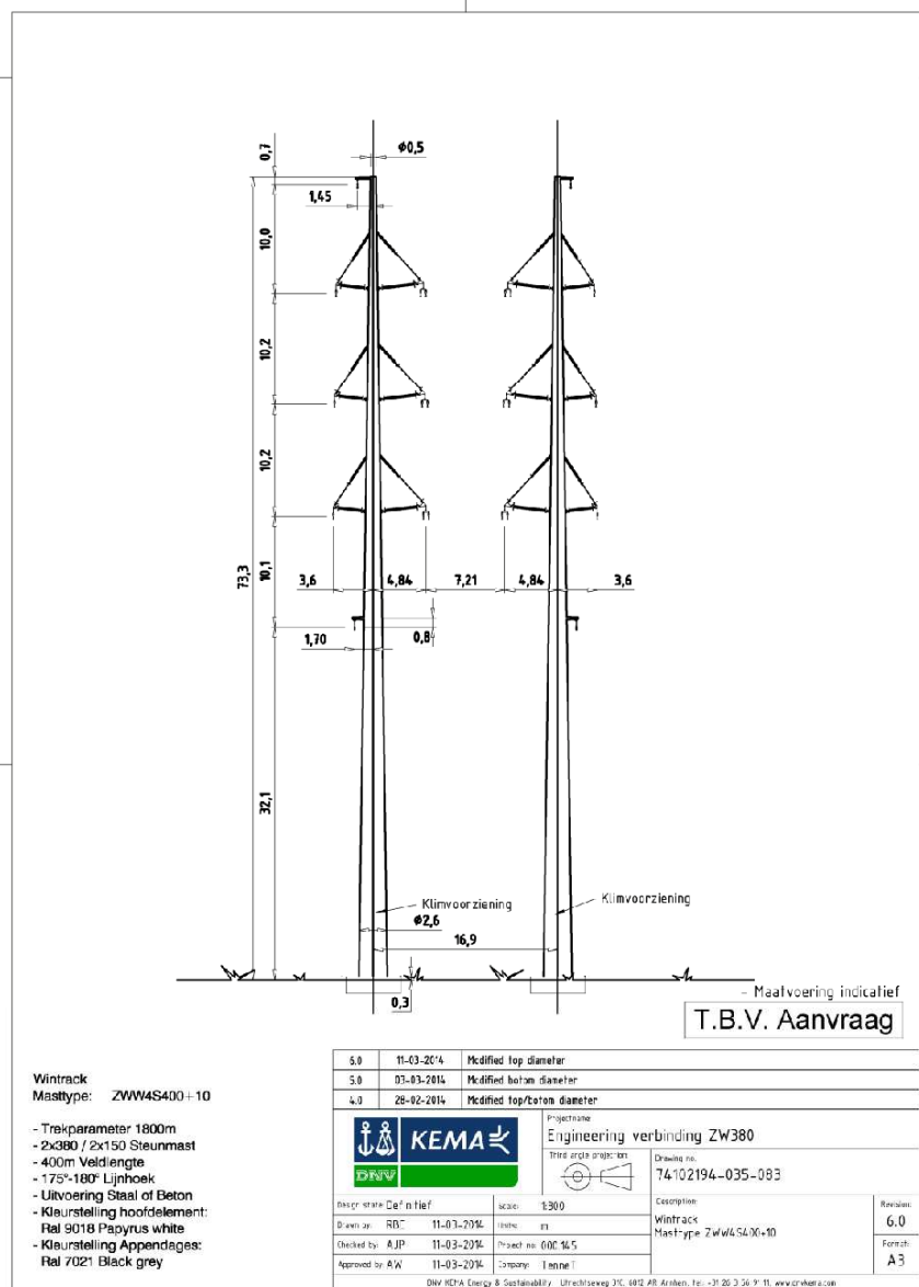
Afbeelding N10, mastbeeld ZWW4S400+10
