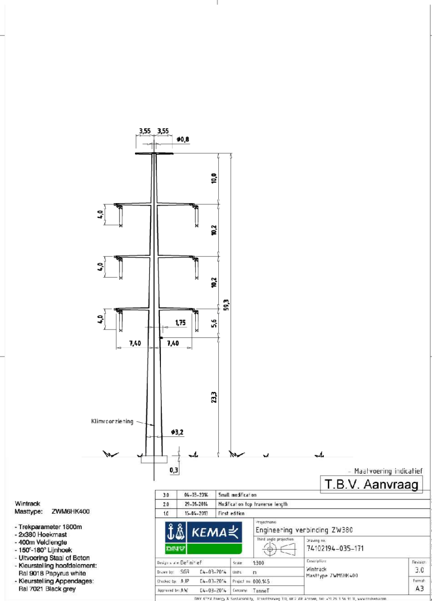
Afbeelding N1, mastbeeld ZWM6HK400
