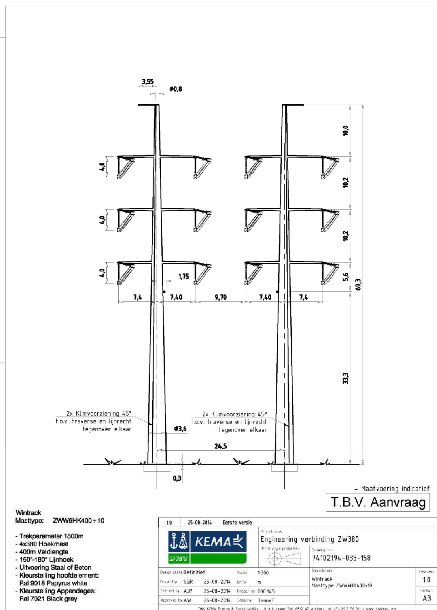
Afbeelding M9, mastbeeld ZWW6HK400+10
