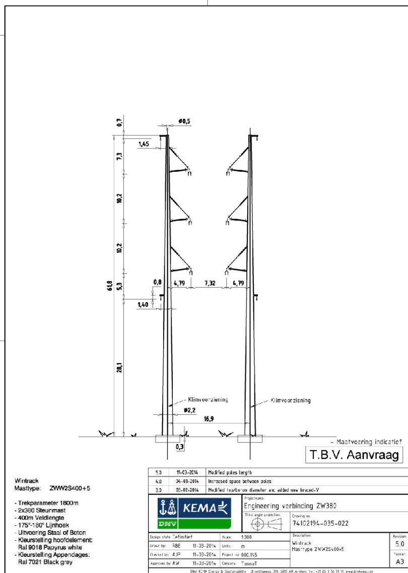
Afbeelding N4, mastbeeld ZWW2S400+5
