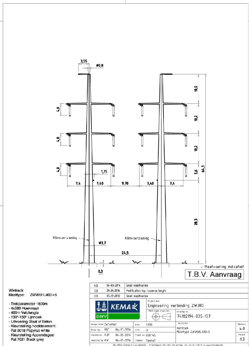
Afbeelding M8, mastbeeld ZWW6HL400+5
