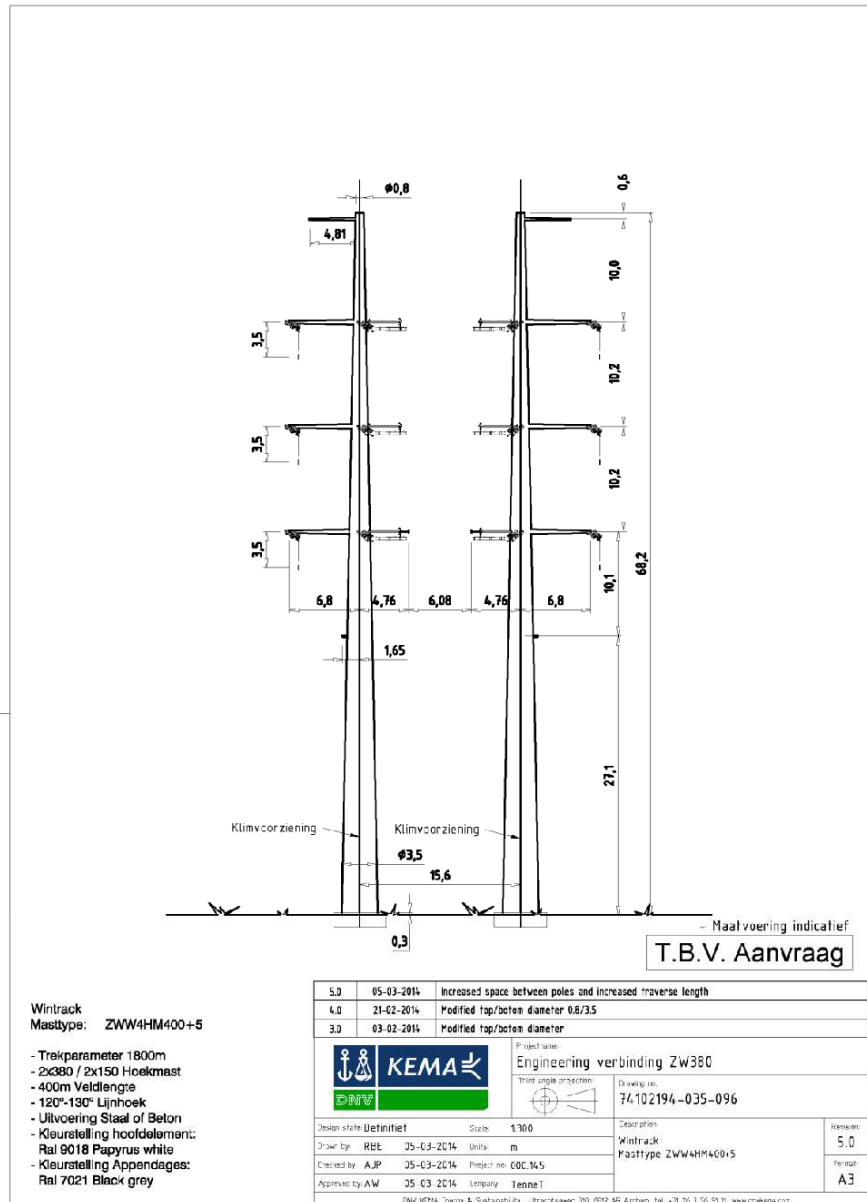
Afbeelding B21, mastbeeld ZWW4HM400+5
