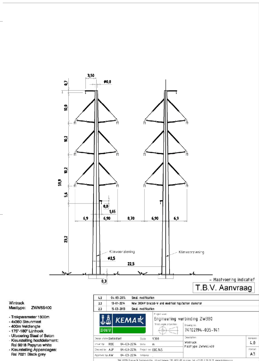
Afbeelding M6, mastbeeld ZWW6S00
