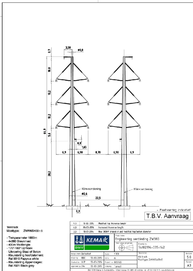
Afbeelding M4, mastbeeld ZWW6S400+5
