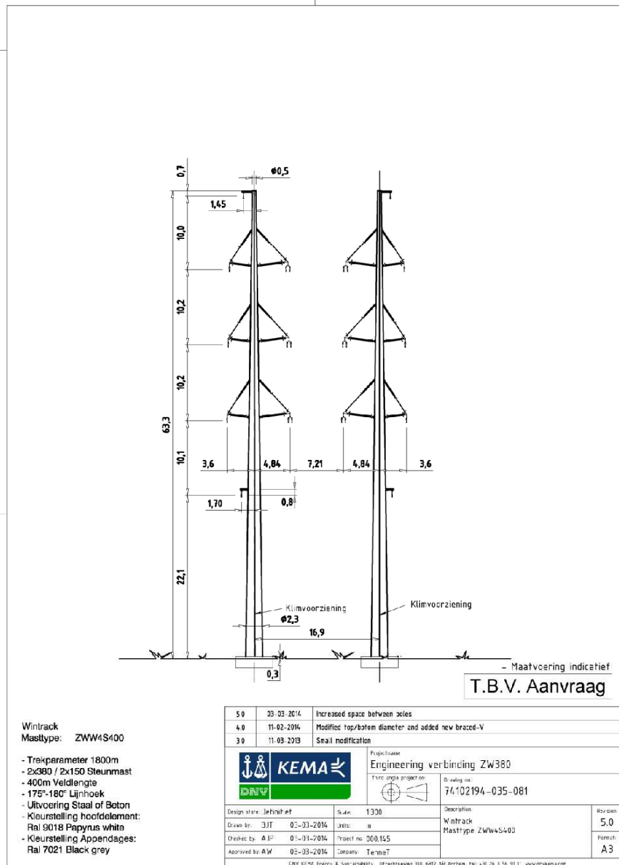
Afbeelding B14, mastbeeld ZWW4S400
