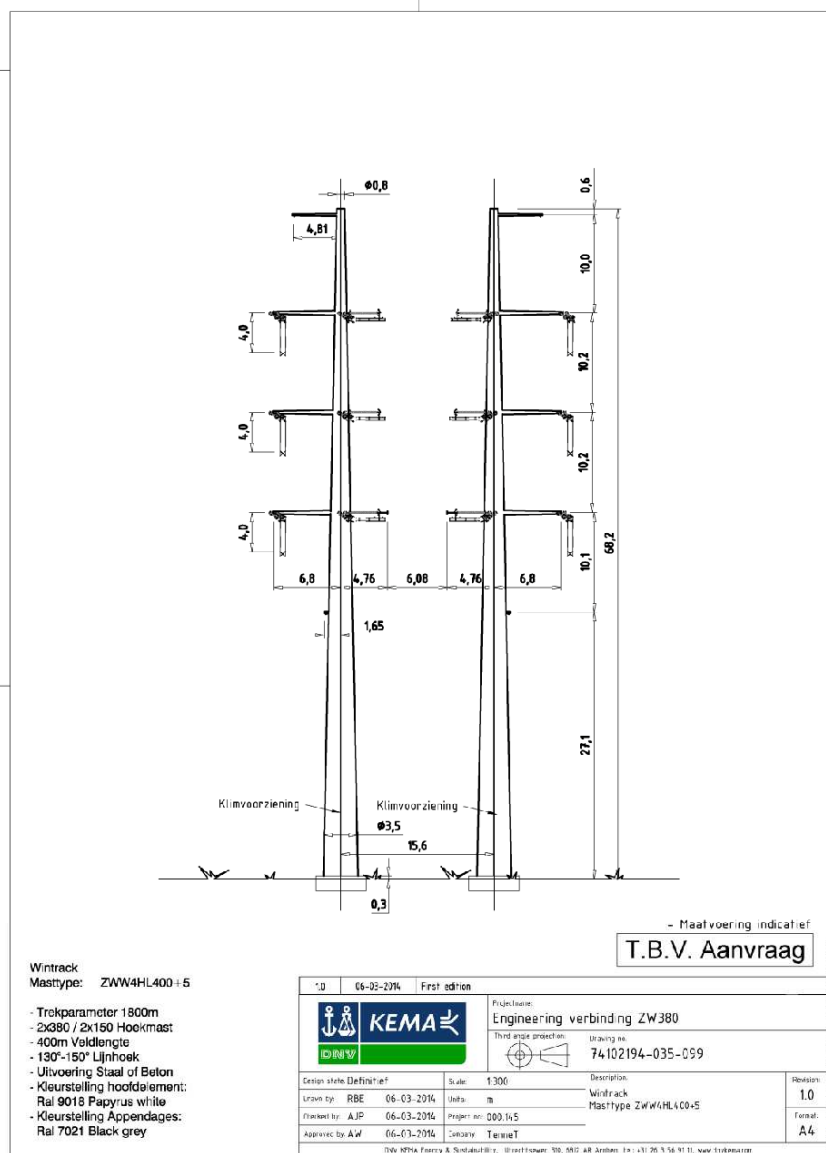
Afbeelding N6, mastbeeld ZWW4HL400+5
