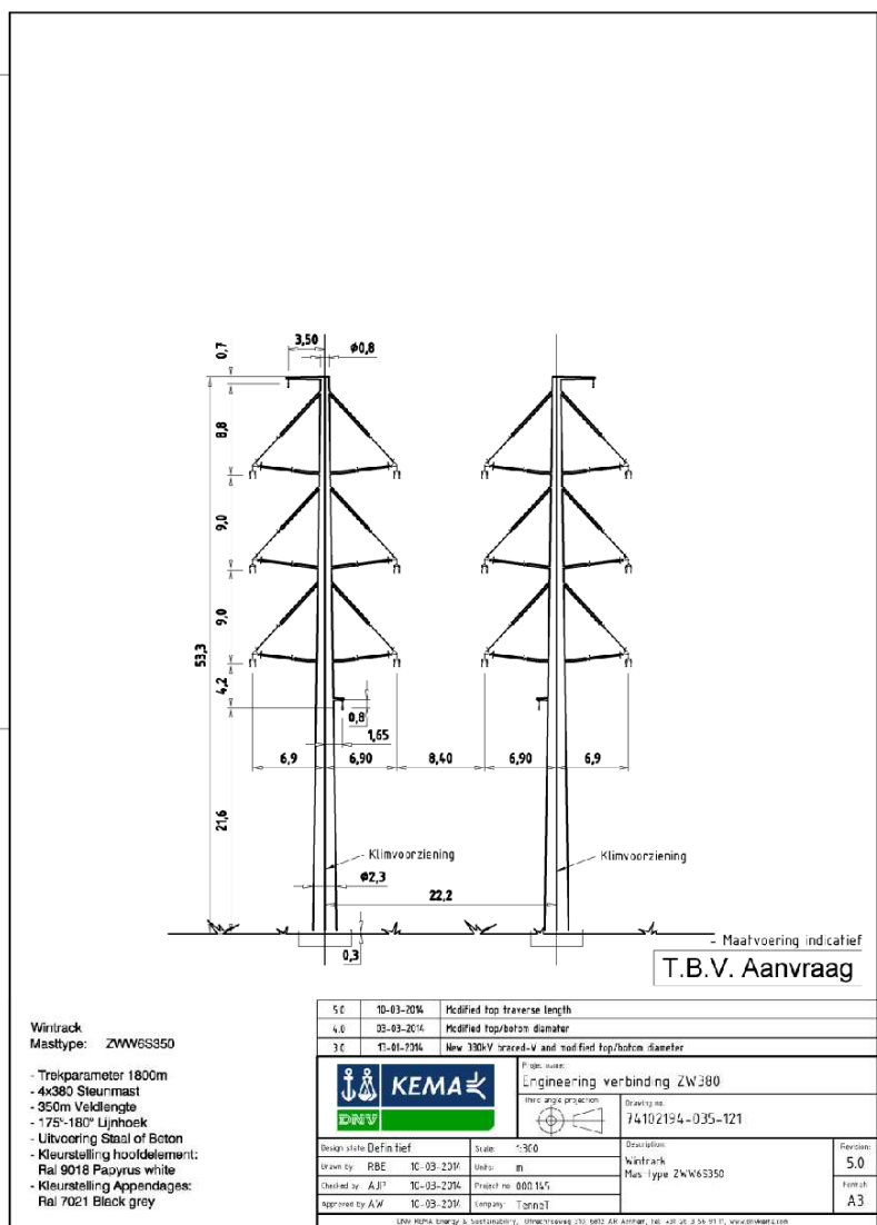
Afbeelding M11, mastbeeld ZWW6S35
