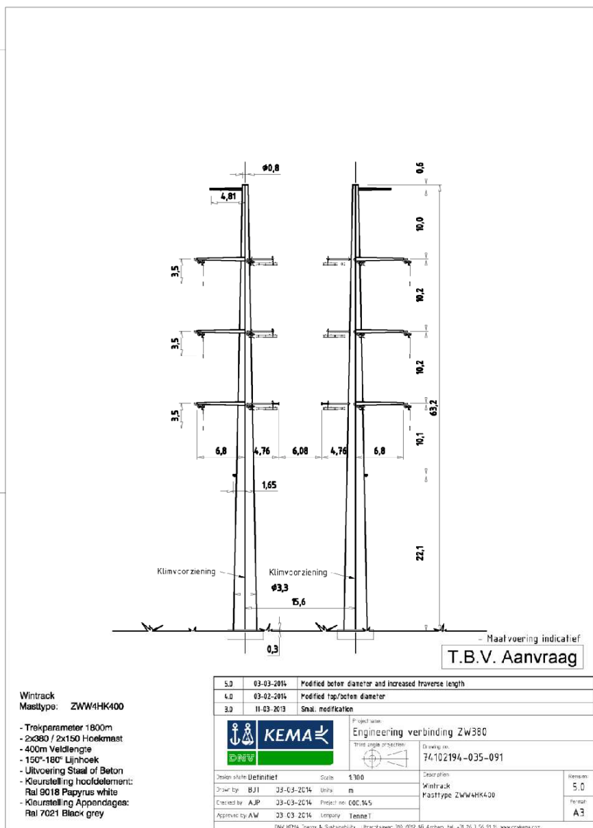
Afbeelding N20, mastbeeld ZWW4HK400
