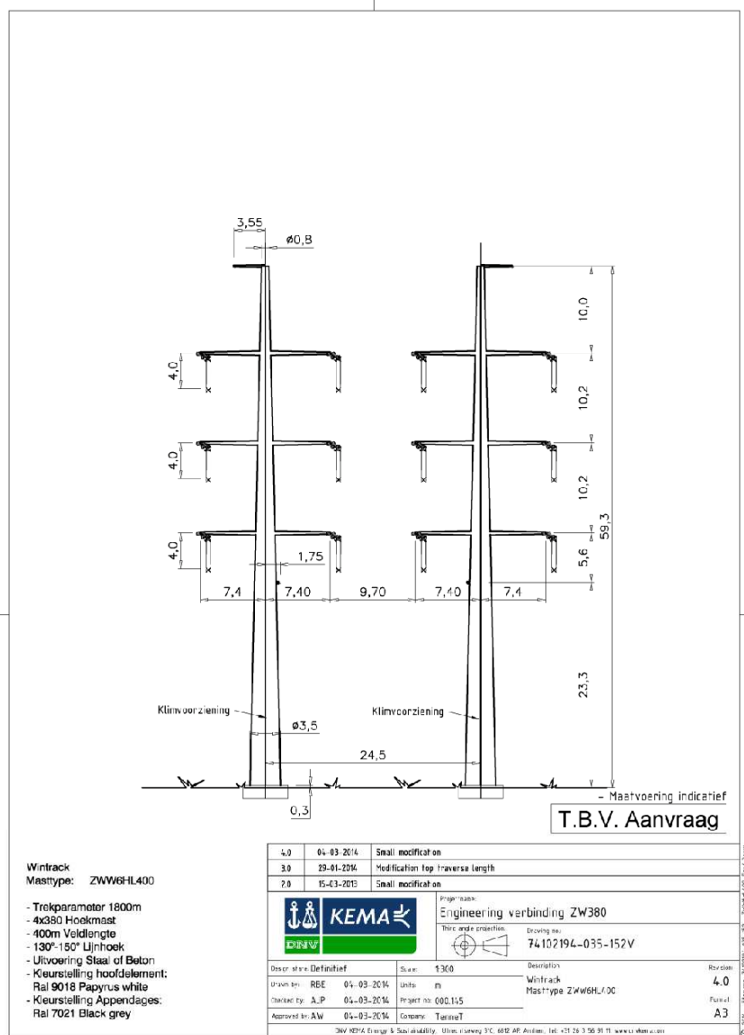
Afbeelding M10, mastbeeld ZWW6HL400
