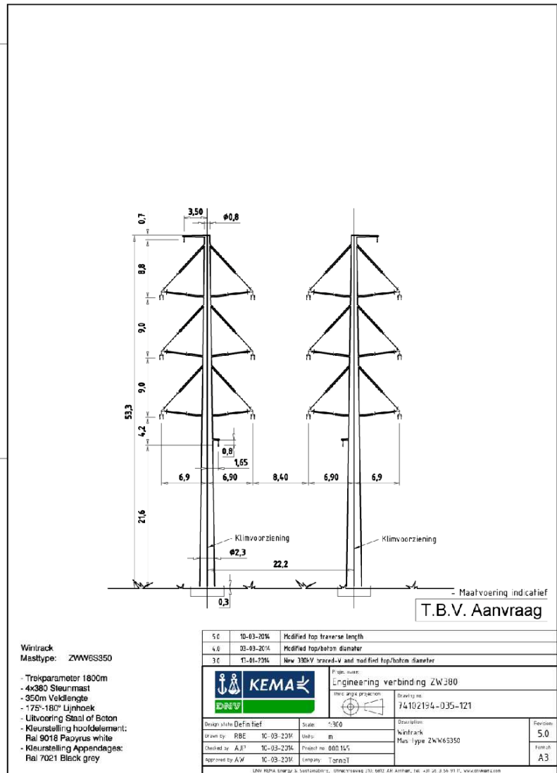
Afbeelding A11, mastbeeld ZWW6S35
