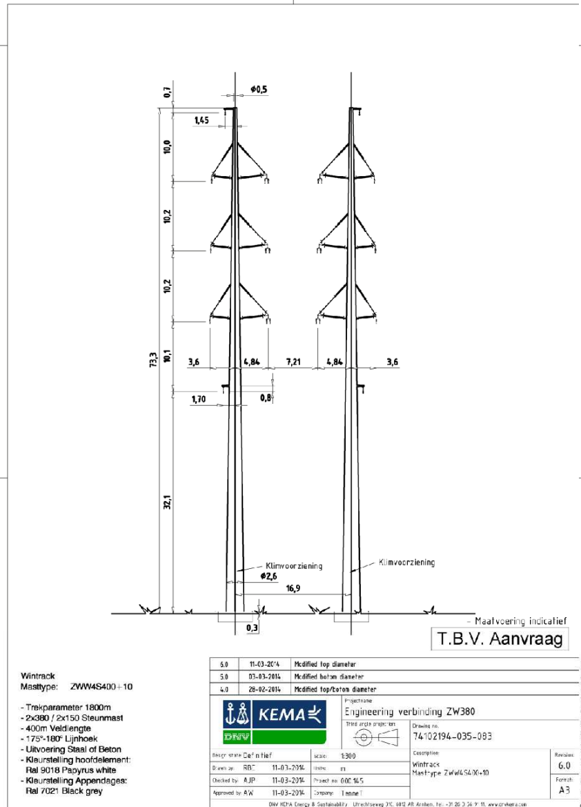
Afbeelding B10, mastbeeld ZWW4S400+10
