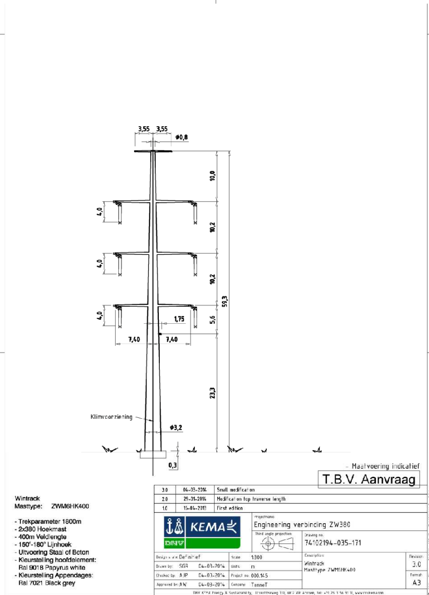
Afbeelding B1, mastbeeld ZWM6HK400
