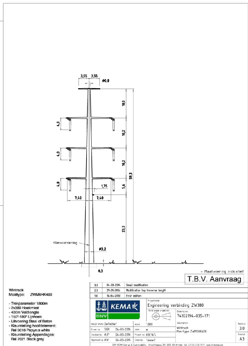
Afbeelding A13, mastbeeld ZWM6HK400
