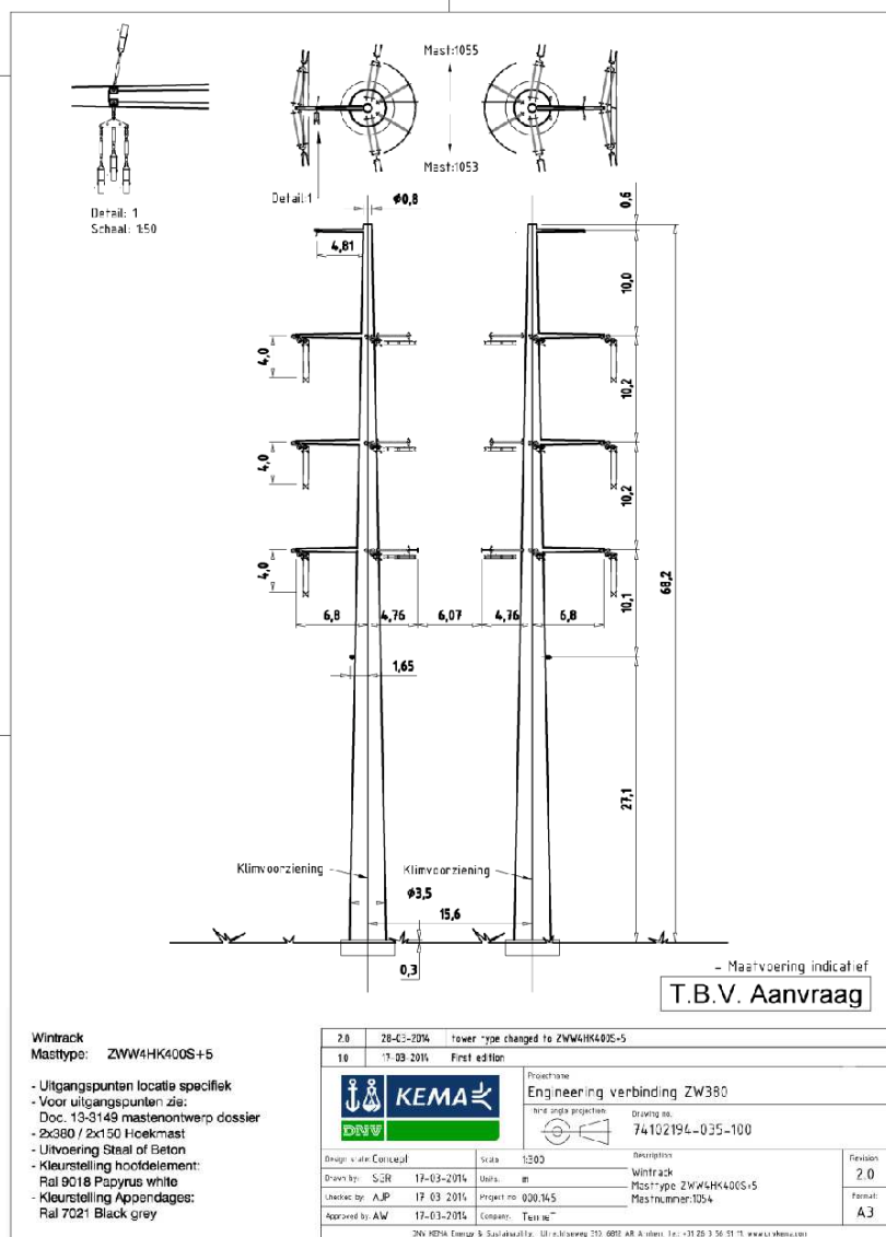
Afbeelding N5, mastbeeld ZWW4HK400S+5
