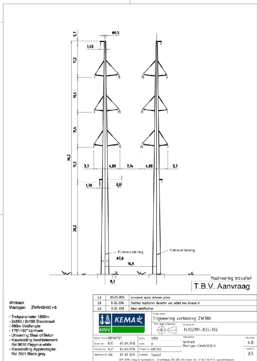
Afbeelding N15, mastbeeld ZWW4S450+5
