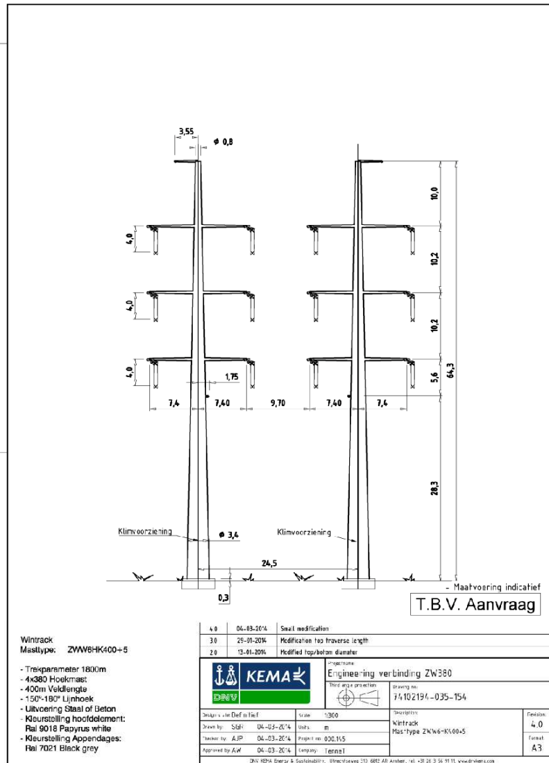
Afbeelding A5, mastbeeld ZWW6HK400+5
