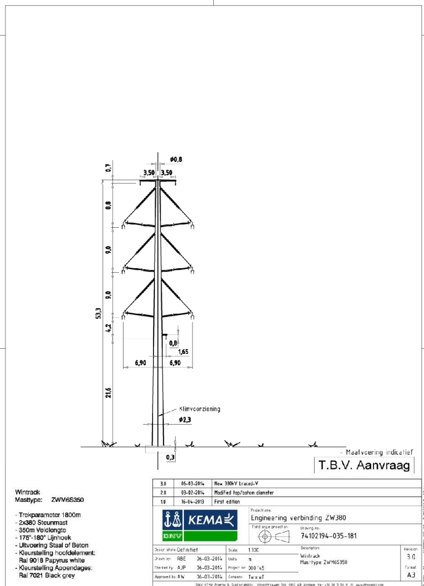
Afbeelding N2, mastbeeld ZWM6S350
