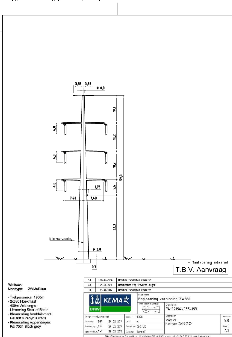
Afbeelding M3, mastbeeld ZWM6E400
