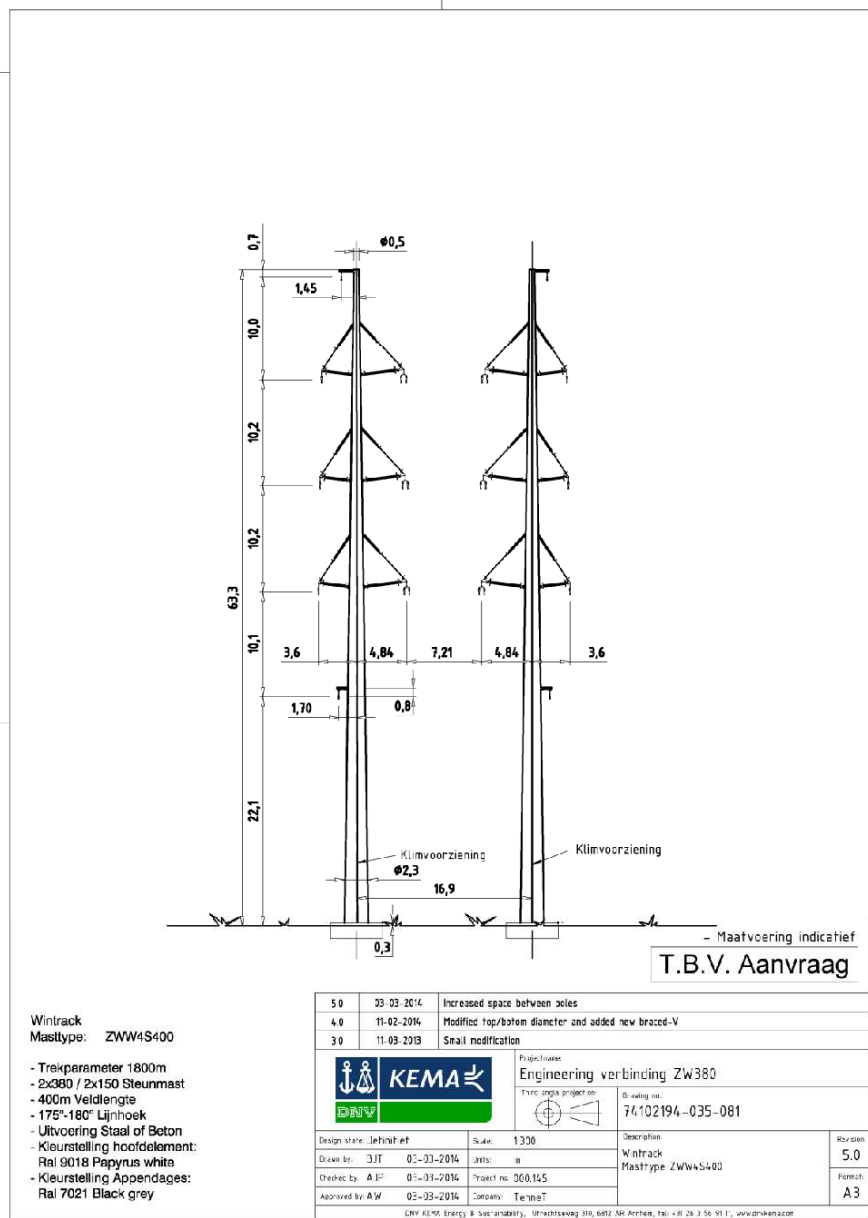
Afbeelding N14, mastbeeld ZWW4S400
