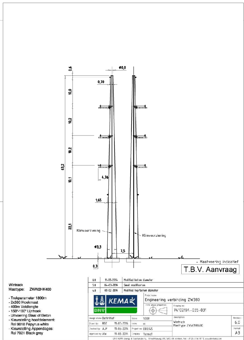
Afbeelding N3, mastbeeld ZWW2HK400
