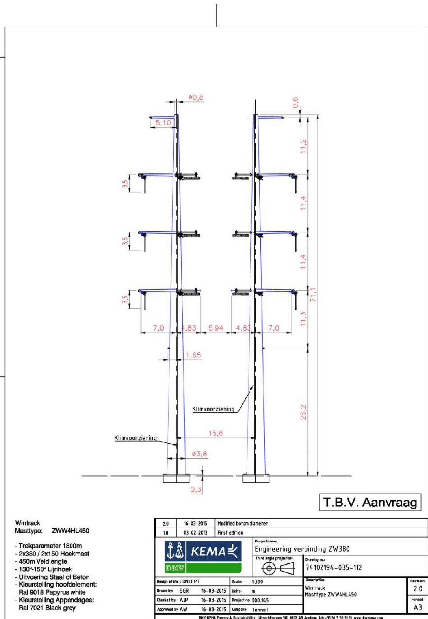
Afbeelding N19, mastbeeld ZWW4HL450
