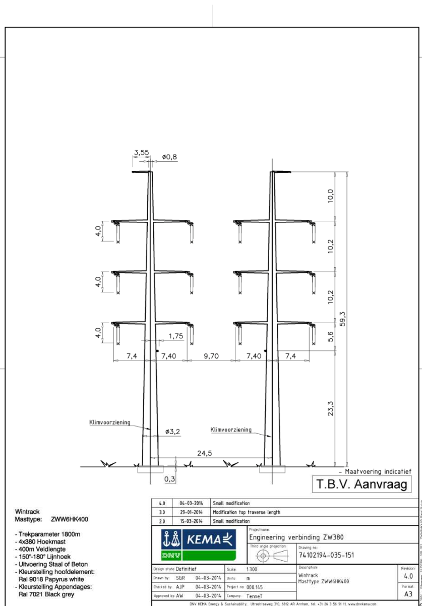
Afbeelding M7, mastbeeld ZWW6HK400
