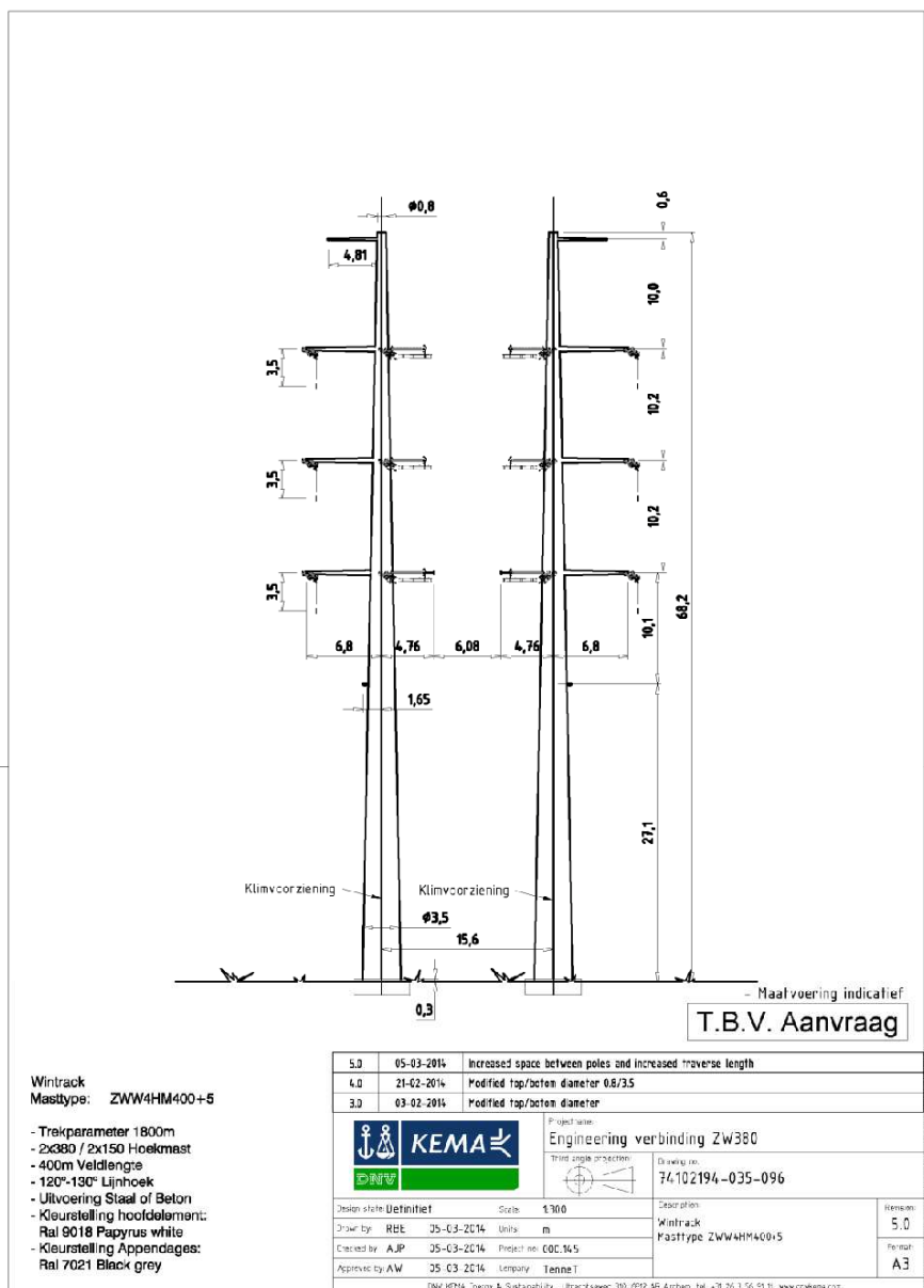
Afbeelding N21, mastbeeld ZWW4HM400+5
