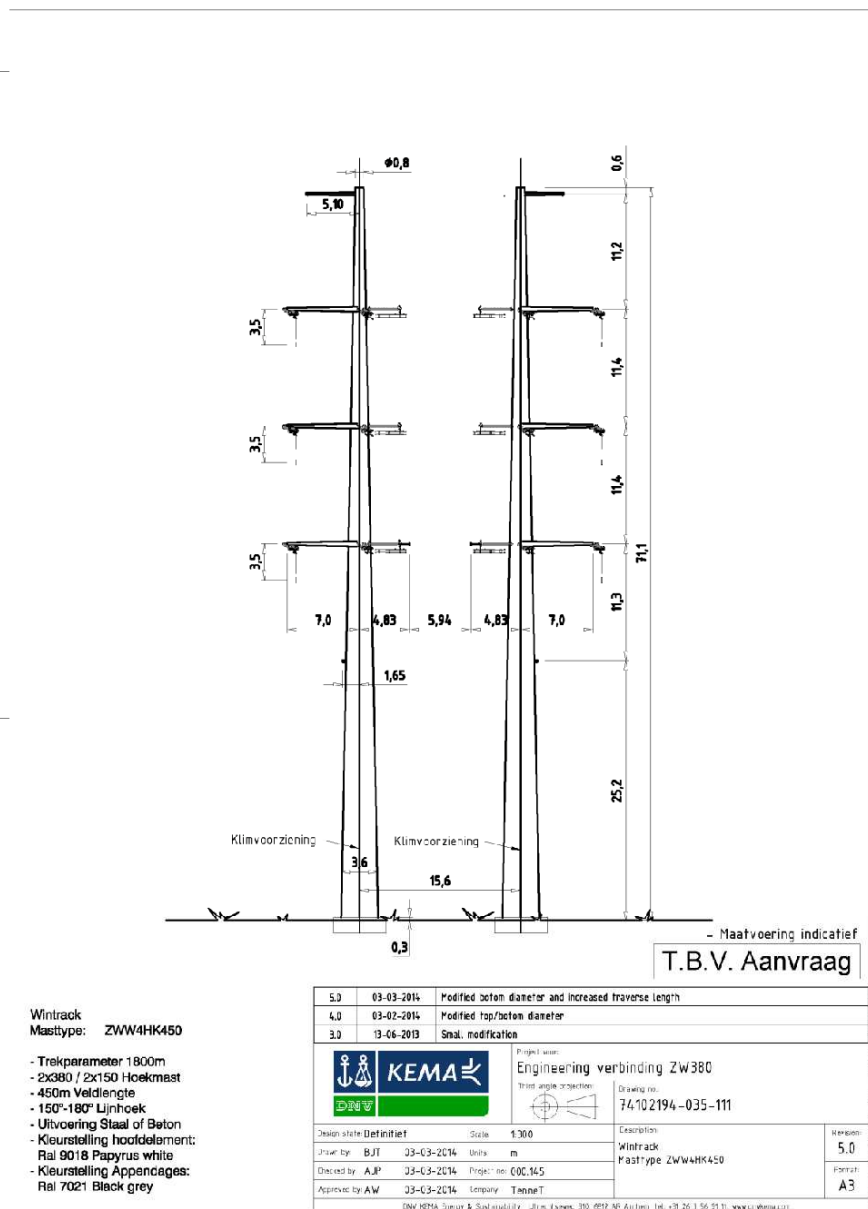
Afbeelding N17, mastbeeld ZWW4HK450
