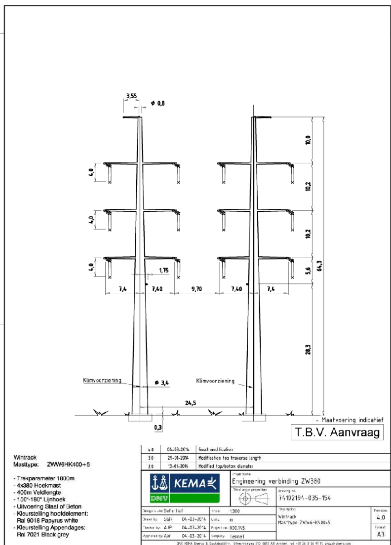
Afbeelding B23, mastbeeld ZWW6HK400+5
