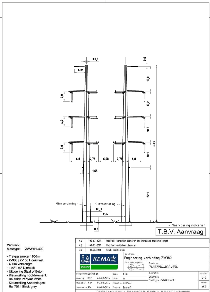
Afbeelding N12, mastbeeld ZWW4HL400
