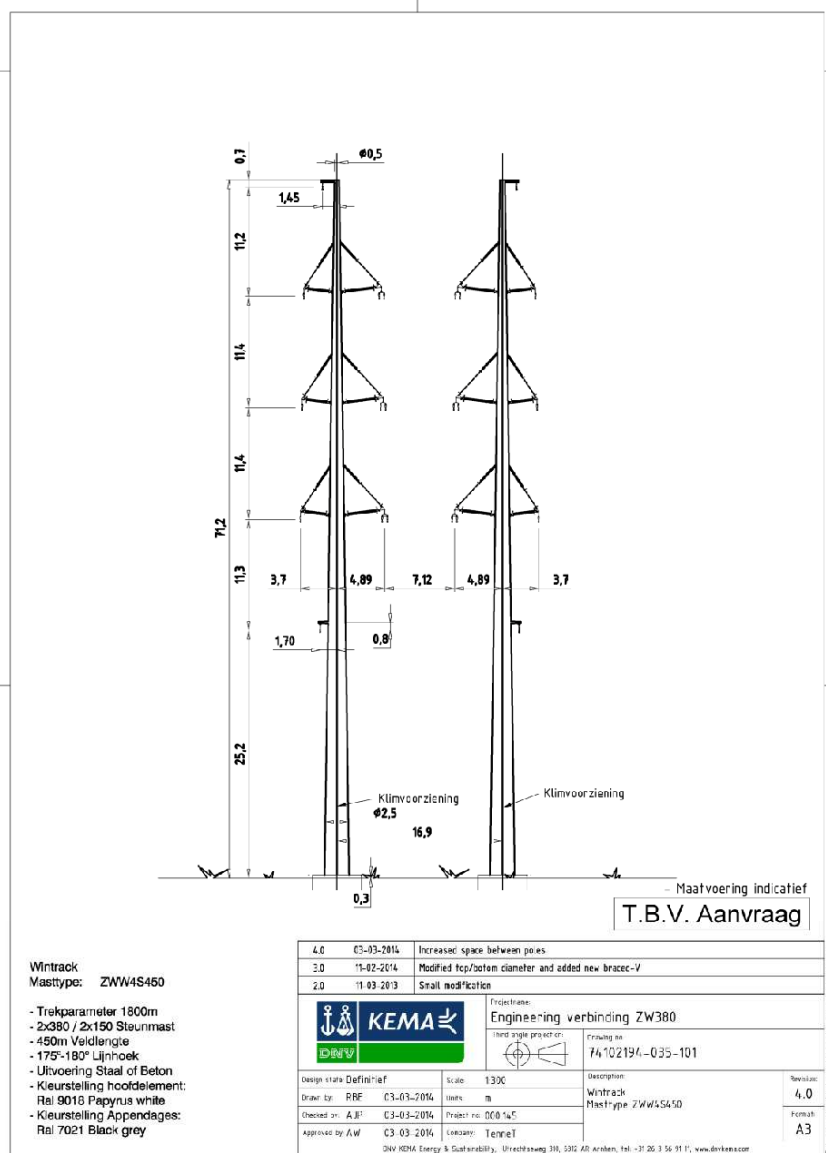
Afbeelding N16, mastbeeld ZWW4S450
