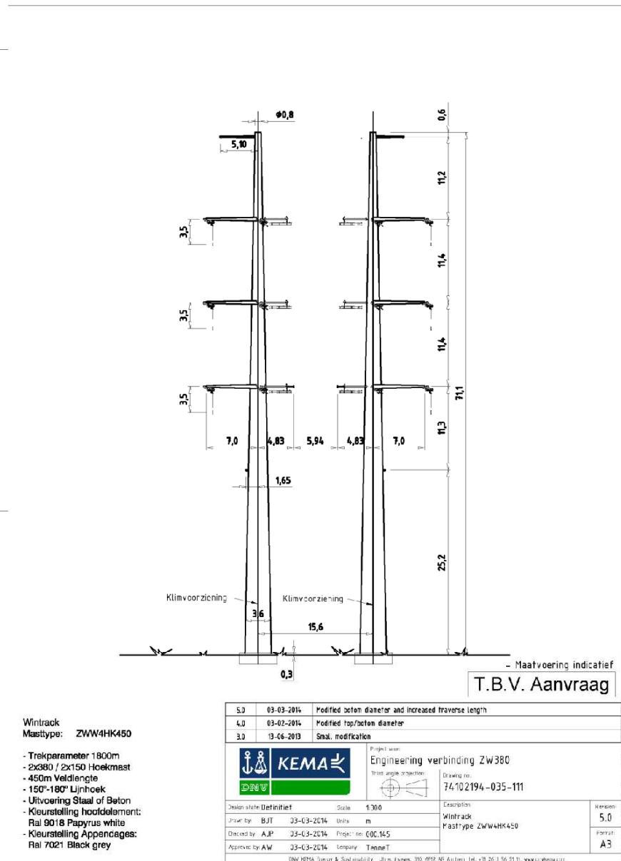
Afbeelding B17, mastbeeld ZWW4HK450
