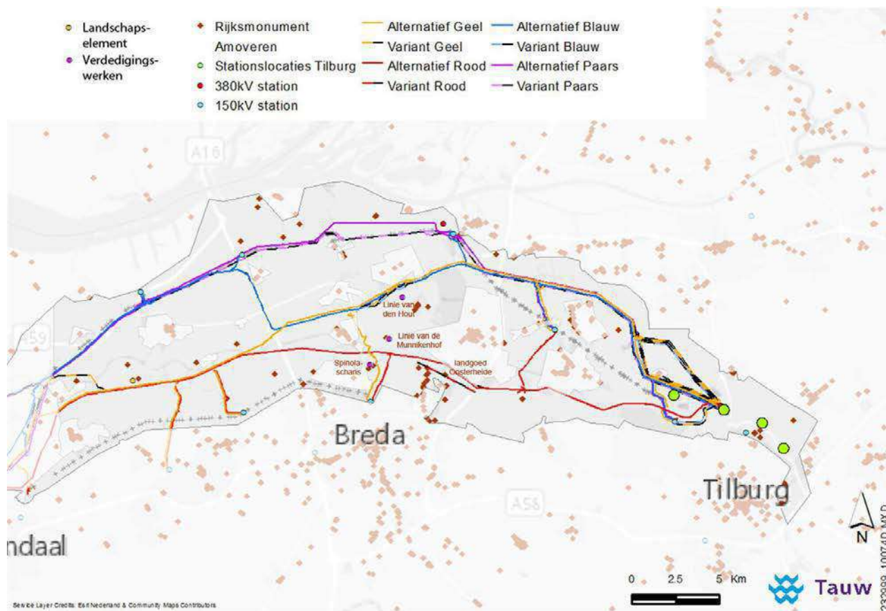
Figuur 3.30 Objecten en elementen op mastniveau, deelgebied 3
