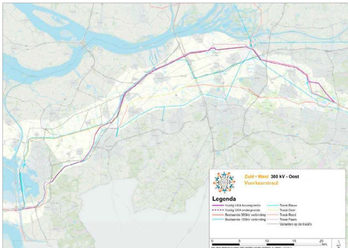
Figuur 2.1 Voorgenomen tracé uit 2017
