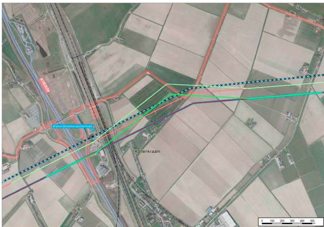
Figuur 9.3 Moerdijk - Zevenbergschen Hoek - Variant Groen
