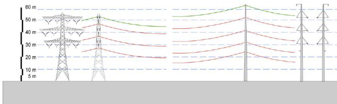
Figuur 2.2 Draadconfiguraties en masthoogte bij Moldaumasten (links) en wintrackmasten (rechts)
