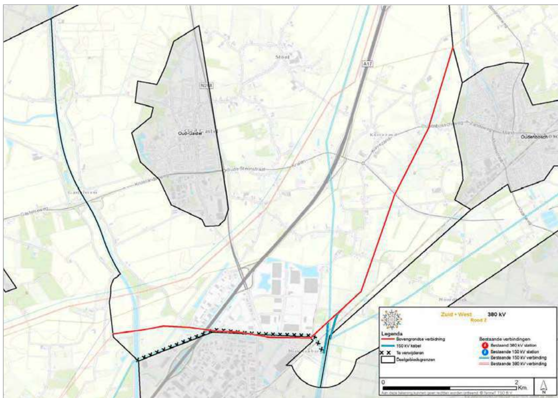
Figuur 6.2 Tracé van Rood 2
