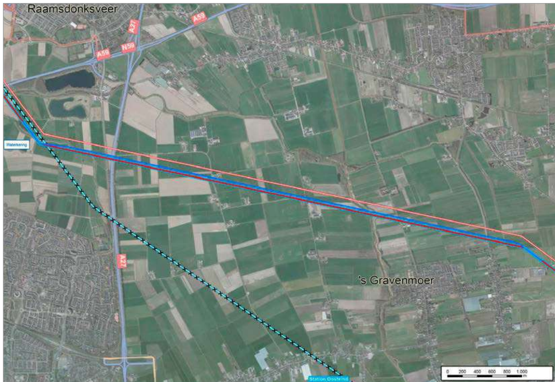
Figuur 12.3 's Gravenmoer - Variant Blauw
