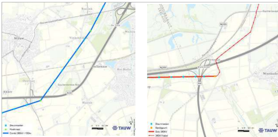
Figuur 5.1. De knik om zo noordelijk mogelijk bij Volckerdorp te passeren en de inpassing bij knooppunt Markiezaat met het opstijgpunt.
