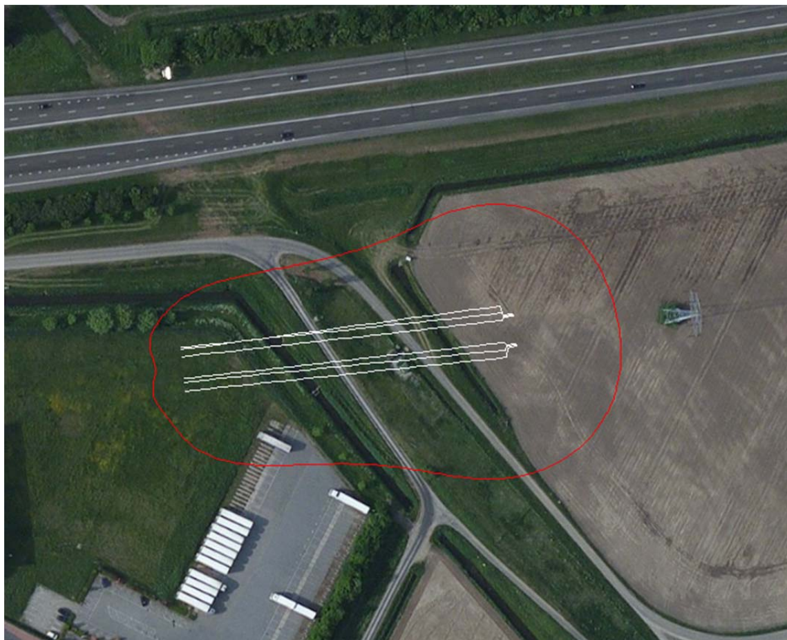
Figuur 2: Weergave "Cumulatieve magneetveld" 0,4 microteslacontour opstijgpunt 94a
