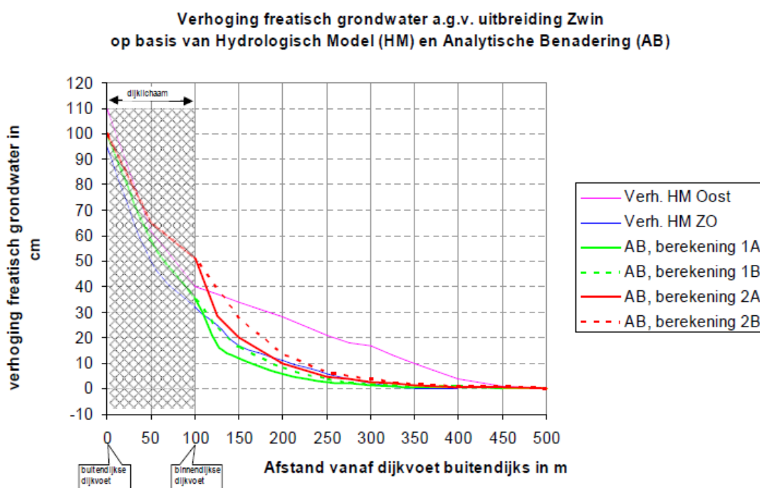
Figuur 12-2: Resultaten analytische berekeningen (AB) en hydrologisch model (HM)
