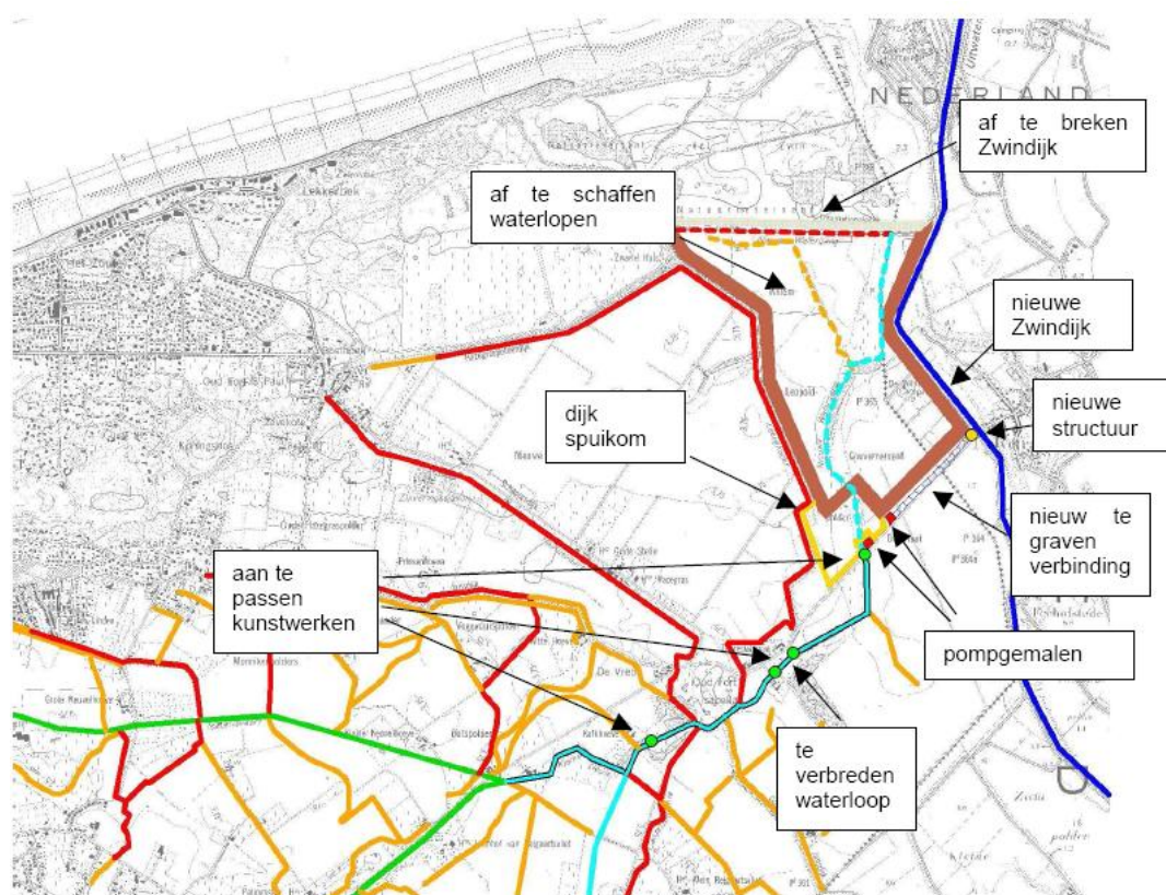
Figuur 5-17: Overzicht ingrepen alternatief 2
