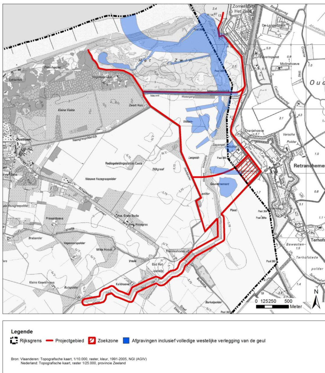
Figuur 5-5: Situering van de westwaarts verlegde Zwingeul
