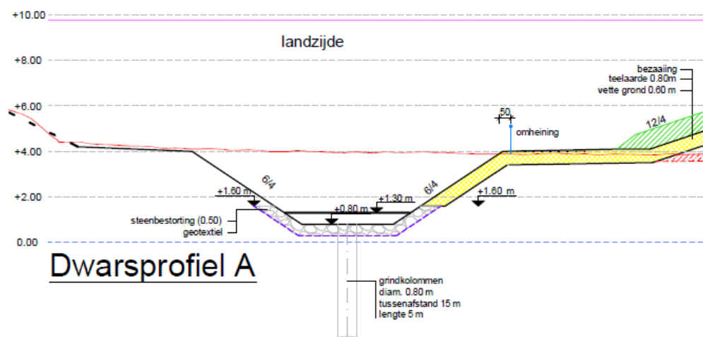
Figuur 12-1: Ontwerp dwarsprofiel zilte gracht
