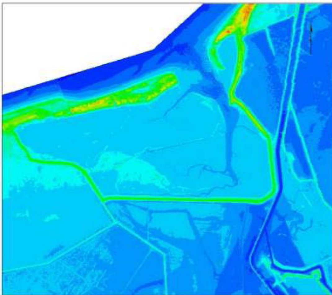
Figuur 4-6: Resulterende topografie na afgraven van de westelijke duin
