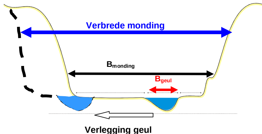
Figuur 4-5: Schematische dwarsdoorsnede van de toegangsgedul, met daarin aangegeven de breedte van de huidige monding tussen de duinmassieven ( B_{\text{mondin}} ), de breedte van de feitelijke toegangsgedul ( B_{\text{geul}} ), de verbrede monding en de geplande verlegging van de geul
