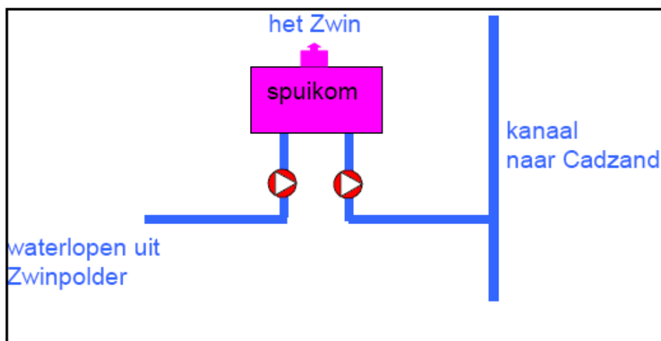
Figuur 5-15: Schematische weergave spuiwerking
