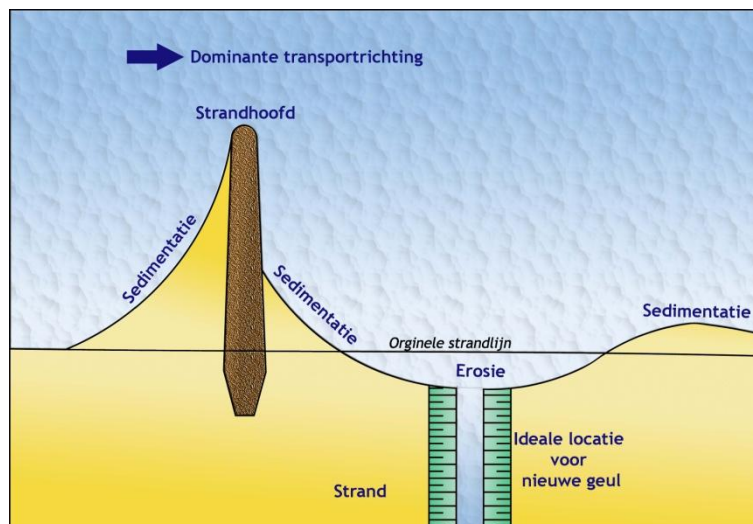
Figuur 5-1: Effect van een strandhoofd of strekdam op de kustlijn
