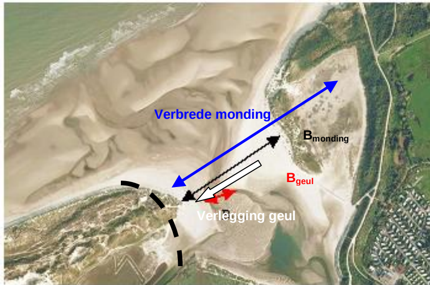
Figuur 4-4: Bovenaanzicht van de huidige toegangsgedul, met de breedte van de huidige monding tussen de duinmassieven ( B_{\text{mondin}} ), de breedte van de feitelijke toegangsgedul ( B_{\text{geul}} ), de verbrede monding en de verlegging van de geul
