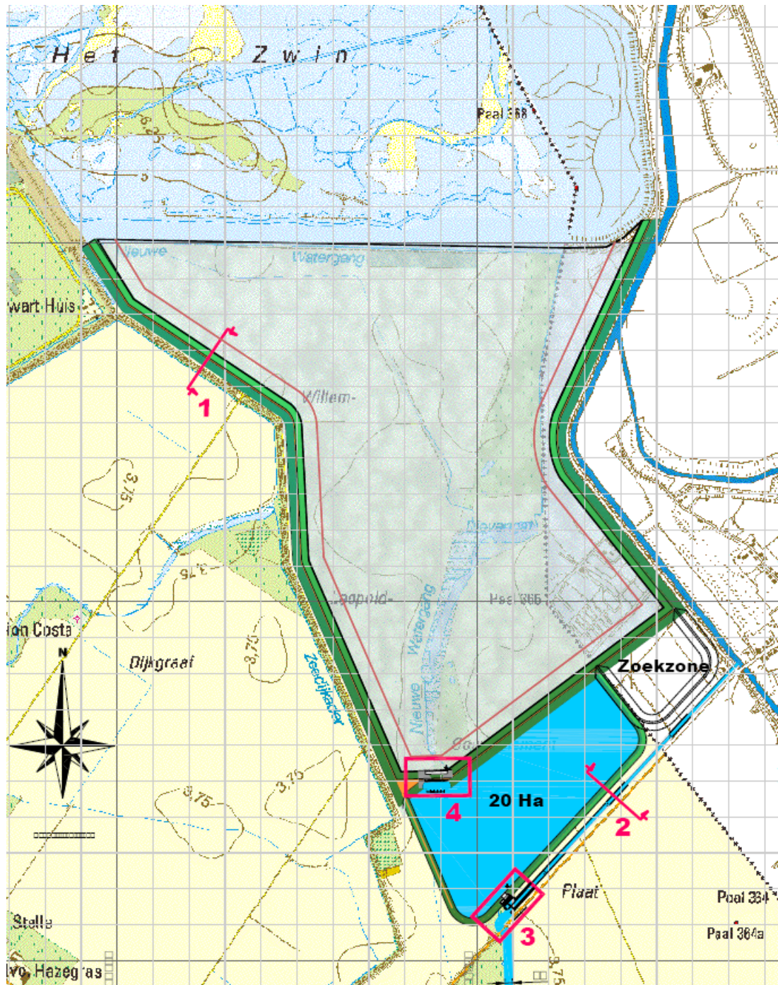
Figuur 5-13: Alternatief 2B met spuikom (voorontwerp)
