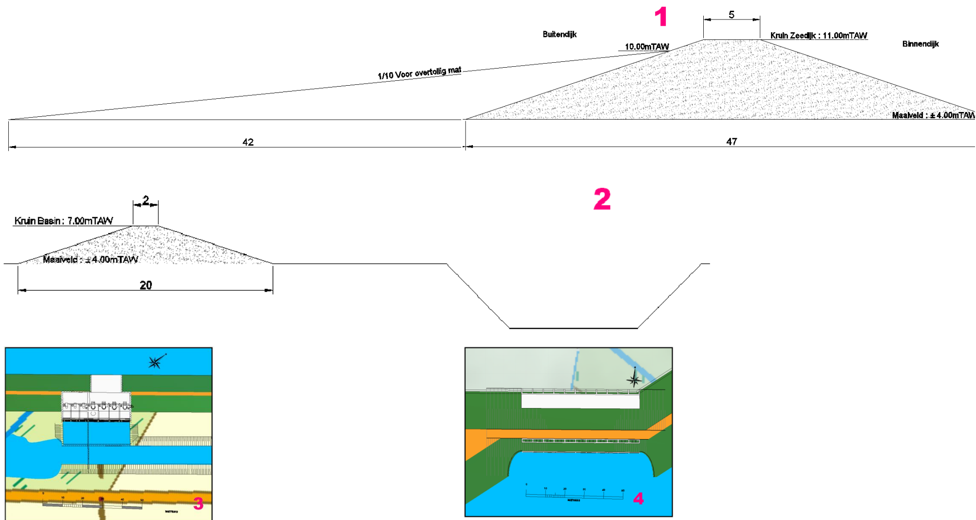
Figuur 5-14: Details alternatief 2B met spuikom (voorontwerp)
