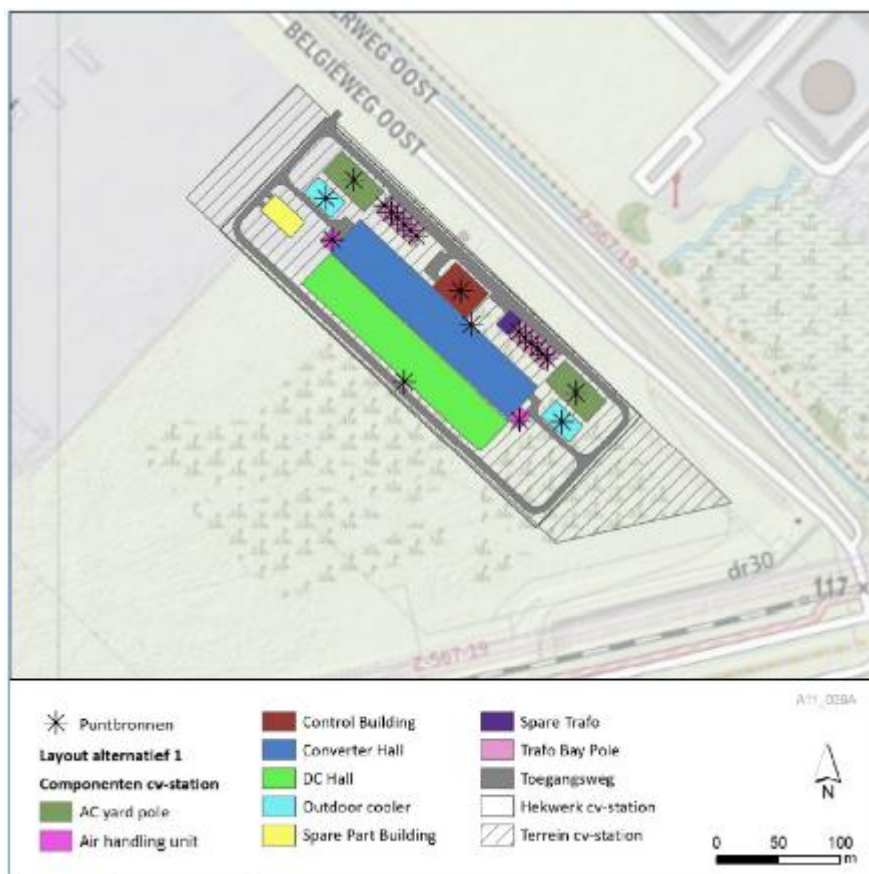
Figuur 5.16. Geluidbronnen converterstation Borssele
