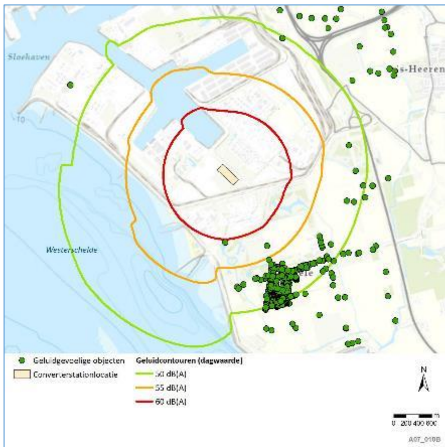
Figuur 5.31. Geluidcontouren heiwerkzaamheden tijdens aanlegfase converterstation Borssele in relatie tot geluidgevoelige objecten
