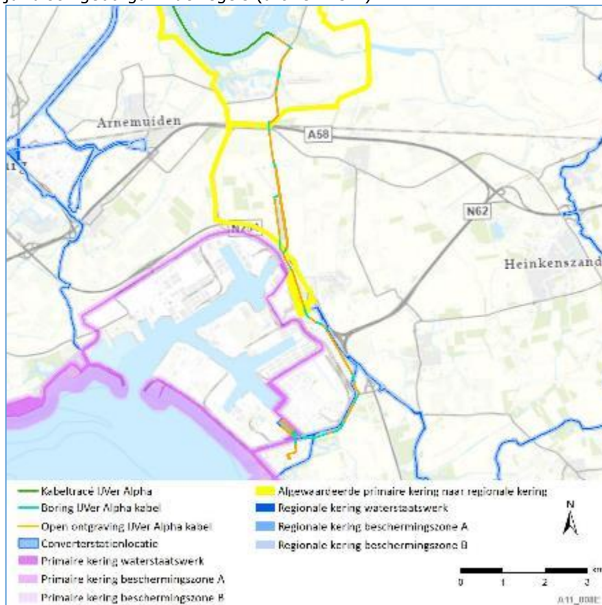
Figuur 5.24. Primaire waterkeringen Borssele op land (Waterschap Scheldestromen, 2012) (hier nog weergegeven met varianten Sloekreek)
