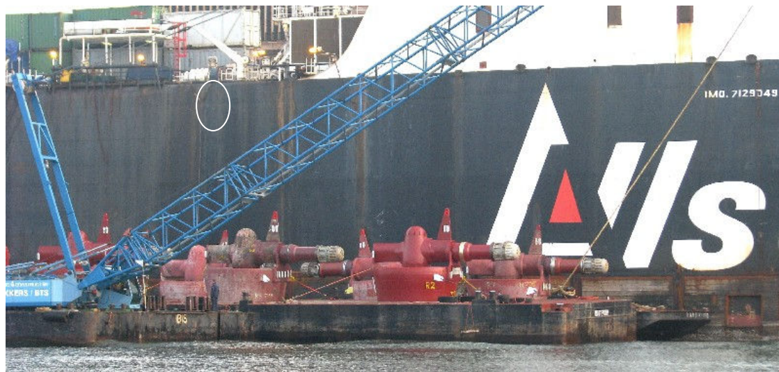
Figuur 3 Enkele thrusters van de pijpenlegger 'Solitaire' (let op de man onder de kraan om een idee te krijgen van de grootte).
