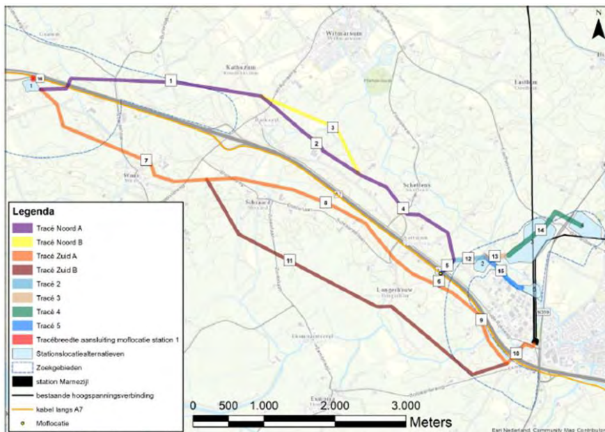
Afbeelding 2.6 Kabeltracéalternatieven
