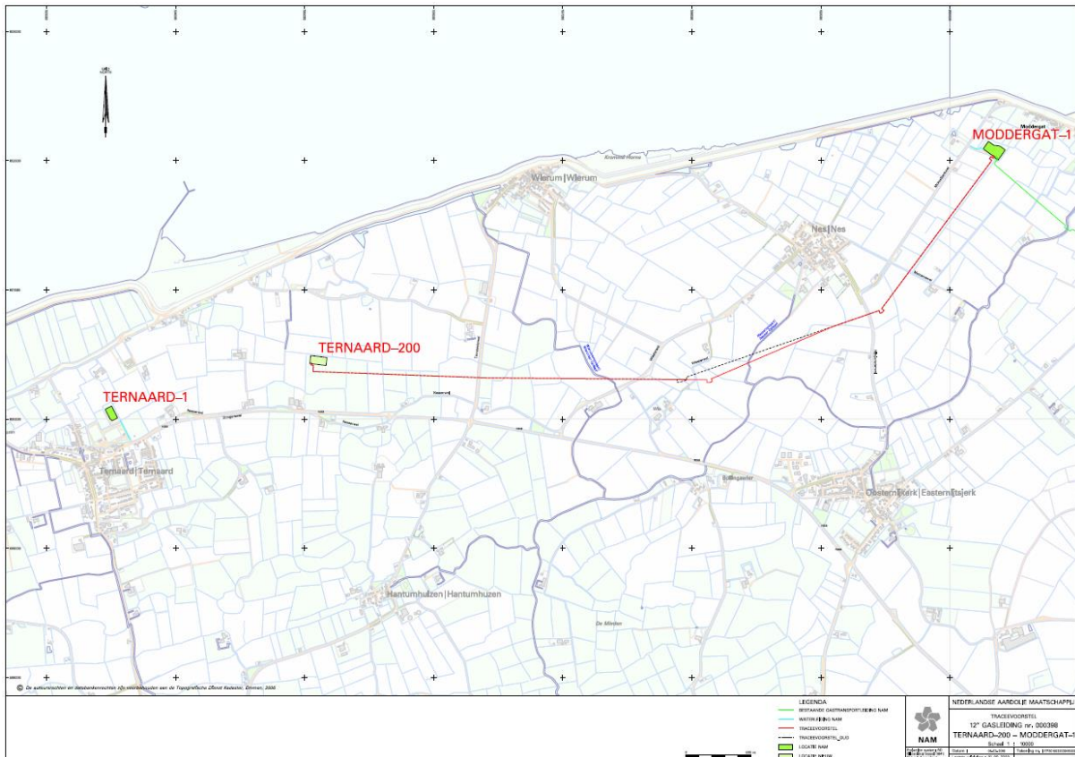
Figuur 3 Aan te leggen tracé Ternaard-Moddergat
