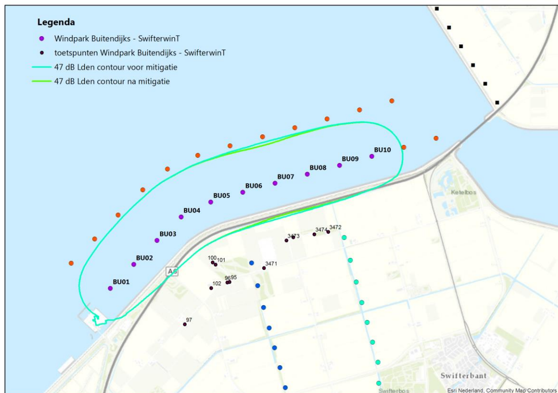
Afbeelding 3.1 47 dB L_{den} geluidscontour van windpark Buitendijks - SwifterwinT
