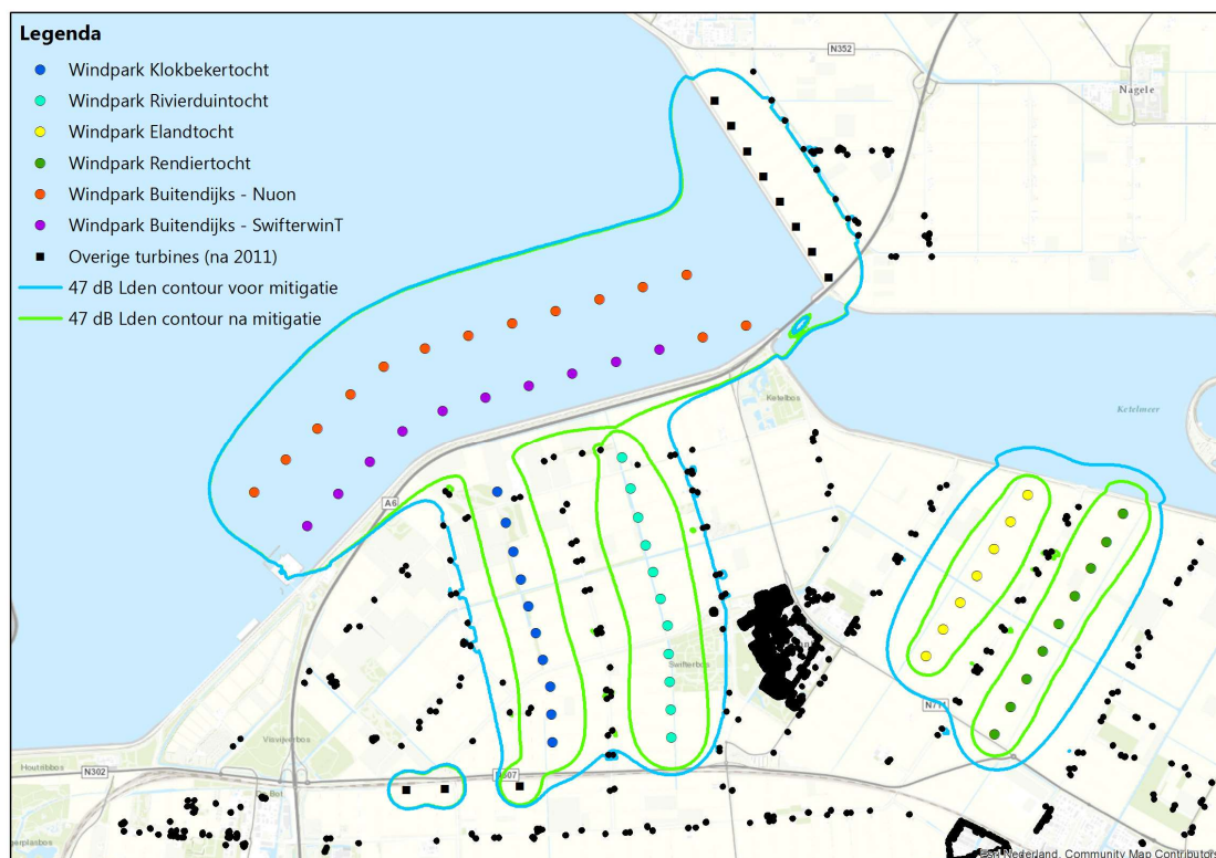
Afbeelding 5.2 47 dB L_{den} geluidscontour voor en na mitigatie
