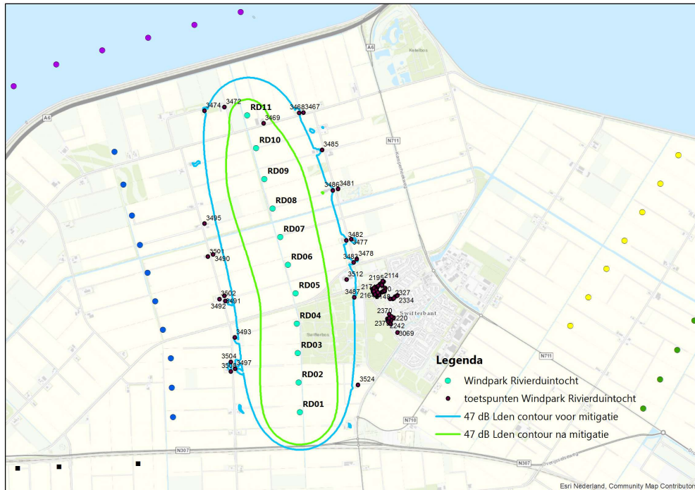
Afbeelding 3.1 47 dB L den geluidscontour van windpark Rivierduintoicht voor en na mitigatie
