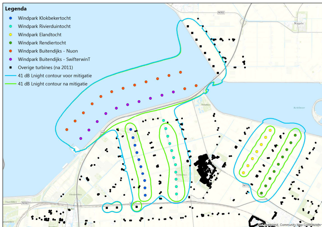
Afbeelding 5.3 41 dB L_{night} geluidscontour voor en na mitigatie
