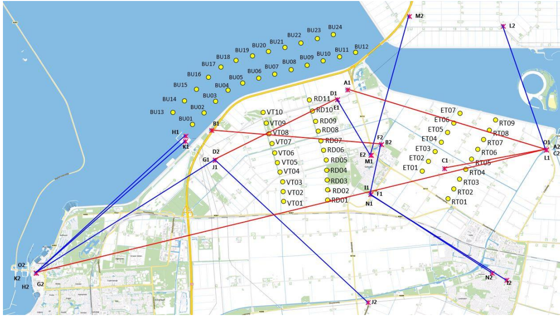
Afbeelding 4.1 Locatie van turbines en straalpaden voor VKA 10.0
