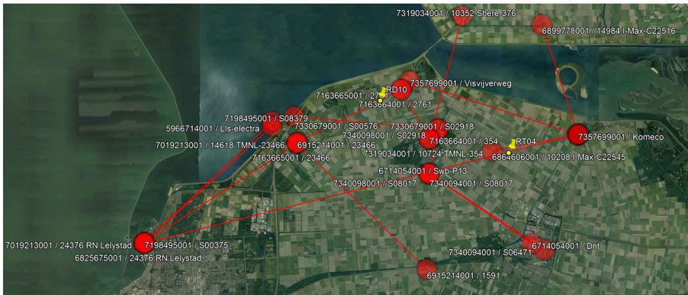
Afbeelding 4.5 Locatie van de twee kritische turbines (RD10) en RT04
