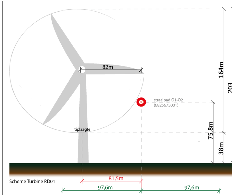
Afbeelding 4.4 Zicht van turbine nummer RD01 van de VKA
