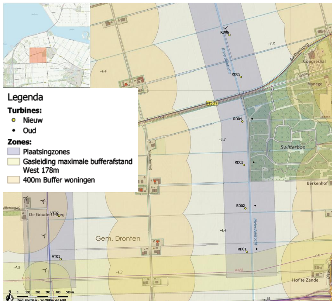
Afbeelding 1.1 Vier zuidelijke turbines van de Rivierduintocht
