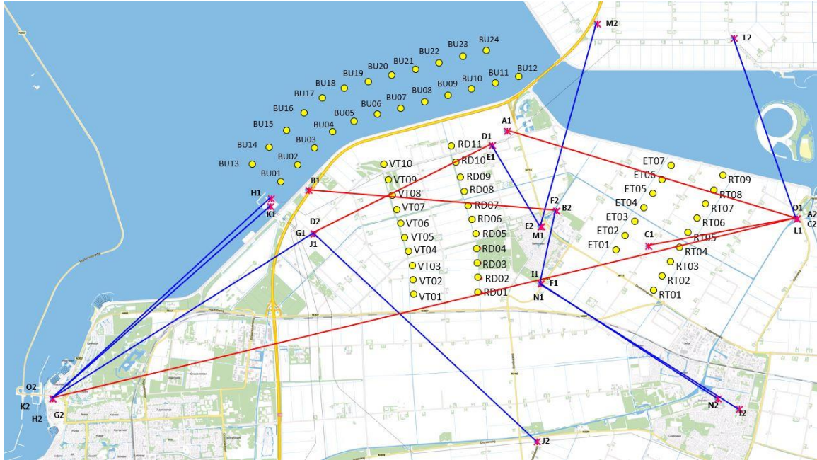
Afbeelding 2.2 Illustratie van straalpaden en VKA 10.0 in het gebied van WP Blauw
