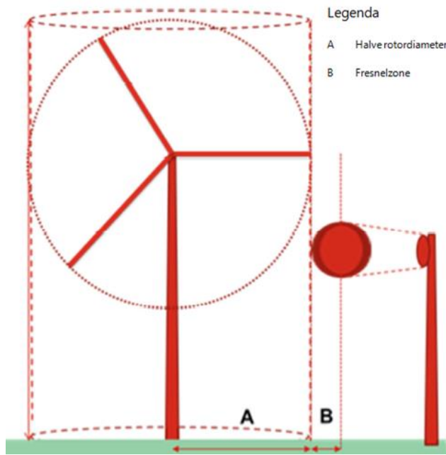
Afbeelding 3.1 Aanbevolen veiligheidsafstand tussen straalpaden
