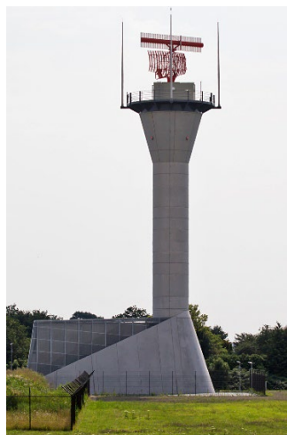
Figuur 3: De luchtverkeersleidingsradar bij Schiphol. De gecombineerde antenne draait rond met 15 omwentelingen per minuut (Bron: Luchtverkeersleiding Nederland (LVNL)).
