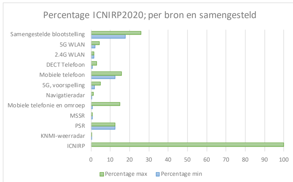
Figuur 4.7 Samengestelde blootstelling met de SMART-L in roterende modus inclusief de eigen RF-systemen op 370 m. De balken geven de minimale (blauw) en maximale (groen) te verwachten elektrische veldsterkte weer. Beide waarden worden vergeleken met de ICNIRP2020-richtlijn. Lager dan 100% betekent dat aan de richtlijn voldaan wordt.
