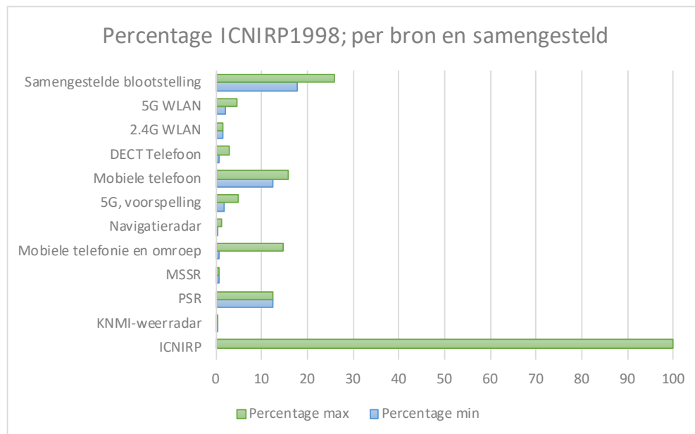
Figuur 4.5 Samengestelde blootstelling met de SMART-L in roterende modus inclusief de eigen RF-systemen op 370 m. De balken geven de minimale (blauw) en maximale (groen) te verwachten elektrische veldsterkte weer. Beide waarden worden vergeleken met de ICNIRP1998 richtlijn. Lager dan 100% betekent dat aan de richtlijn voldaan wordt.
