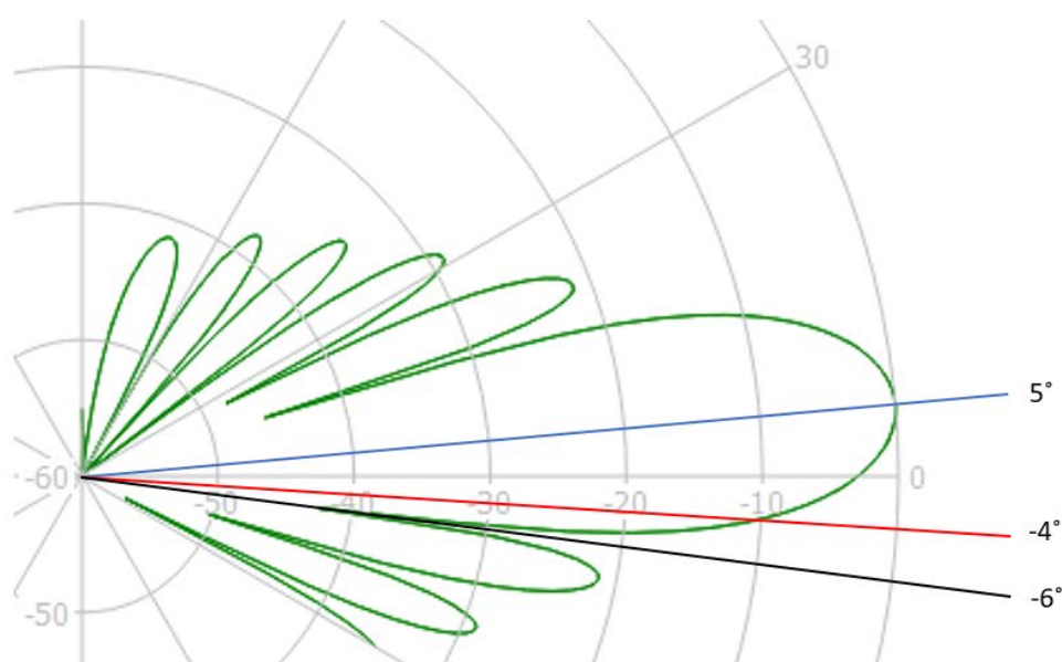
Figuur 2.2 Afbeelding van een elevatie antennepatroon (groene lijn) bij zenden. De cirkels geven het niveau van de antenne-uitstraling aan. Dit is in decibels (dB) gegeven en 0 dB is het maximum en de waarde van de antenne-uitstraling in een bepaalde richting is de antennewinst.
