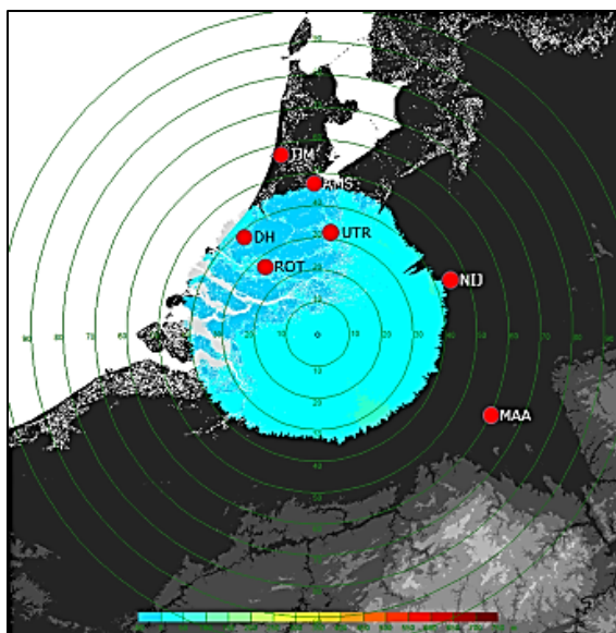
Fig. 5. Bereik radar bij plaatsing op vliegbasis Gilze Rijen
