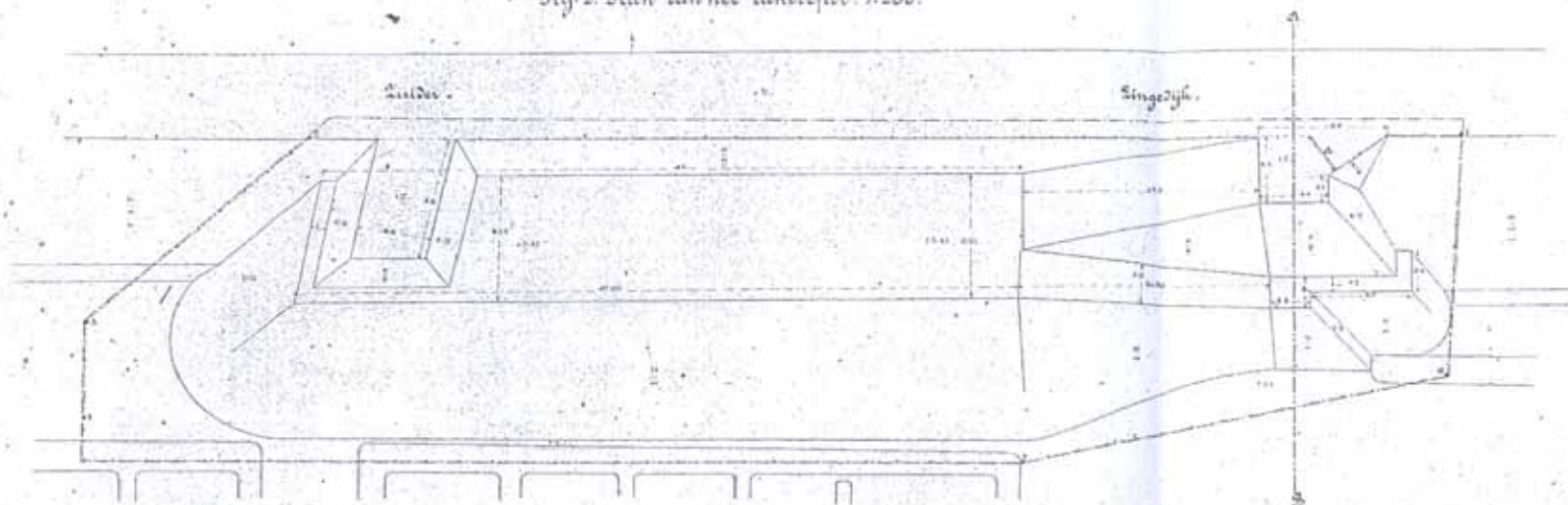
Fig 2. Plan van het landepoort. 1:200.
