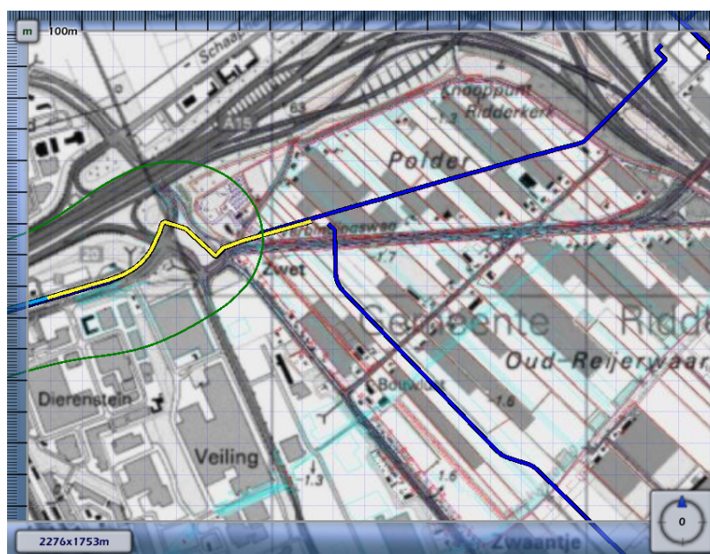
Figuur 2.7 Plaatsgebonden risico doorgaande hogedrukaardgastransportleiding A-559 groene contour : 10^{-8} per jaar
