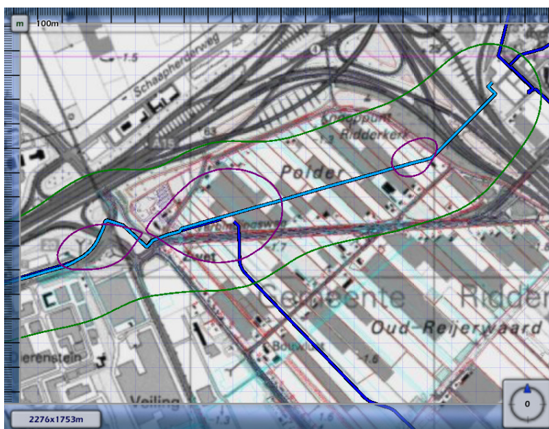
Figuur 2.5 Plaatsgebonden risico doorgaande hogedrukaardgastransportleiding A-517 gele contour : 10^{-7} per jaar groene contour : 10^{-8} per jaar
