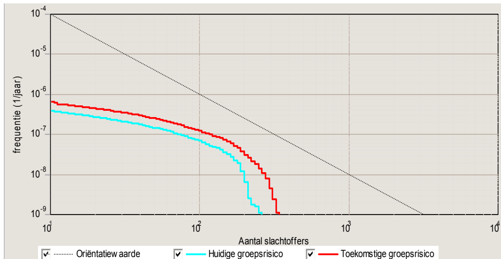
Figuur 2.8 Groeprisico van rijkswegen A15 en A15/16 ter hoogte van Reijerwaard
