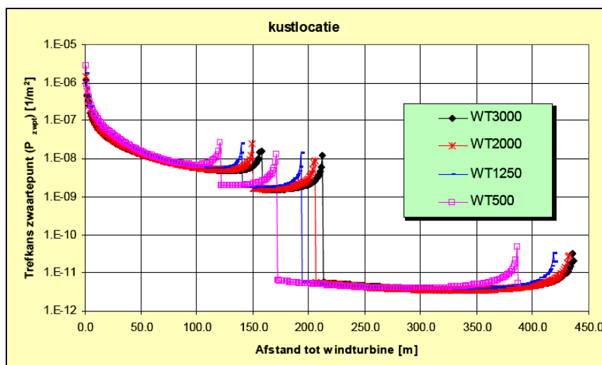
Figuur 5.1 Trefkans per jaar van het zwaartepunt van het blad als functie van de afstand tot de turbine voor een kustlocatie.
