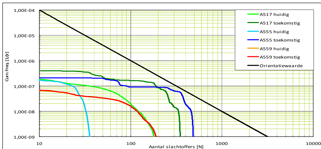
Figuur 3.3 Groepsrisico hogedrukaardgastransportleidingen
