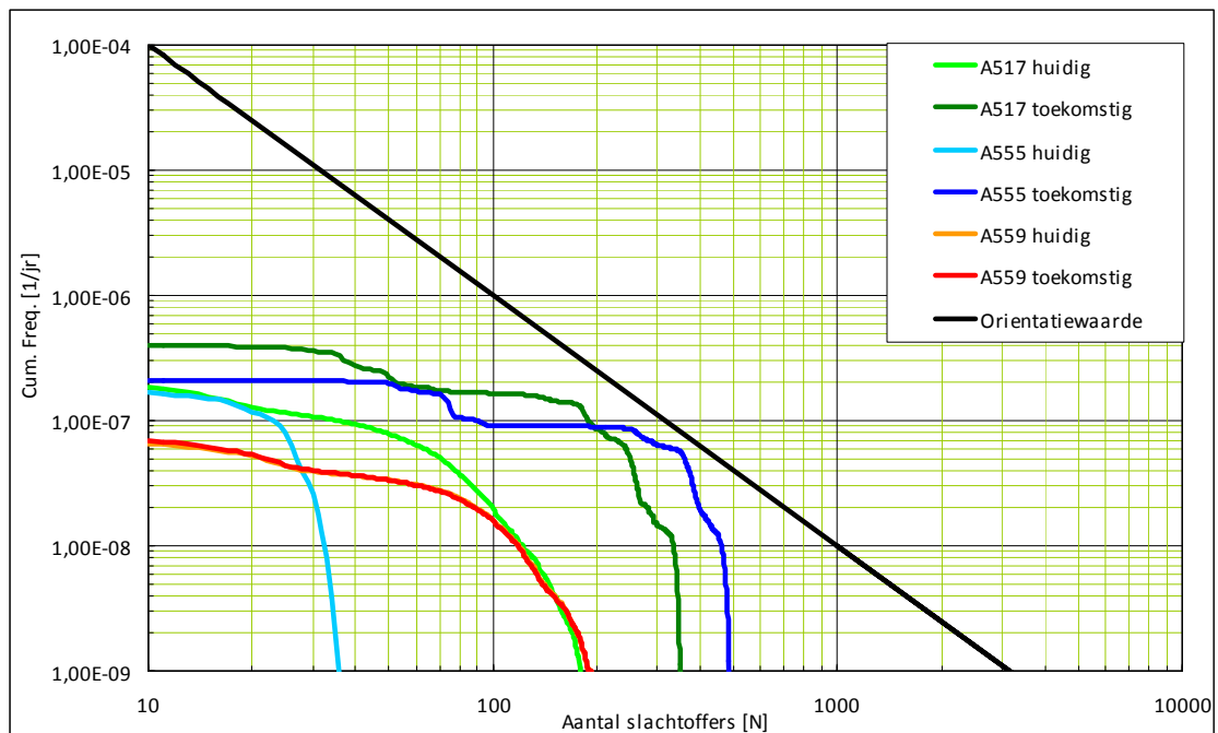
Figuur 2.1 fN-curves van hogedruk-aardgastransportleidingen
