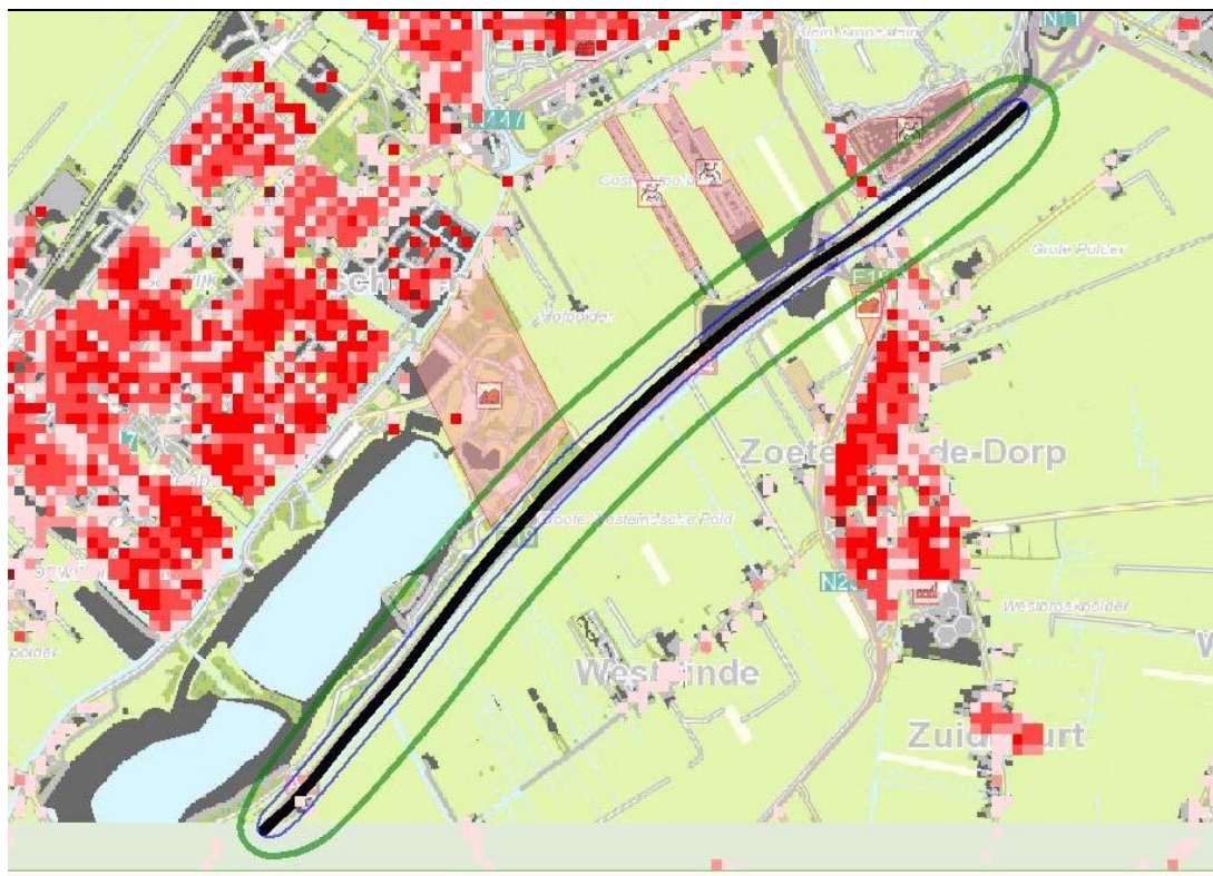
Figuur 4.10 PR-contouren Toekomstige situatie A4 (Blauw = 1 \times 10^{-7} /jaar, groen = 1 \times 10^{-8} /jaar)
