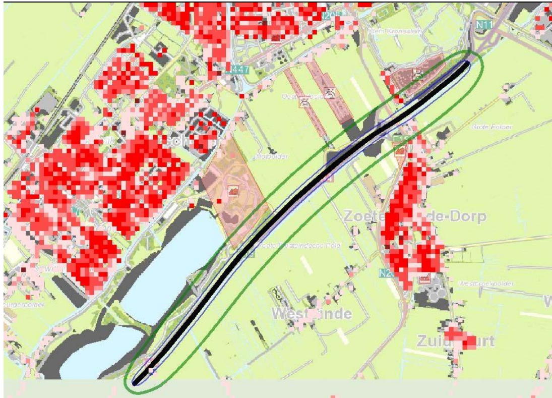
Figuur B3.2 Plaatsgebonden risicocontour. Autonome situatie A4 (Blauw = 1 \times 10^{-7} /jaar, groen = 1 \times 10^{-8} /jaar)
