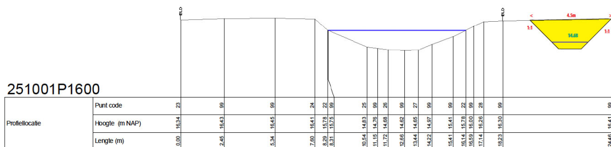
Figuur 4.2.2c. Nieuwe doorsnede van de Peelse Loop benedenstrooms in traject II. De nieuwe bedding (geel) ligt rechts van de oude bedding, die als langgerekte vijver blijft bestaan. NB, de schaal van beide profielen verschilt, de bedding is in beide gevallen vergelijkbaar.
