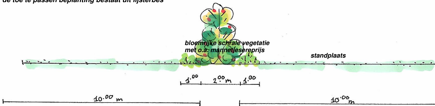
dwarsdoorsnede C – C': strook met struikvegetatie/schraal grasland de toe te passen beplanting bestaat uit lijsterbes
