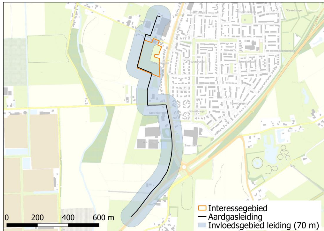
Figuur 1. Interessegebied en invloedsgebied rond aardgasleiding Z-525-01
