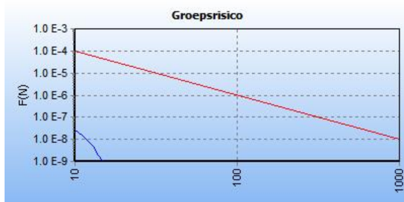
Figuur 3. Groepsrisico Z-525-01 in de huidige en toekomstige situatie
