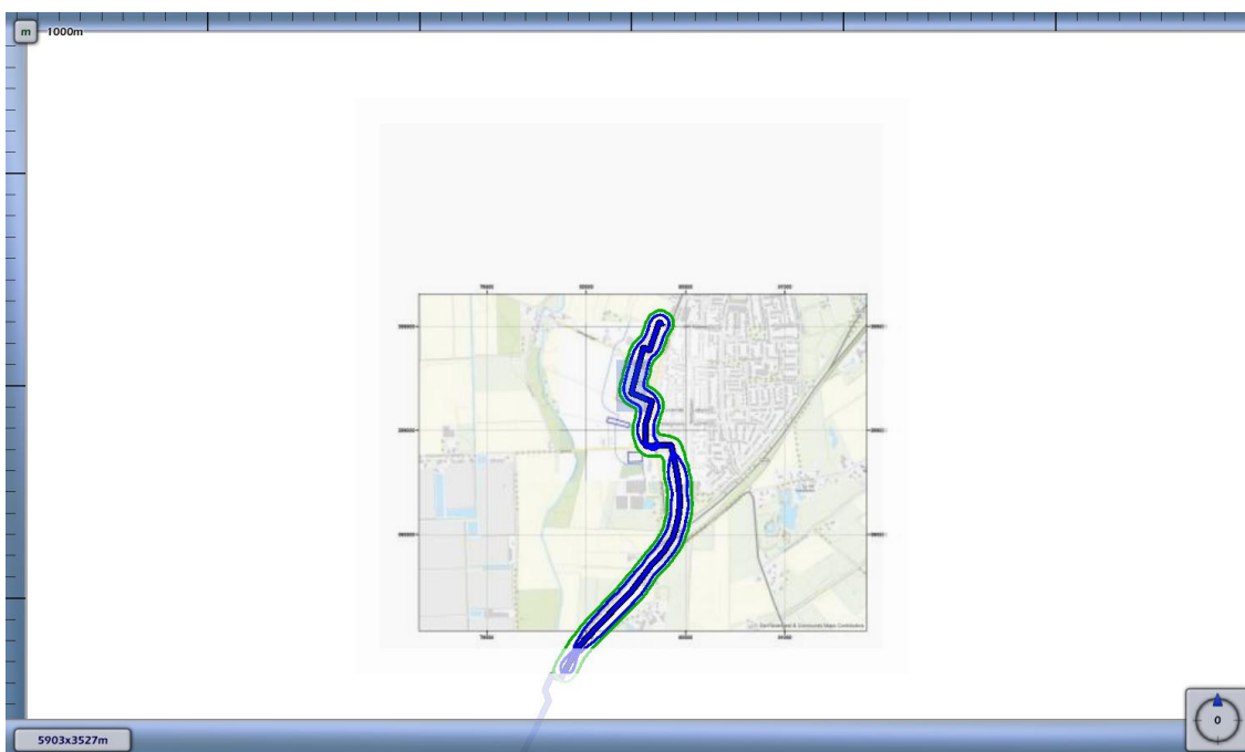
3.1 Figuur 3.1 Plaatsgebonden risico voor 4252_leiding-Z-525-01-deel-1 van N.V. Nederlandse Gasunie
