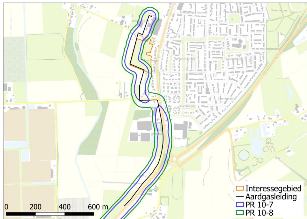
Figuur 2. PR-contouren aardgasleiding Z-525-01
