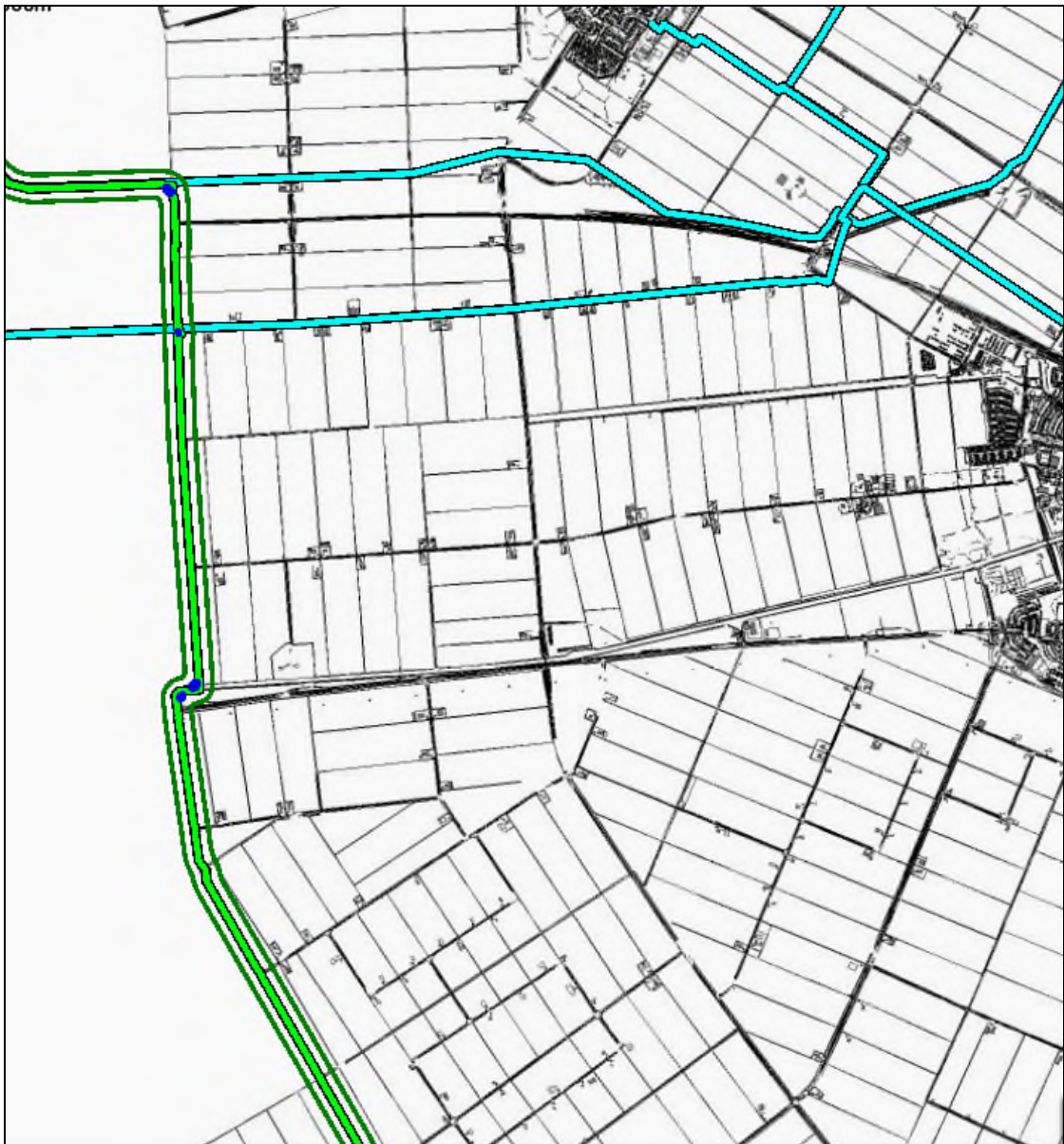
Figuur 4.1a Plaatsgebonden risico hogedruk-aardgastransportleiding
