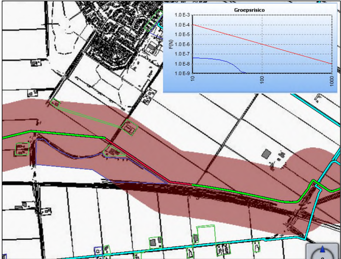
Figuur 4.13d Resultaat groepsrisicoberekening: groepsrisicocurve en ligging km met maximaal groepsrisico (rode lijn)
