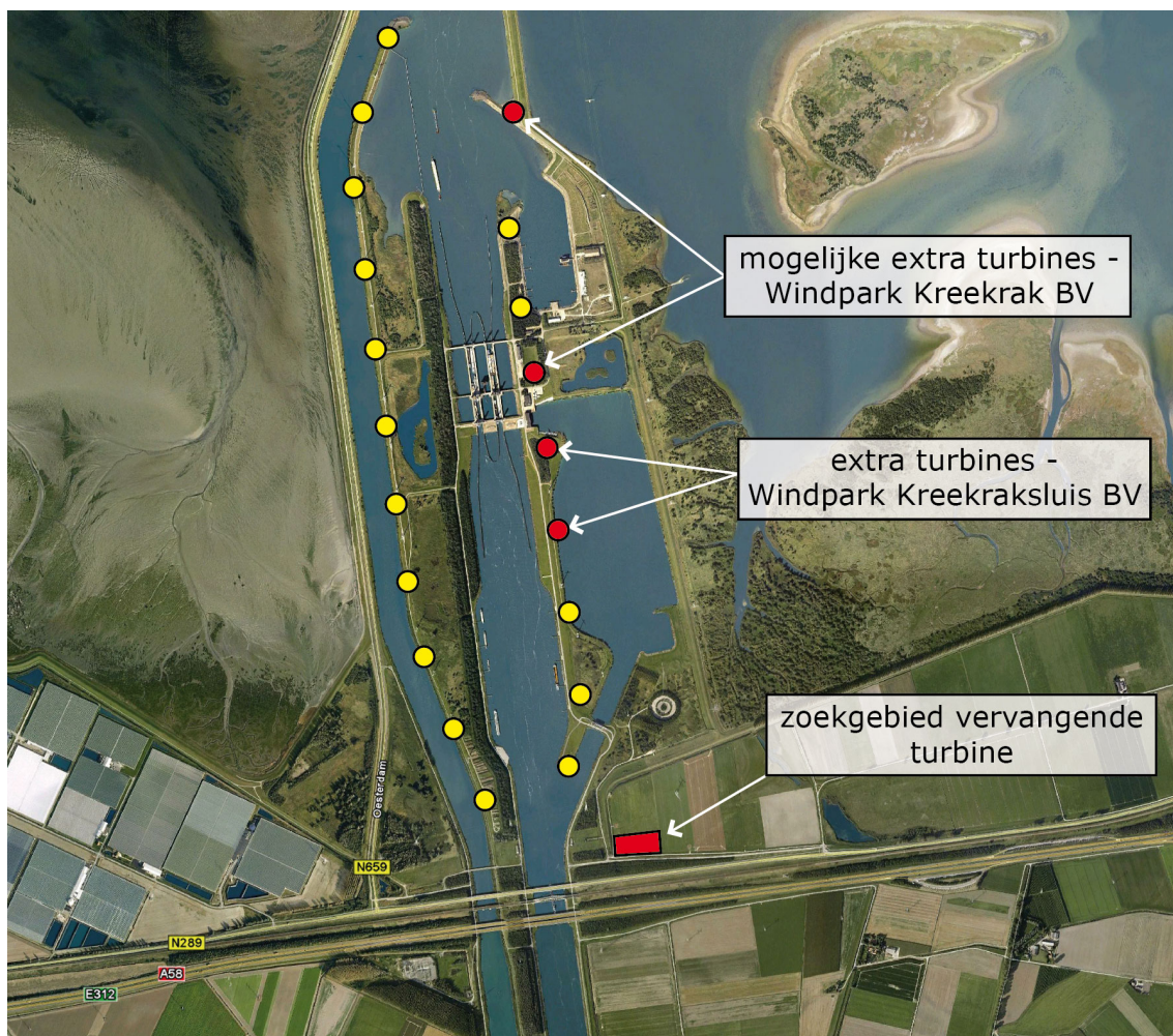
Figuur 1.2. Beoogde opstelling Windturbinepark Kreekraksluizen inclusief de drie afzonderlijke deelprojecten voor optimalisatie (bron: Google Maps)
